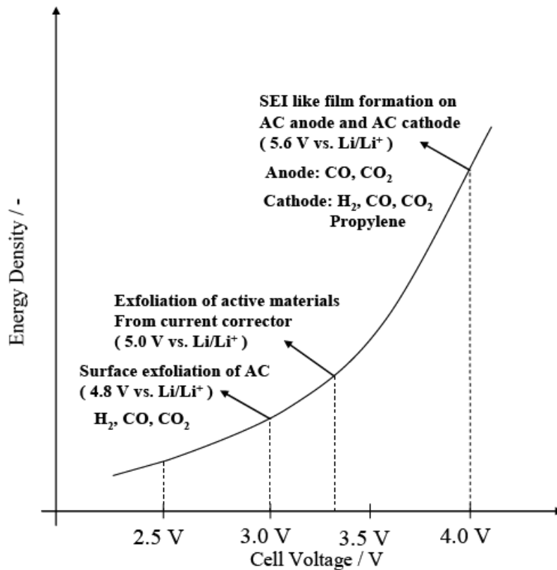
Figure I-12 : processus de vieillissement d'un supercondensateur à base de PC selon
