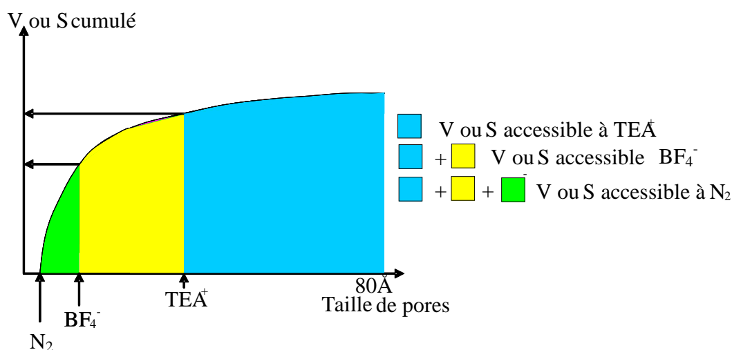
Figure III-35 : représentation du volume et de la surface accessible pour une espèce donnée
