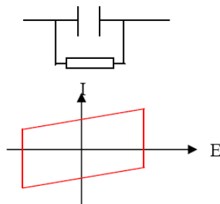
Figure I-6 : voltampérogramme d'un condensateur et d'une résistance montés en parallèle
