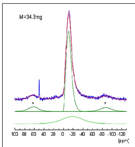
Figure III-39 : RMN ^{27}\text{Al} MAS sur le séparateur cellulosique
