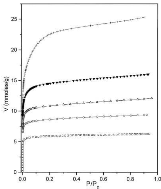
Figure VI-1 : isothermes d'adsorption d'azote de carbones activés avec différents degré d'activation : □, D8; ○, D19; △, D34; ▼, D52; +, D80, chaque chiffre correspond au % de degré d'activation du carbone activé
