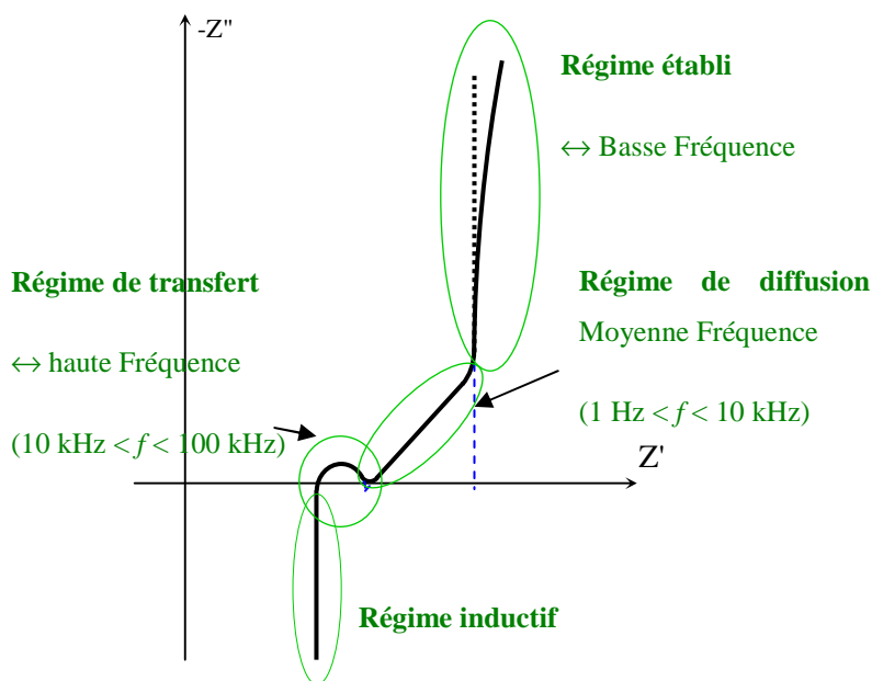
Figure II-19 : Diagrammes de Nyquist du schéma générique équivalent d'une structure "supercondensateur"
