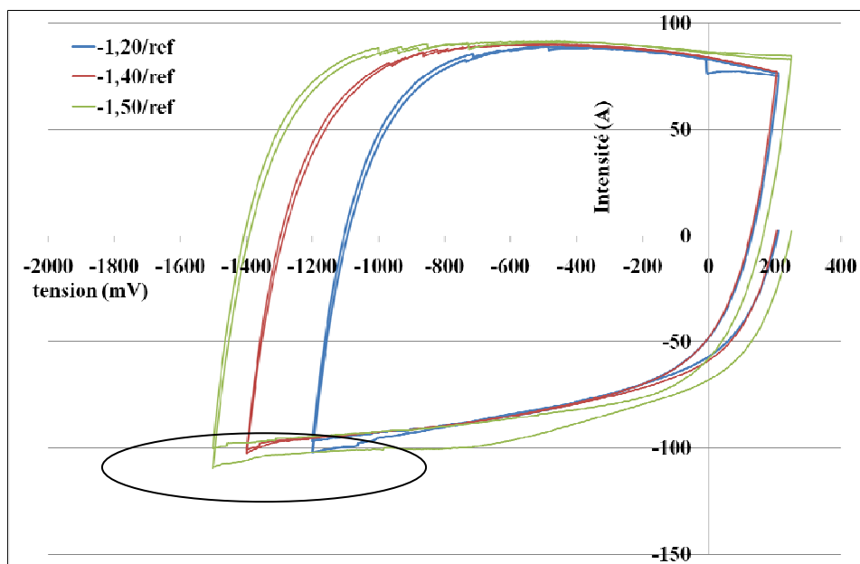
Figure IV-25 : Voltampérogrammes cathodique dans un système électrolyte purifié + \text{Na}_2\text{CO}_3 en fonction du potentiel imposé entre l'électrode et l'électrode de référence obtenus avec un film Batscap de 6\text{cm}^2 comme électrode de travail et de contre électrode, un fil d'argent enrobé par AgCl comme électrode de référence, l'ensemble à une température de 25^\circ\text{C} avec V_{\text{balayage}} = 20\text{mV/s}
