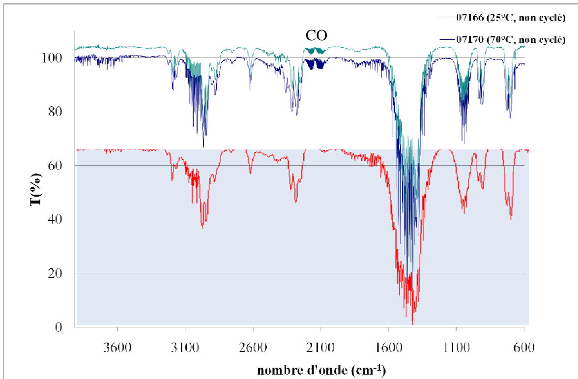
Figure II-9 : Spectres IR des gaz issus des supercondensateurs 07166 et 07170 maintenus respectivement à 25°C et 70°C sans mise sous tension superposé au spectre IR de l'acétonitrile tiré de la base NIST Chemistry Webbook (rouge)
