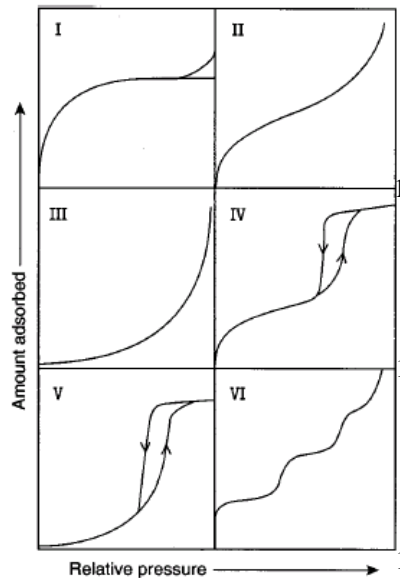
Figure I-8 : Classement IUPAC des diverses isothermes d'adsorption obtenues pour des pressions relatives P/P_0 variant de 0 à 1.
