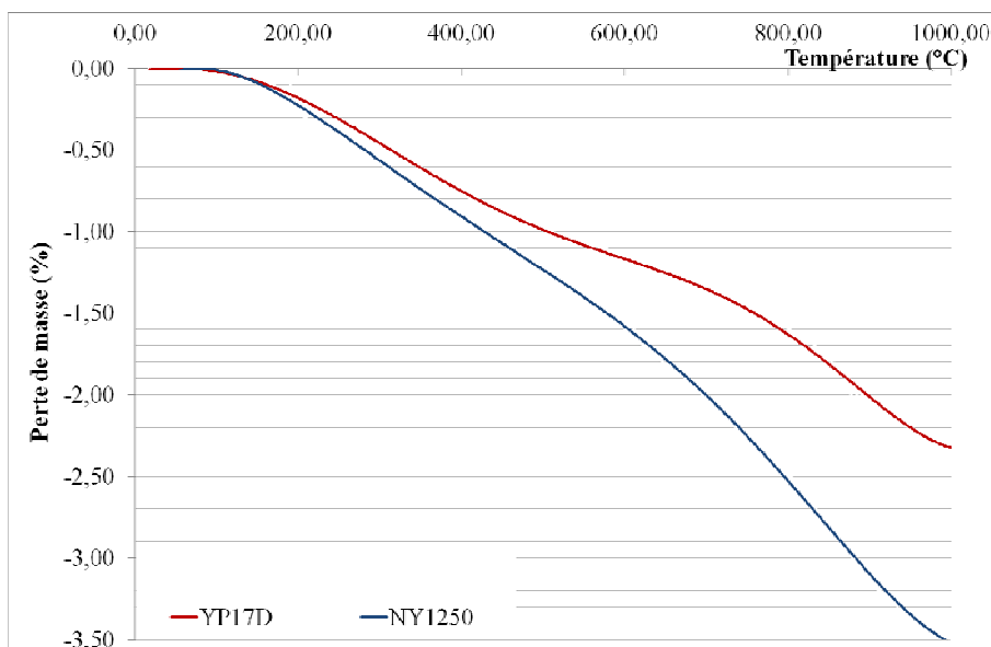
Figure III-4 : thermogramme des carbones activés F et B obtenu avec une vitesse de chauffe de 3°C/min sous balayage d'hélium
