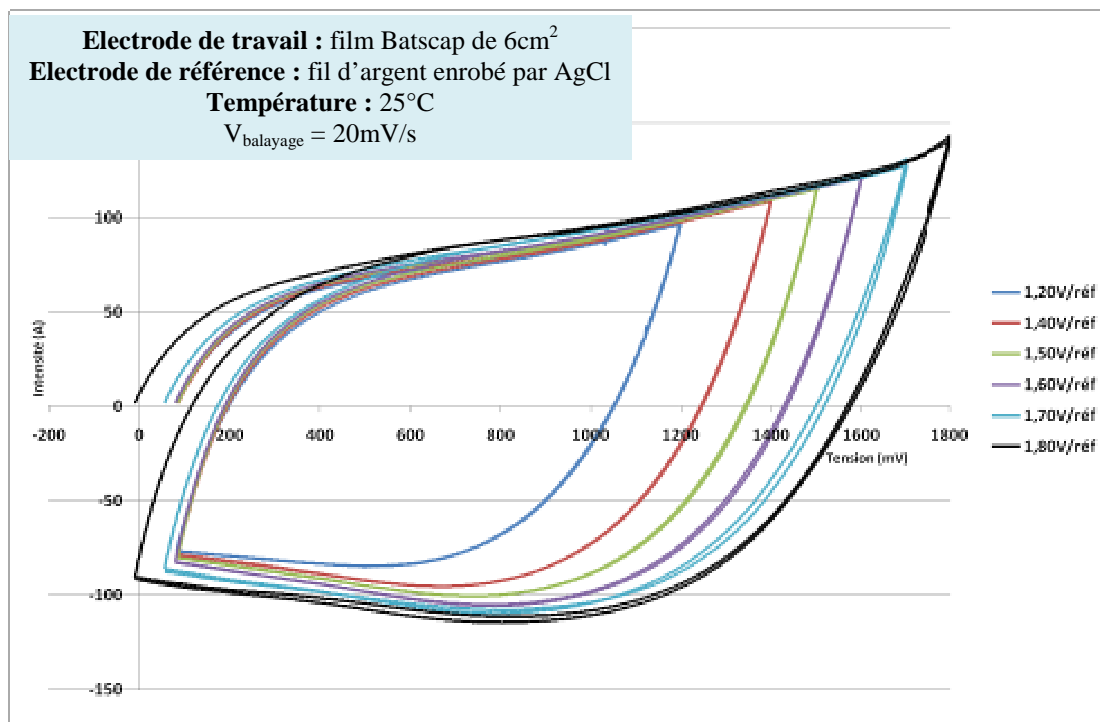
Figure VI-4 : Voltampérogrammes anodique dans un système sans séparateur en fonction du potentiel imposé entre l'électrode et l'électrode de référence (Ag/AgCl). (V = 20mV/s)
