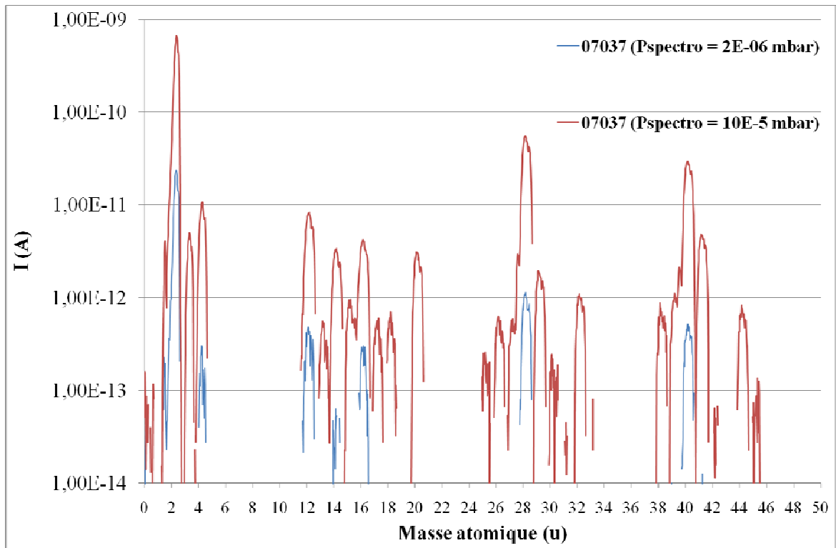
Figure II-2 : Spectres de masse obtenus sur un élément avec différentes pressions d'entrée du SM
