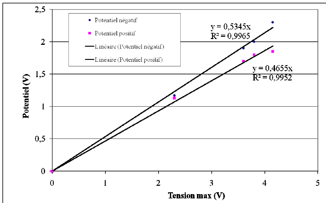
Figure IV-23 : potentiel accessible à chaque électrode en fonction des tensions maximales obtenues pour chaque type de séparateur
