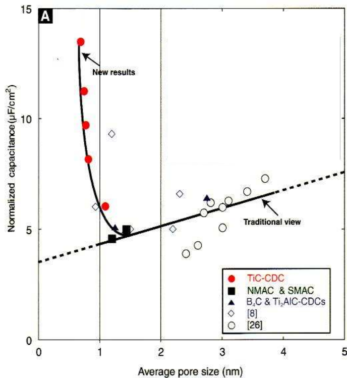
Figure I-13 : Variation de la capacitance de divers supercondensateurs en fonction de la taille des pores 74
