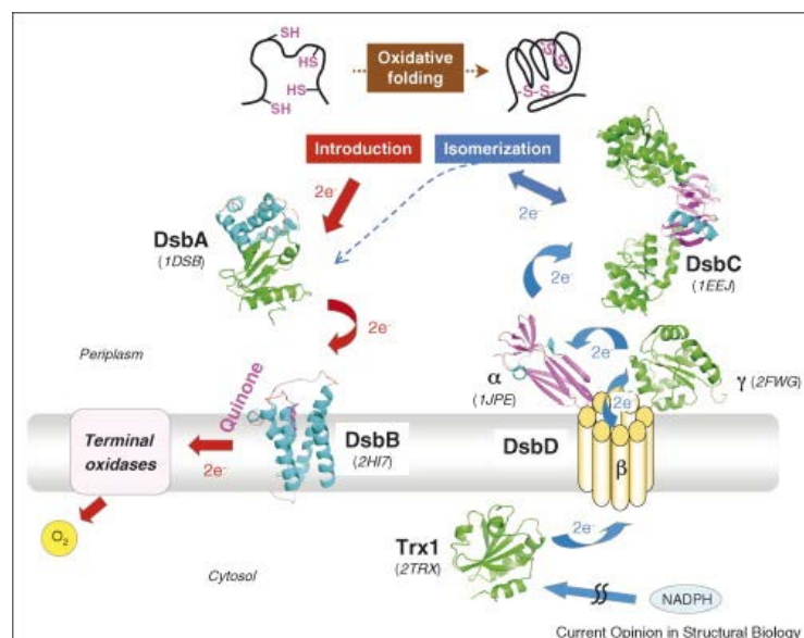
Figure 28 : Présentation du système Dsb d' E. coli impliqué dans le repliement des protéines par la formation de ponts disulfures (Ito et Inaba, 2008).
