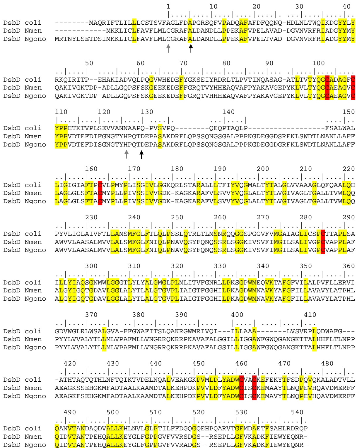
Figure 77 : Alignement des séquences des protéines DsbD d' E. coli , de N. meningitidis et de N. gonorrhoeae . La numérotation indiquée est celle de la nDsbD d' E. coli , les résidus conservés sont surlignés en jaune et les six cystéines essentielles en rouge. Les flèches indiquent les extrémités N- et C-terminales des protéines nDsbD d' E. coli (gris) et de N. meningitidis (noir) produites sous forme soluble.
