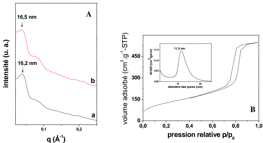
Figure 33 : (A) Diffractogrammes SAXS du matériau préparé à partir de F127 (a) après traitement par NH 3 (g) (b) après lavage à l'éthanol ; (B) isotherme d'adsorption-désorption d'azote et distribution du diamètre des pores du matériau lavé à l'éthanol
