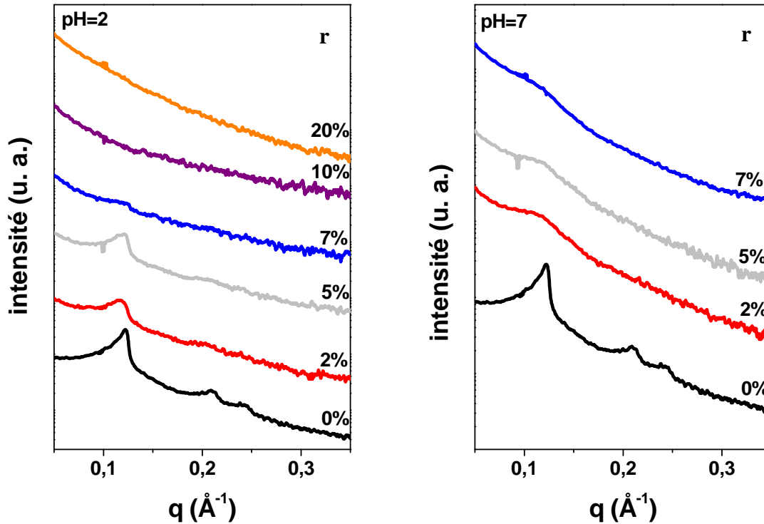
Figure 2 : Diffractogrammes SAXS des matériaux préparés selon le mécanisme CTM à pH=2 et 7 en fonction du taux de titane r
