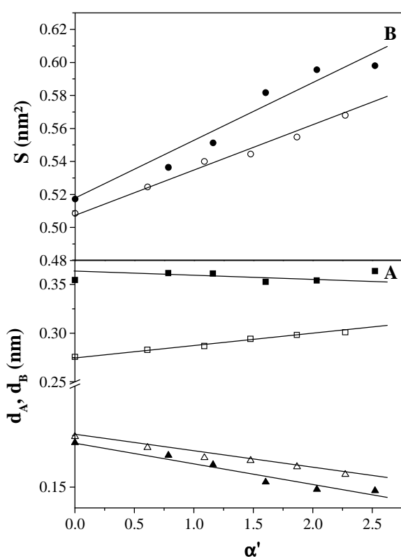
Figure 7 : Système R^F_{7}(EO)_8/CH_3OH/eau : (A) variation de l'épaisseur hydrophobe ( d_B ) et hydrophile ( d_A ) et (B): variation de la surface par tête polaire ( S ) en fonction de \alpha' pour différentes valeurs de R ( R^F_8(EO)_9/eau ) dans la phase lamellaire L\alpha . R = 2,85 , (■) d_A , (▲) d_B , (●) S , R = 5,64 , (□) d_A , (△) d_B , (○) S
