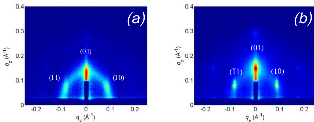
Figure 1 : Clichés GISAXS de films préparés avec \text{TiCl}_4 à partir de la même solution dans différentes conditions (a) dépôt à 12,5 \text{ cm.min}^{-1} sur plaque de silicium, (b) dépôt à 46 \text{ cm.min}^{-1} sur plaque de verre
