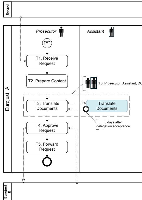
Figure 1: Scénario de délégation MLA
