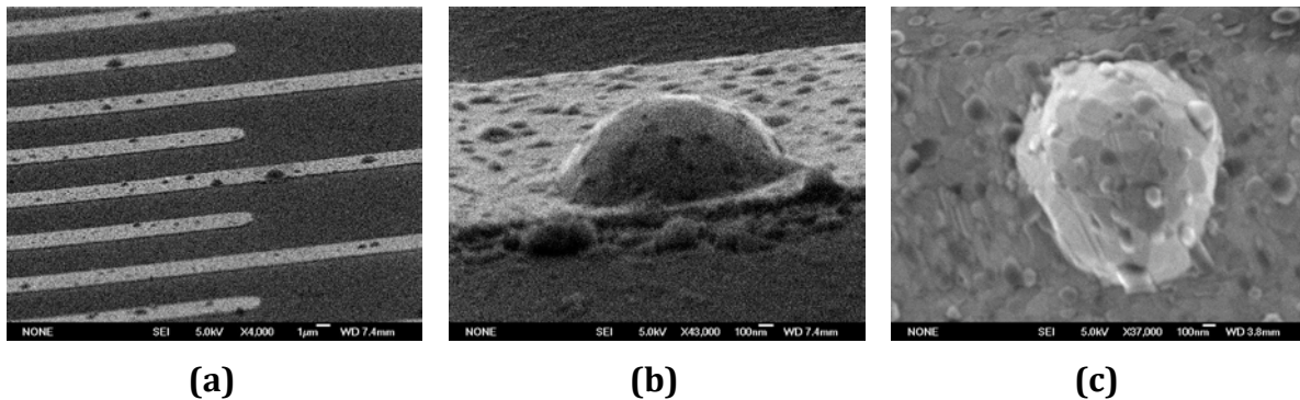
Fig. 2.12 Images MEB d'un IDT en Pt/Co après recuit à 900°C (a), gros plan sur un doigt (b), et sur une "cloque" (c)
