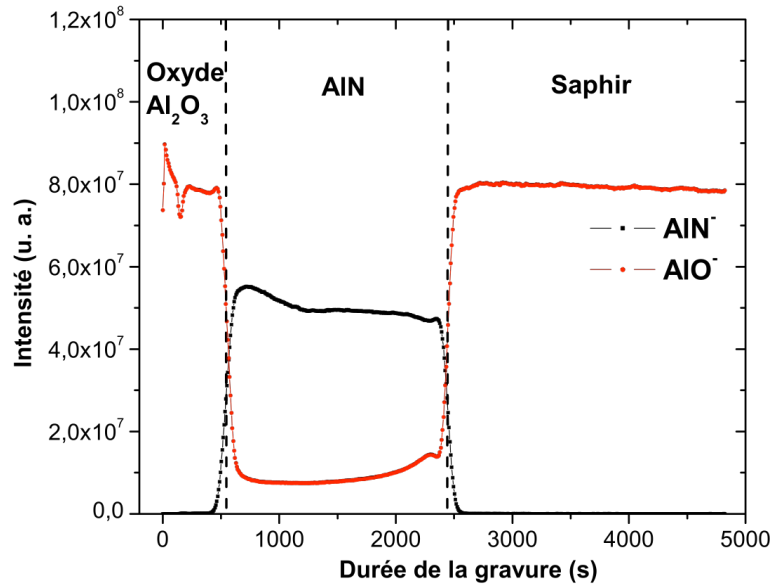
Fig. 5.18 Profil en profondeur de l'échantillon n°= 5 (recuit 2h à 1000°C) obtenu par SIMS. Les oscillations visibles sur le signal AIO - dans la couche d'oxyde surfacique sont liées à des effets de charge, les échantillons traités étant isolants
