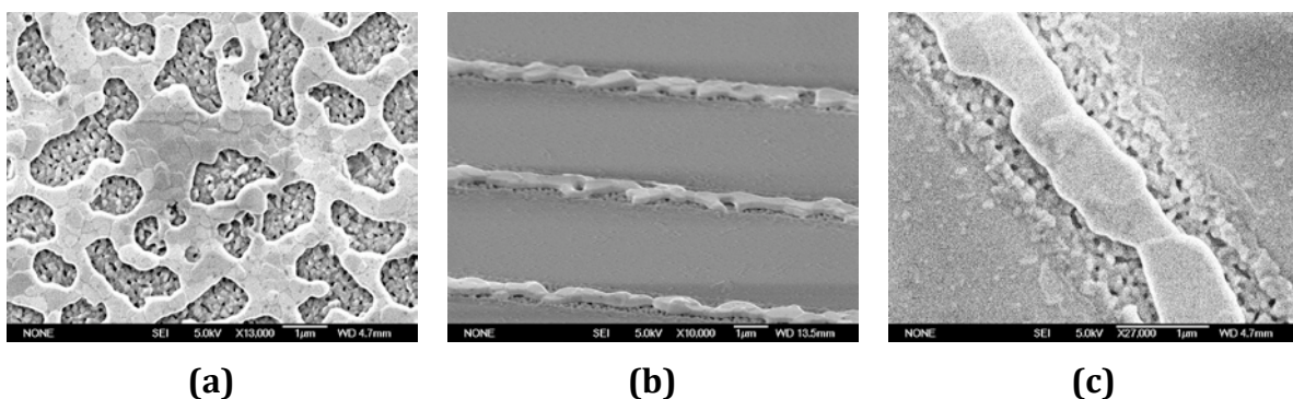
Fig. 2.13 Images MEB d'un IDT en Pt/Co après 30 min. de recuit à 1000°C : gros plan sur le bus (a), vue de profil des doigts (b), gros plan sur un doigt (c)
