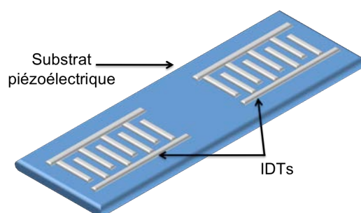
Fig. 1.1 Représentation schématique d'un dispositif SAW de type ligne à retard
