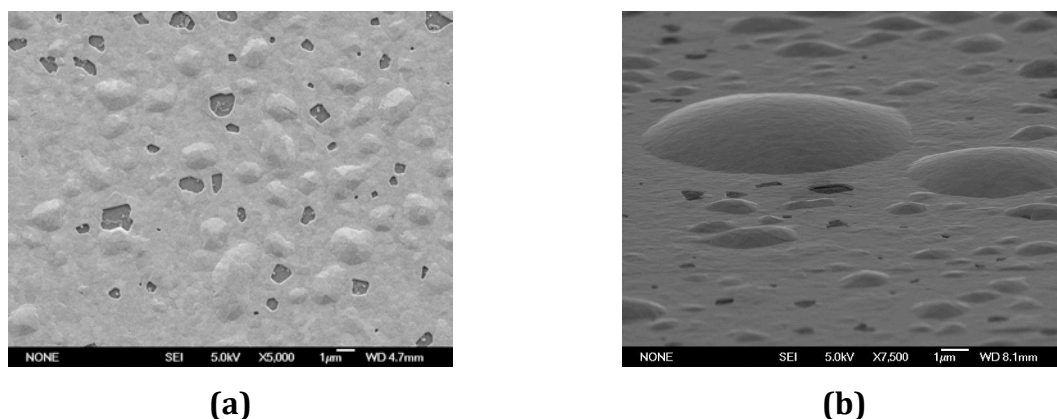
Fig. 2.9 Images MEB du bus de connexion d'un IDT en Pt/Ir suite à 30 minutes de recuit à 1000°C, vue de dessus (a) et en incidence rasante (b)
