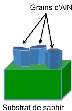
Fig. B.7 Schématisation de la microstructure d'un film d'AlN texturé, orienté (002). Les plans atomiques (002) sont parallèles à la surface du substrat de saphir. Par contre, les grains d'AlN sont, a priori , orientés aléatoirement dans le plan du substrat de saphir.
