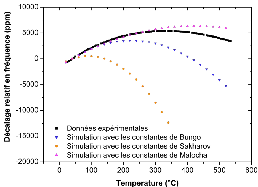
Fig. 3.25 Comparaison de la dérive fréquentielle relative obtenue expérimentalement et par la simulation. Cette dernière a été réalisée par la méthode de Campbell et Jones. La dilatation du substrat avec la température a été prise en compte.
