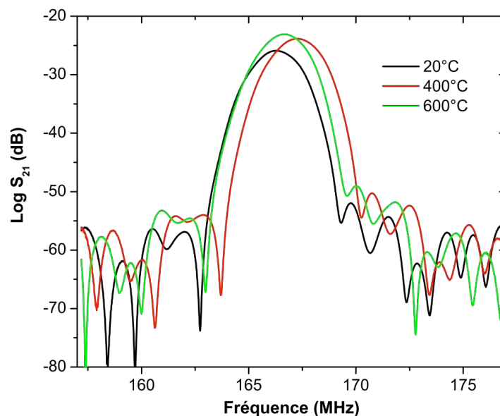
Fig. 3.23 Signal SAW obtenu pour différentes températures
