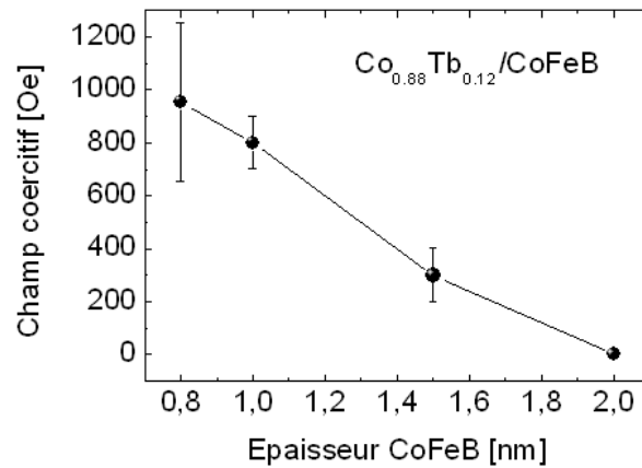
FIG. 4.4 – Cycle d'aimantation et champ coercitif après recuit pour (\text{Co}_{0.88}\text{Tb}_{0.12}) 20\text{nm} / \text{CoFeB} (x \text{ nm}) . Le champ coercitif nul correspond à une aimantation qui s'est couchée dans le plan de la couche.
