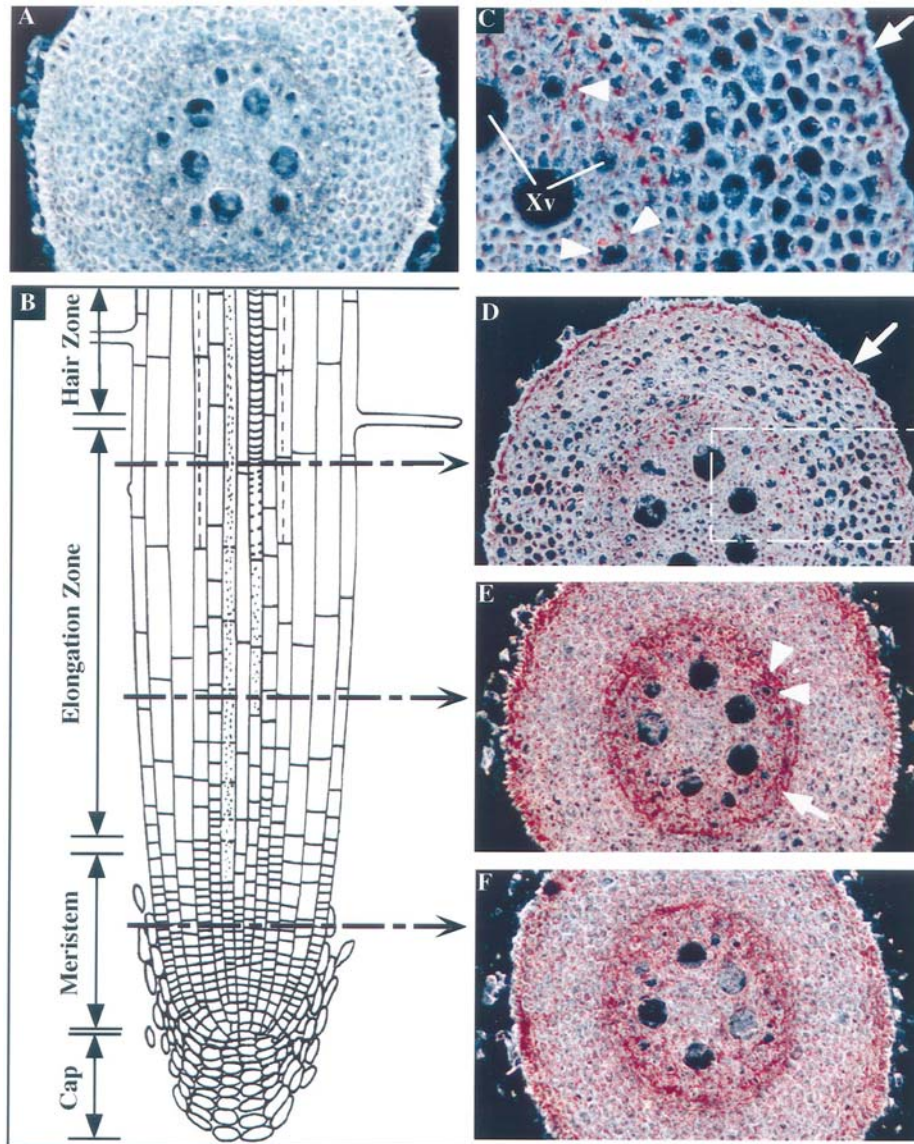
Figure 18 : Localisation des transcrits de ZmTIP1 dans la racine du maïs. Les transcrits sont visualisés (en rouge) par hybridation in situ sur des sections transversales réalisées le long de la racine (A, C-F). A. Contrôle négatif. B. Représentation schématique de la section longitudinale d'une racine de maïs. Les flèches en pointillés indiquent la position des sections transversales D, E et F. C. Grossissement du cadre présent dans la figure D. D. Section transversale en fin de zone d'expansion. Les flèches blanches indiquent la position de l'épiderme. E. Section transversale au milieu de la zone d'expansion. Les flèches blanches indiquent la position de l'endoderme et du péricycle. Les triangles blancs indiquent l'accumulation des transcrits au niveau des cellules du parenchyme qui entourent les vaisseaux du métaxylème. F. Section transversale dans la zone de division. (Barrieu et al. , 1998)
