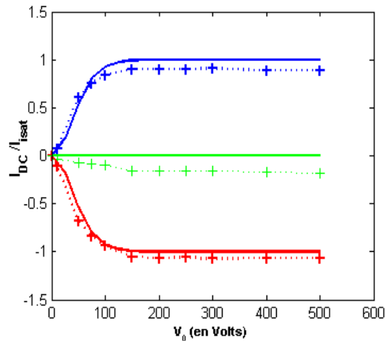
Figure III.24 : Courants DC collectés (normalisé à I_{\text{sat}} ) sur les électrodes sonde (en bleu) et antenne RF (en rouge) en fonction de V_0 (en Volts). En vert le courant DC perpendiculaire. Les paramètres du plasma sont ceux de la série 2 (avec f = 20 MHz). En traits pleins modèle analytique et en pointillés simulations PIC.
