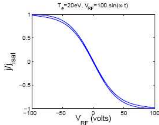
Figure II.22 : caractéristique courant-tension d'un modèle double sonde avec des gaines capacitives. C=0.1 \mu\text{F} .
