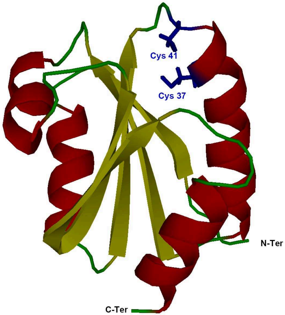
Figure 6 : Structure tridimensionnelle de la Trxh1 de peuplier. PDB: 1T13. On observe les 4 feuilletts \beta au centre de 4 hélices \alpha caractéristiques de la structure “Trx-fold”. Les cystéines du site actif sont représentés en bleu.
