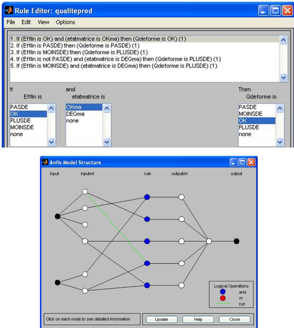
Figure 74. Règles pour l'ANFIS calculant la propriété Qdeforme et la structure associée
