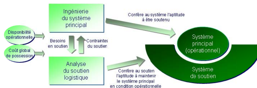
Figure 6. Analyse intégrée du Système de Soutien Logistique (AFIS, 2009)
