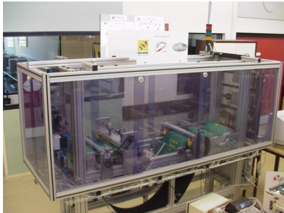
Figure 53. La plateforme TELMA (vue réelle et schématique)
