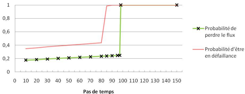
Figure 77. Evolutions temporelles des probabilités de perdre le flux et d'être en défaillance
