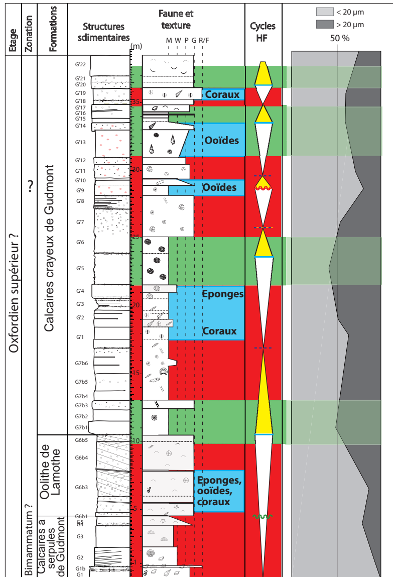
Figure 3.5 Mise en parallèle des associations microfaunistiques obtenus par analyses statistiques et dont les résultats sont décrits dans l'article en Annexe 1 et pourcentages d'éléments PM4 supérieurs ou inférieurs à 20 µm. La couleur rouge est associée aux bancs dominés par le petit benthos (association A, intervalle contenant les maxima transgressifs), la couleur verte colore les bancs dominés par les foraminifères complexes (Association B souvent associée aux maxima régressifs) et la couleur bleue représente les épisodes contenant des nombreux éléments remaniés.
