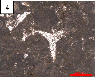
4. Spicule triaxone de spongiaires (G6b1)
