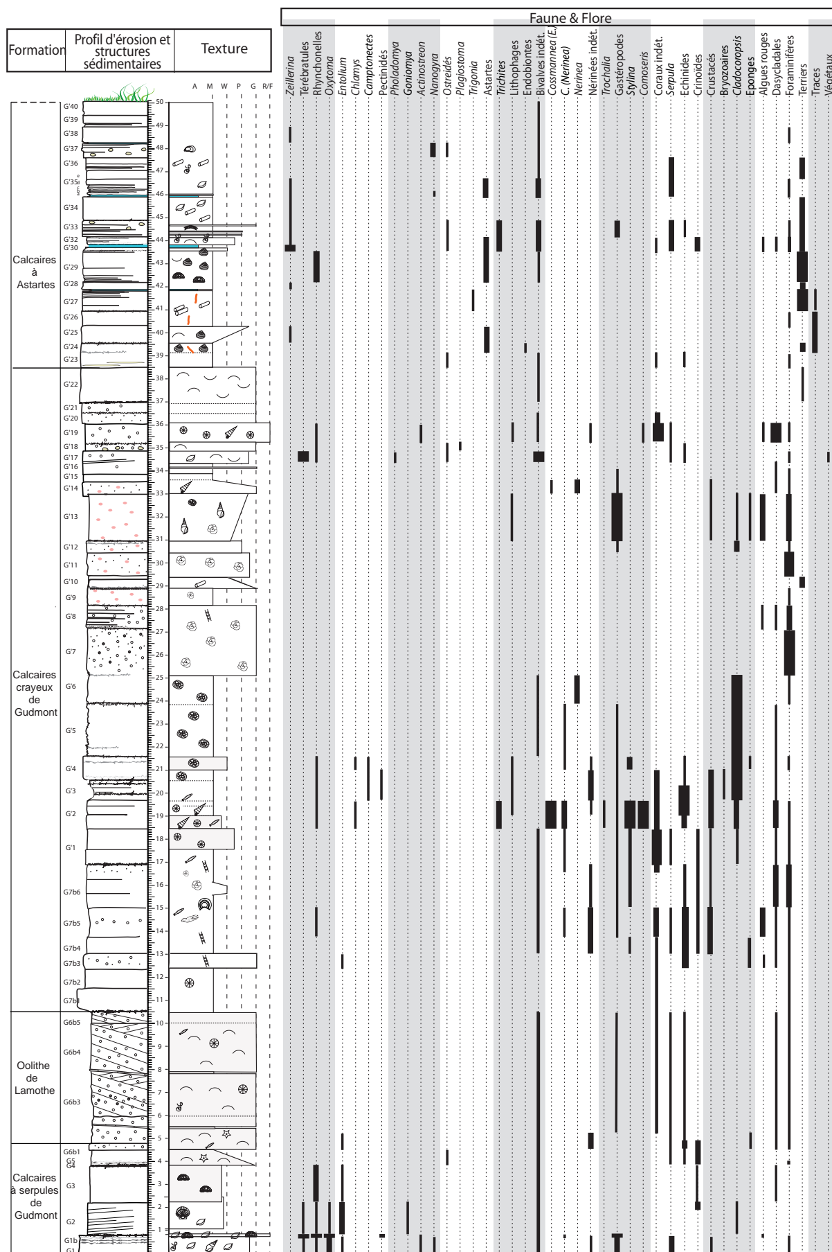
Coupe de Gudmont-Villiers au bord de la route nationale 67
