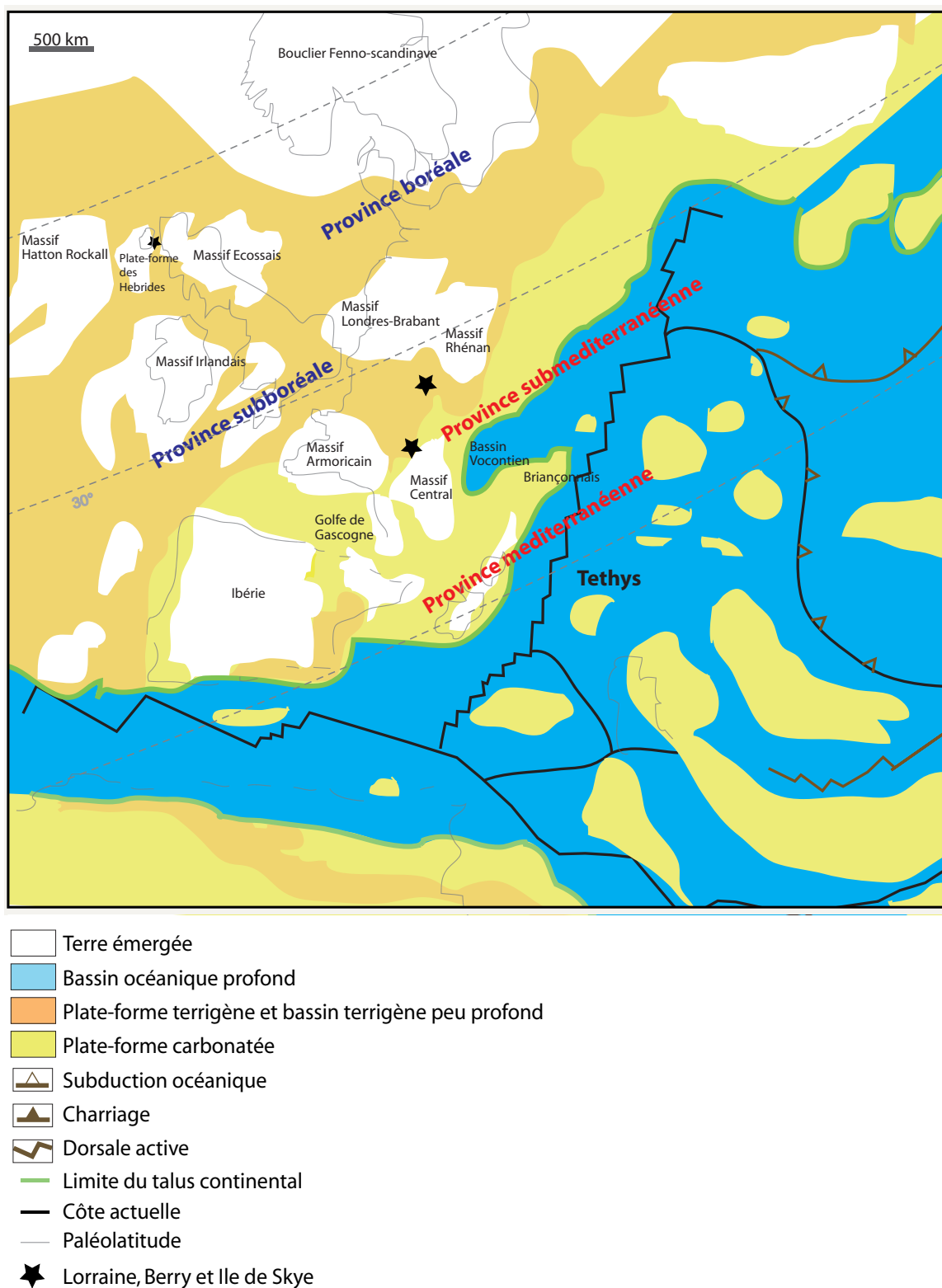
Figure 1.7. Carte paléogéographique de l'Europe de l'Ouest au Kimméridgien inférieur. Simplifié de Cecca in Dercourt et al. (1993) et Thierry in Dercourt et al. (2000).
