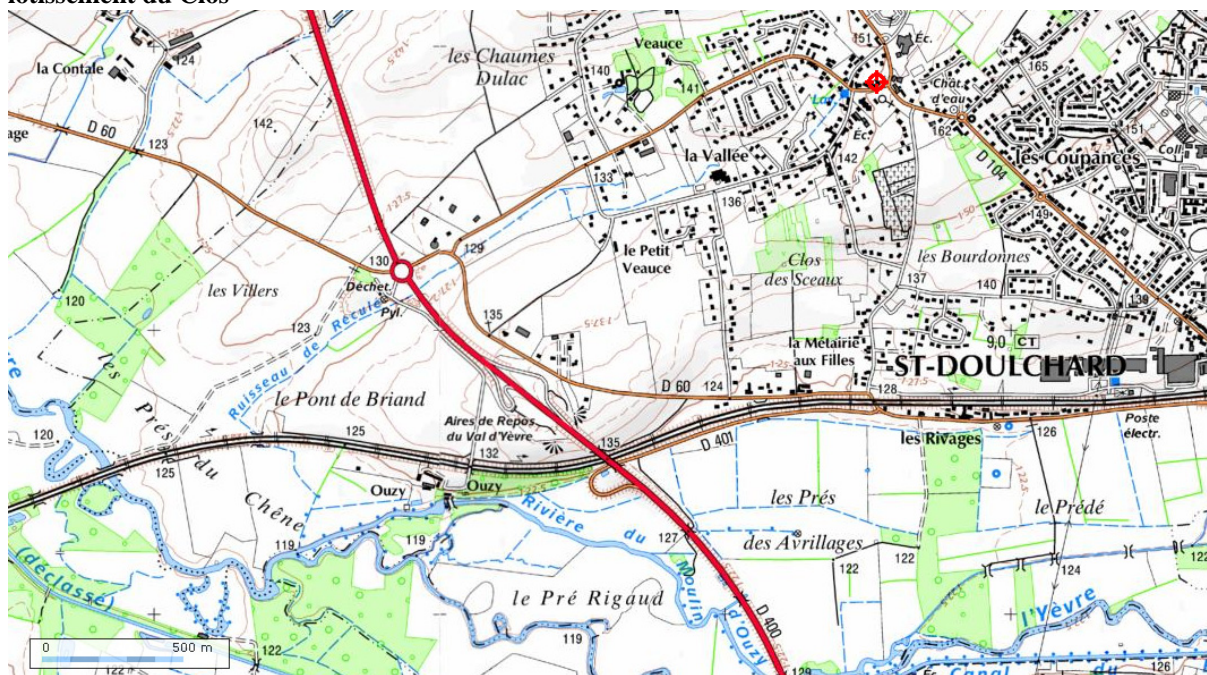
Figure 4.20. Situation géographique des prélèvements effectués au niveau de la construction du lotissement du Clos
