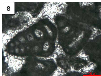
8. Petits agglutinés (Textulariidae) G'8
