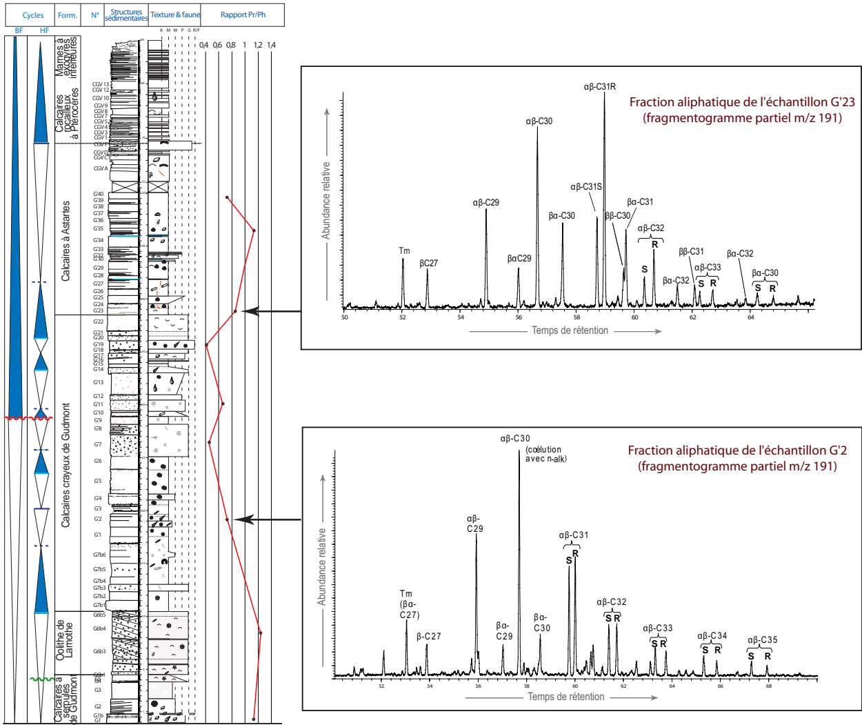
Figure 3.13. Courbe représentant le rapport Pr/Ph calculés dans les échantillons de matière organique soluble de la coupe de Gudmont-Villiers et fragmentogrammes m/z 191 de la fraction aliphatique des échantillons G'2 et G'23 indiquant la présence des isomères R et S des hopanes.
