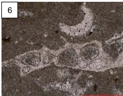
6. Bryozoaires (Calcaires crayeux de Gudmont ; Vi10)
