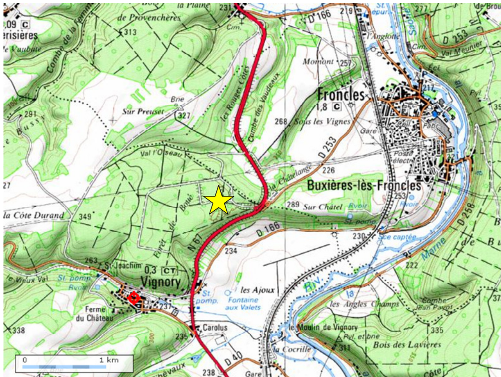
Figure 3.19 Situation géographique de la coupe de Vignory (IGN 1/25000)
