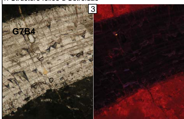
3. Structure prismatique de Trichites
