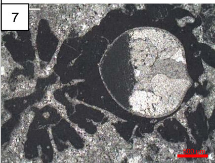
7. Gastrochaenolites dans un corail plocuide G'2
