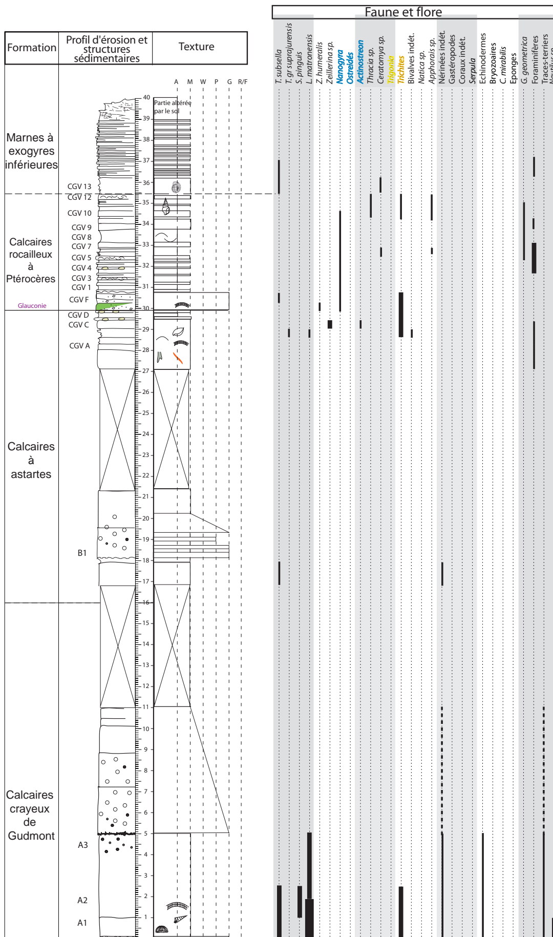
Coupe de Gudmont-Villiers de la carrière Cemex
