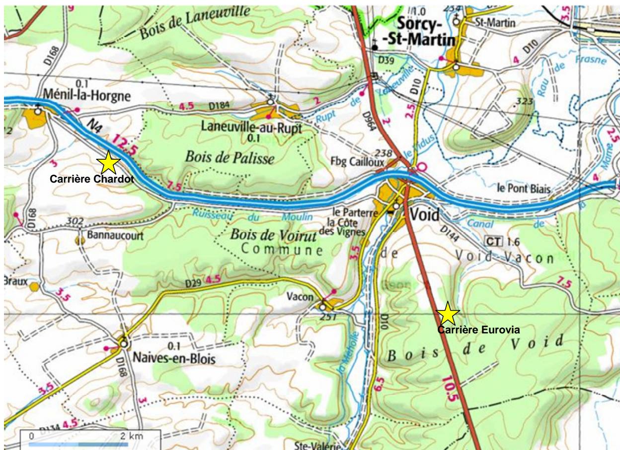
Figure 3.21. Situation géographique des coupes à proximité de Void-Vacon 1. Carrière Chardot proche de la commune de Méné-la-Horgne et 2. Carrière Eurovia
