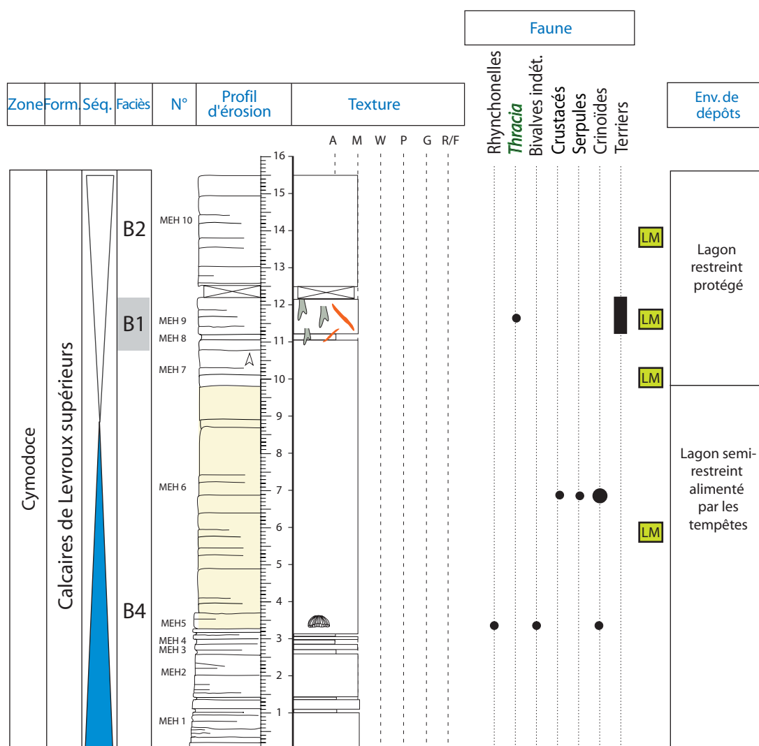
Figure 4.17. Coupe de la carrière de Mehun
