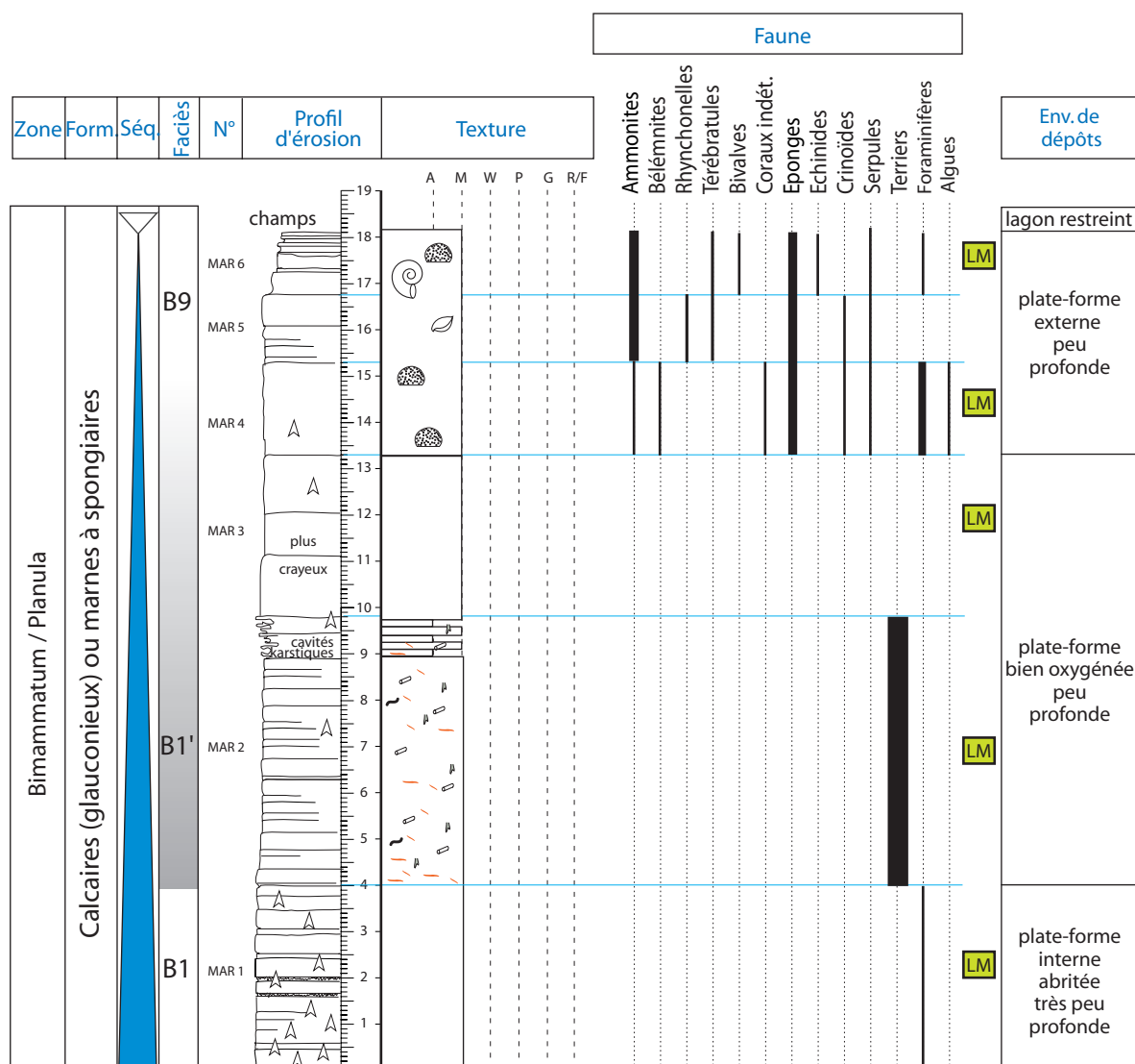
Figure 4.2 Coupe de la carrière de Mâron.
