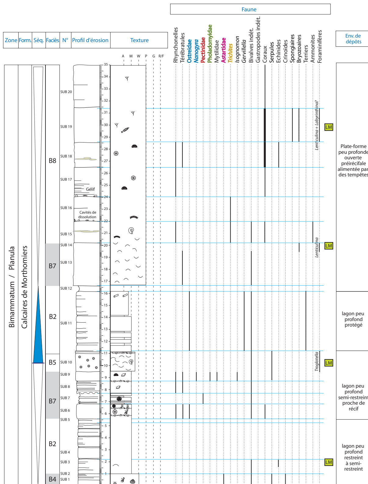
Figure 4.8. Coupe de la carrière du Subdray
