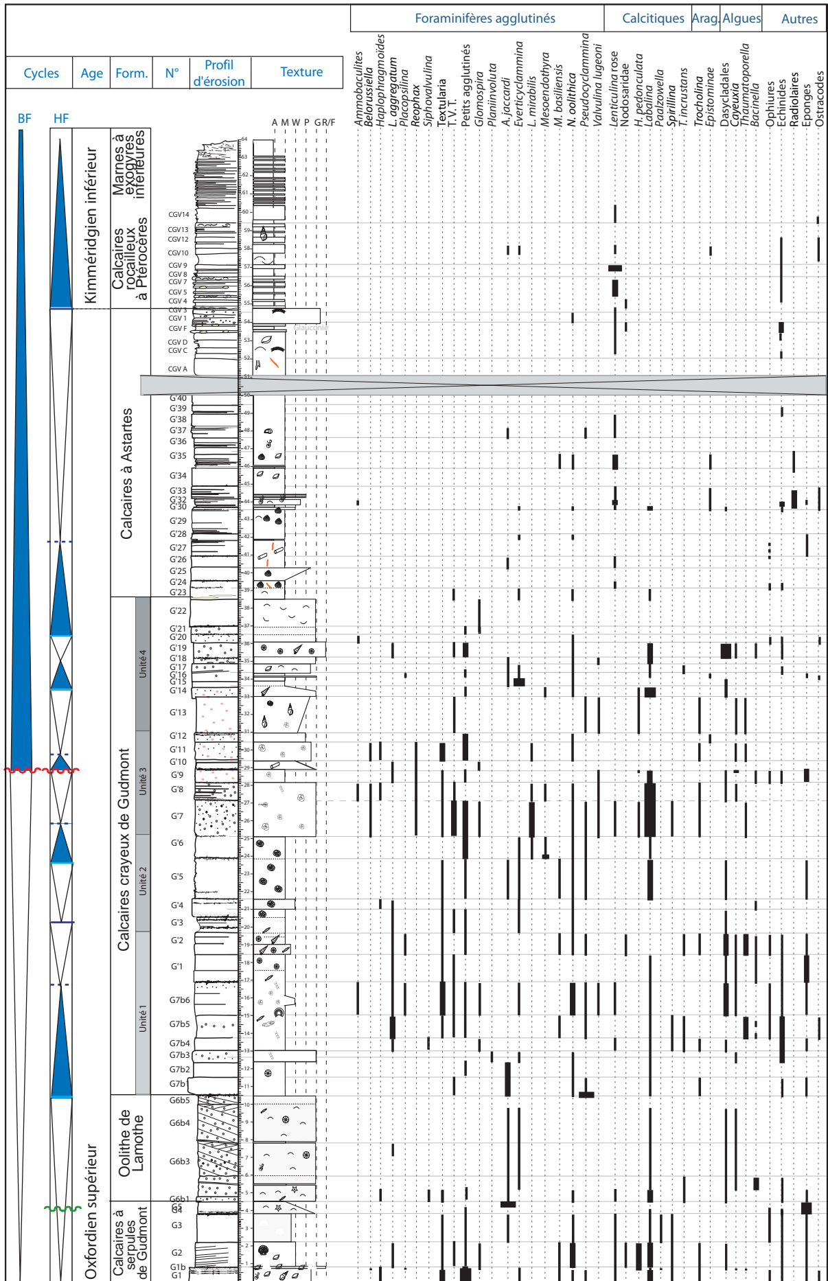
Figure 3.3. Coupe synthétique de Gudmont-Villiers : distribution de la microfaune et courbes de diversité
