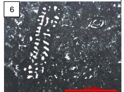
6. Labyrinthina mirabilis (à gauche) et Labalina sp., miliole la plus abondante (G'6)
