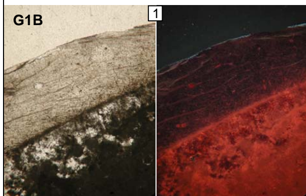
1. Structure foliée d'Ostreidae
