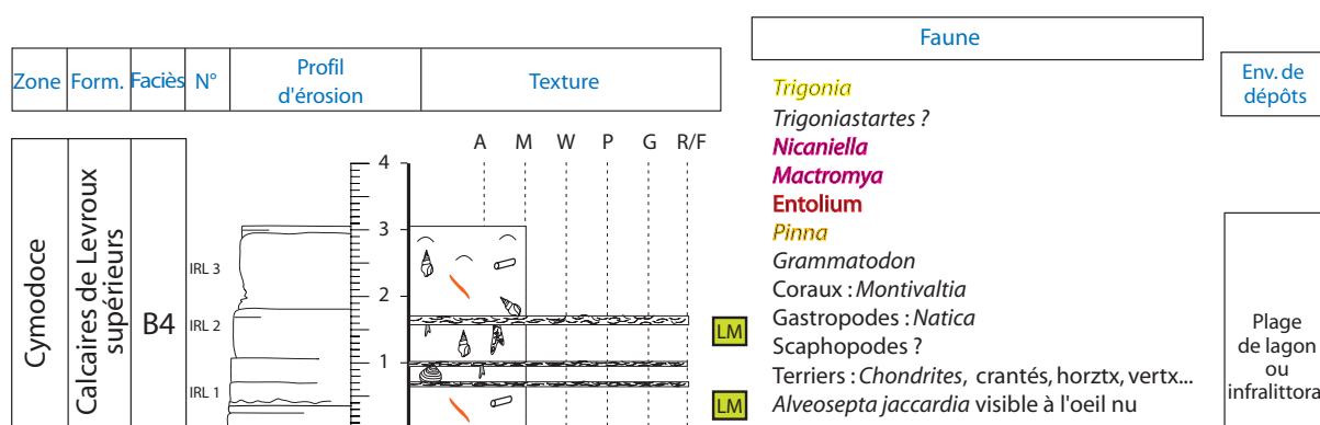
Figure 4.14. Coupe située entre les lieux-dits l'Irlandaise et Bel-Air
