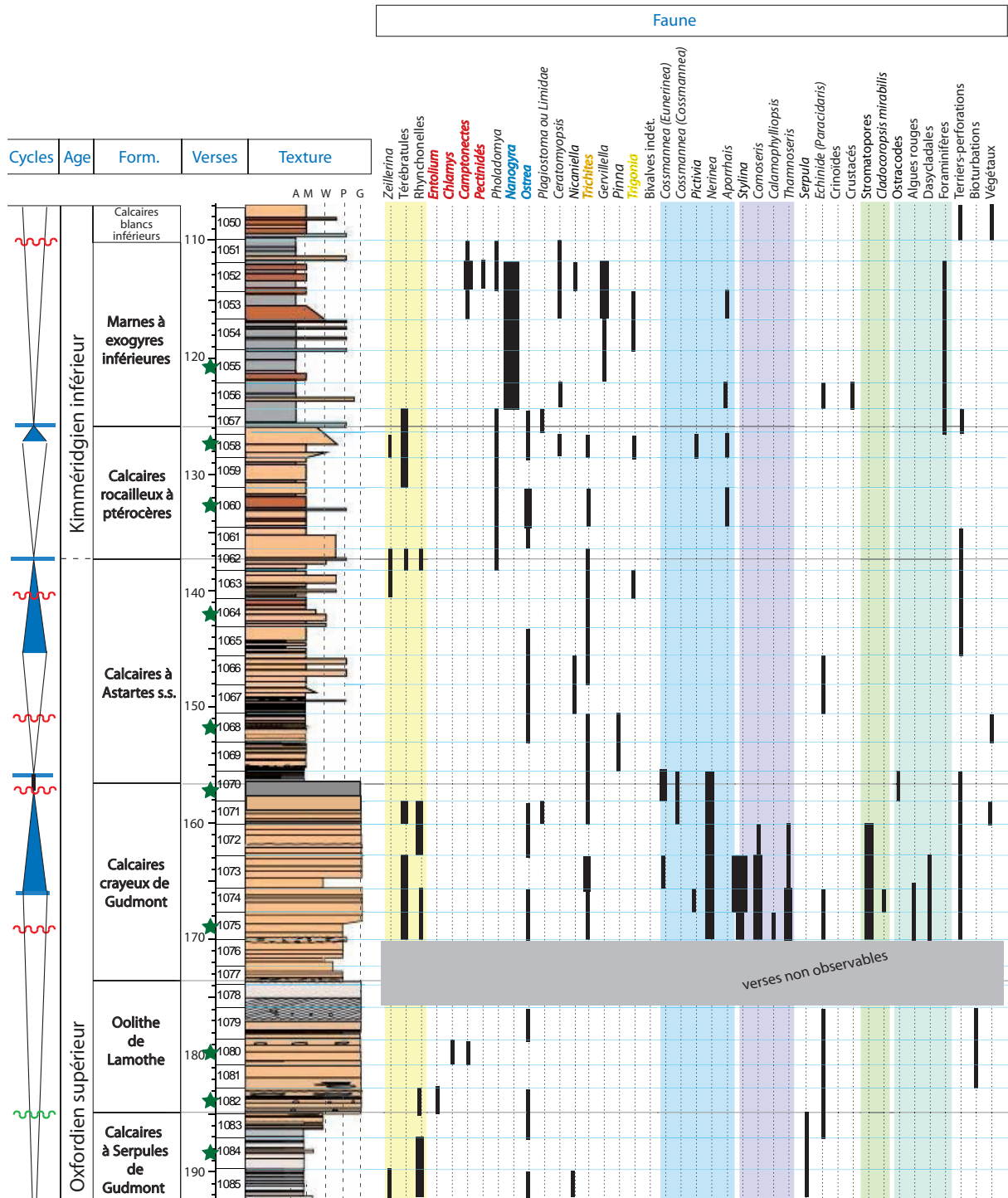
Figure 3.16. Coupe lithologique du puits principal d'accès de Bure, distribution des macrofossiles d'après Lathuilière et al. (2006) et cadre séquentiel. Les étoiles vertes indiquent les verses qui ont été échantillonnées pour l'analyse de la matière organique soluble.
