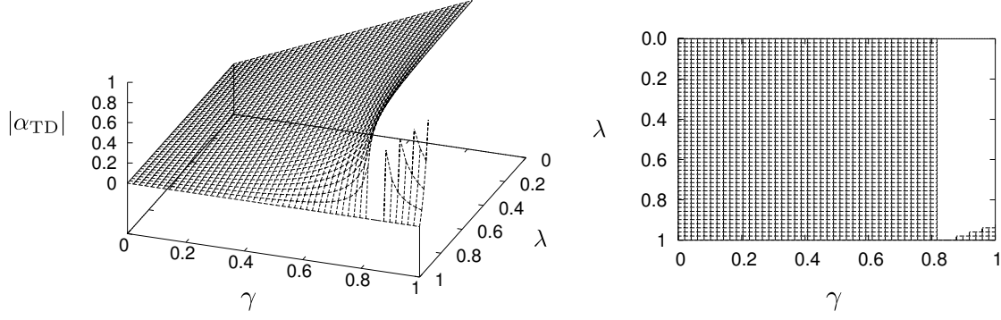
FIGURE 4.2 – Méthode LS \lambda TDQ. Gauche : |\alpha_{TD}| en fonction de \lambda et \gamma . Droite : domaine où |\alpha_{TD}| < 1 .
