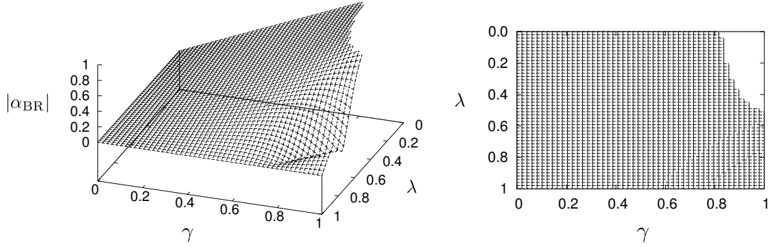
FIGURE 4.3 – Méthode LS \lambda BRQ. Gauche : |\alpha_{BR}| en fonction de \lambda et \gamma . Droite : domaine où |\alpha_{BR}| < 1 .
