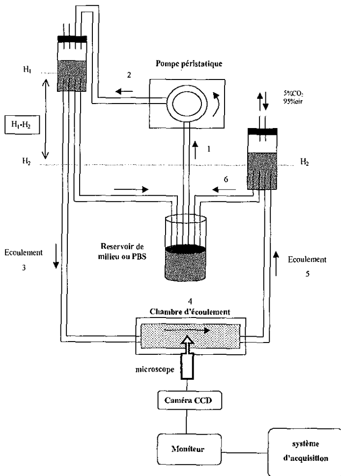
Figure II-3. Circuit d'écoulement.
