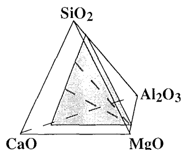
Figure III.17 : Représentation en 3D du quaternaire CaO-MgO-Al 2 O 3 -SiO 2 , le triangle gris représente le système à 15 pds% d'Al 2 O 3 . Les compositions étudiées se trouvent sur les lignes pointillées grises, chaque ligne a un rapport Ca/Si constant et une teneur variable en magnésium.
