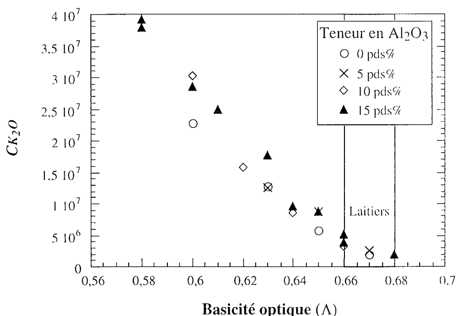
Figure V.5 : Capacité de K_2O en fonction de la basicité optique du liquide silicaté. La zone grisée correspond au domaine des laitiers de hauts fourneaux présentés dans le tableau V.3.
