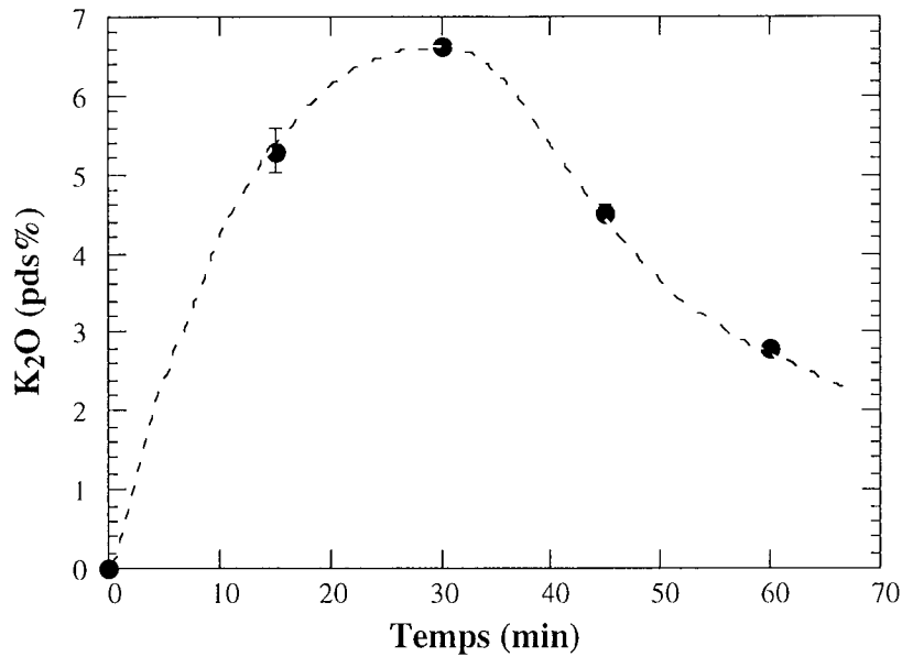
Figure II.8 : Evolution de la teneur en K_2O des échantillons trempés à des temps différents au cours de la même expérience. Expérience réalisée à 1450°C, sous une PO_2 de 10^{-12,4} atm et un débit de gaz de 200 cc/min.
