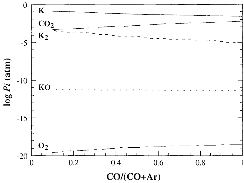
Figure II.3 : Logarithmes des pressions partielles des espèces gazeuses en équilibre avec le mélange K_2CO_3+2C à 1000^\circ C en fonction du rapport CO/(CO+Ar) , (d'après les données de GEMINI1®).
