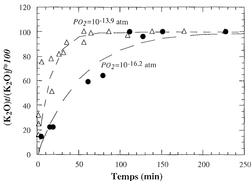
Figure III.6 : Influence de la PO_2 . Teneurs en K_2O à un instant t normalisées à la teneur maximale atteinte dans chacune des expériences. Les triangles correspondent aux résultats obtenus sous une PO_2 de 10^{-13,9} atm et les ronds, à ceux obtenus sous une PO_2 de 10^{-16,2} atm. Les courbes en pointillés correspondent aux équations (K_2O)_t = (K_2O)_{eq} [1 - \exp(-6,65 \cdot 10^{-2} \cdot t)] et (K_2O)_t = (K_2O)_{eq} [1 - \exp(-1,90 \cdot 10^{-2} \cdot t)] .
