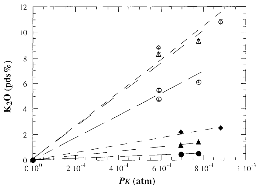
Figure III.18 : Influence de la PK sur la teneur en K_2O à 1410^\circ C sous une PO_2 de 10^{-13.9} atm pour des liquides contenant 15 pds% d' Al_2O_3 et des teneurs en MgO variables. Les symboles pleins et vides représentent les liquides de type CMASx/15-1 et CMASx/15-4. Les triangles, ronds et losanges correspondent à des teneurs en MgO de 0, 2.5 et 15 pds% respectivement. Les barres d'erreur ont été également reportées.
