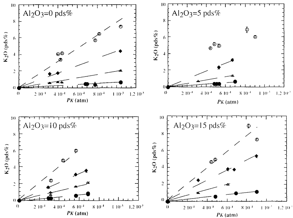
Figure III.15 : Influence de la PK sur la teneur en K_2O à 1410^{\circ}C sous une PO_2 de 10^{-13,9} atm pour des compositions à teneur en Al_2O_3 variables. Dans chaque cas, les ronds noirs, les triangles, les losanges et les ronds blancs représentent les compositions de type CMAS10/x-1, CMAS10/x-2, CMAS10/x-3 et CMAS10/x-4 respectivement ( x=0, 5, 10, 15 pds% d' Al_2O_3 ). Les barres d'erreur sont également reportées.
