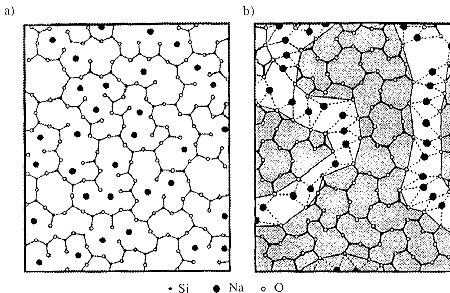
Figure I.2 : Schéma bi-dimensionnel d'un réseau silicaté. a.) d'après le modèle CRN (Continuous Random Network) de Zachariasen (1932) et b.) d'après le modèle MRN (Modified Random Network) de Greaves et al. (1981).
