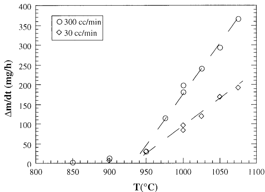
Figure II.14 : \Delta m/dt en fonction de la température et du flux de gaz. Les cercles et les losanges représentent les résultats obtenus sous des flux de 300 et 30 cc/min respectivement.
