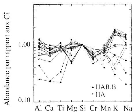
Figure V.3 : a.) Compositions globales de chondres de type IAB, IB et IA de la météorite de Semarkona en termes d'abondance relative à Si et CI, d'après Jones (1994) et b.) compositions globales de chondres de type IIB, IIB et IIA de la météorite de Semarkona d'après Jones (1996).
