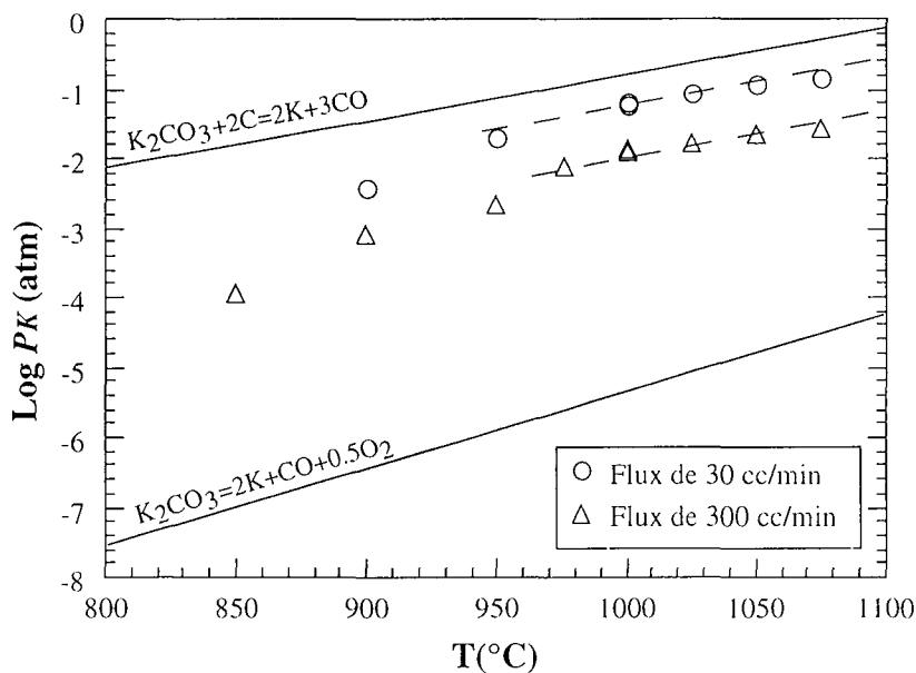
Figure II.15 : Logarithmes des pressions partielles de potassium calculées d'après l'équation II.9, pour des flux de 30 cc/min (cercles) et 300 cc/min (triangles), à différentes températures. Les deux droites représentées correspondent aux valeurs calculées à partir des données thermodynamiques pour les équations K_2CO_3 + 2C = 2K + 3CO et K_2CO_3 = 2K + CO + 1/2O_2 . Quand la température est supérieure à 950^{\circ}\text{C} , la courbe des PK expérimentales suit celle des PK théoriques (traits pointillés).
