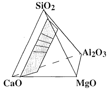
Figure III.14 : Représentation en 3D du quaternaire CaO-MgO-Al 2 O 3 -SiO 2 . Les compositions étudiées se trouvent sur les lignes grises.
