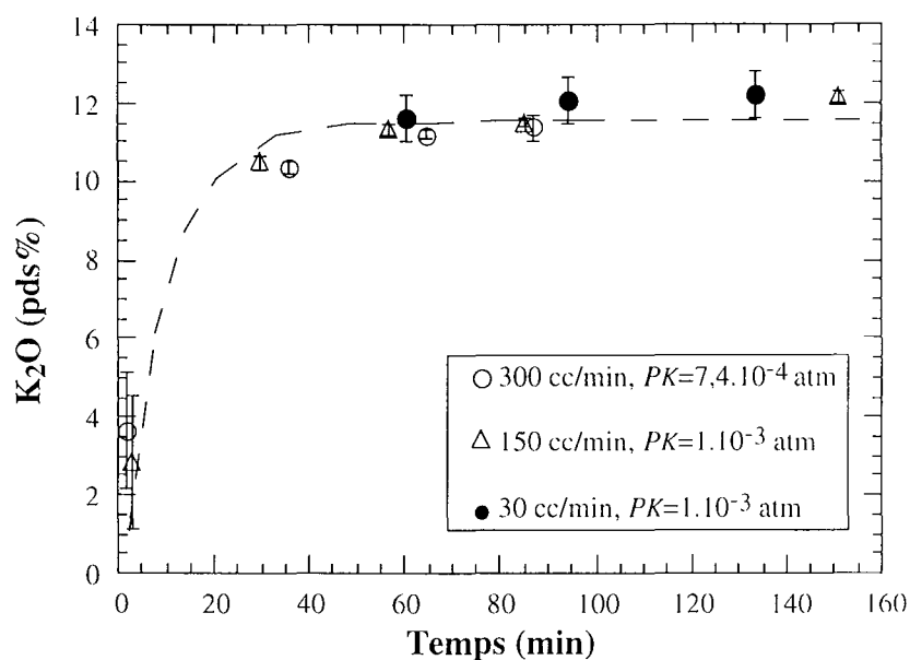
Figure III.1 : Influence du flux de gaz sur la teneur en K_2O à l'équilibre dans le liquide CMAS1, à 1410^\circ C sous une PO_2 de 10^{-13,9} atm (cf.§.II.5.2). Les ronds noirs, triangles et ronds blancs correspondent aux expériences réalisées sous des flux de 30, 150 et 300 cc/min respectivement. Les barres d'erreur correspondent aux écart-types obtenus sur des profils de n ( 10 \leq n \leq 20 ) points réalisés à la sonde électronique.
