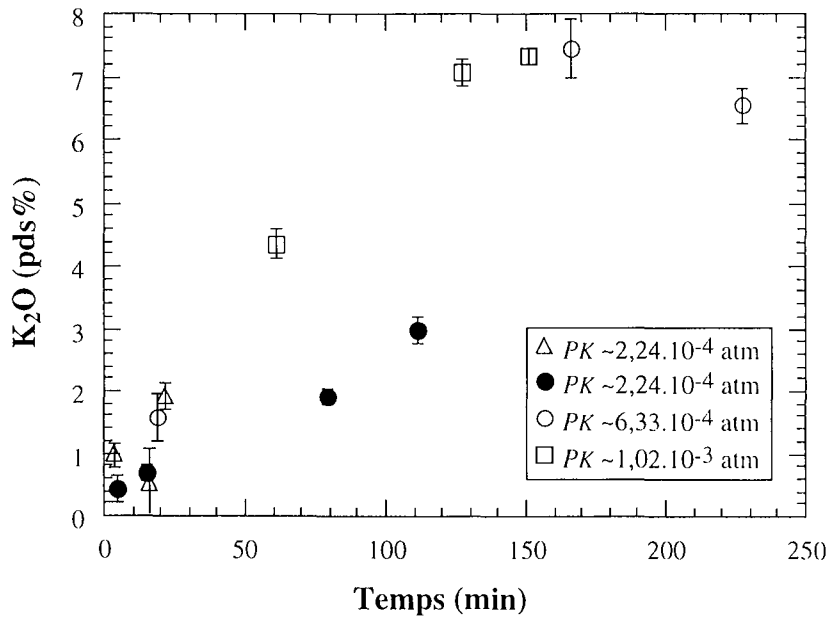
Figure III.5 : Evolution de la teneur en K_2O des échantillons de composition CMAS1 en fonction du temps à 1410^\circ C sous PO_2=10^{-16.2} atm et sous différentes PK . Les barres d'erreur correspondent aux écart-types obtenus sur les profils de n points ( 10 \leq n \leq 20 ) réalisés à la sonde électronique.
