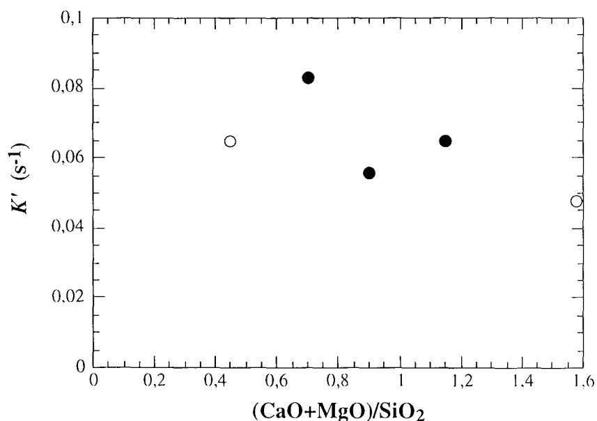
Figure IV.4 : Evolution de la constante de condensation K' en fonction de l'indice de basicité du liquide silicaté. Sont reportés les résultats de cette étude (ronds blancs) et ceux obtenus par Amatatsu et al. (1985) (ronds noirs).
