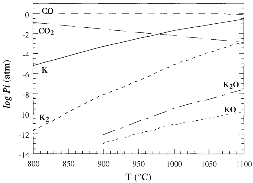
Figure II.4 : Logarithmes des pressions partielles des espèces gazeuses en équilibre avec le mélange K_2CO_3+2C en fonction de la température sous atmosphère de CO, (d'après les données de GEMINI1®).
