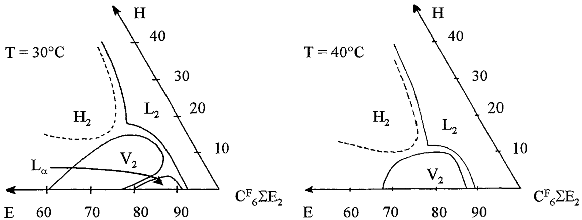
Figure 20. Diagrammes de phase du système C_6F_{13}E_2 /eau/PFD à différentes températures.
