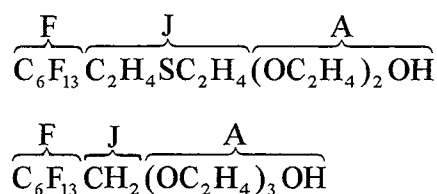
Figure A.1. Représentation schématique des molécules de tensioactif
