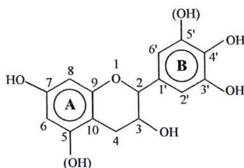
Figure 1. structure d'un monoflavonoïde.
