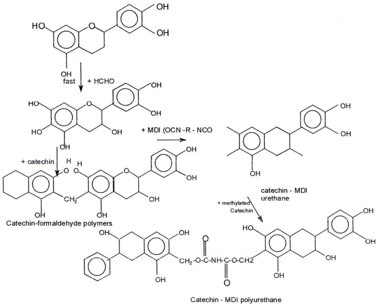
Figure 26. Réaction du système tanins/ PMDI [59]
