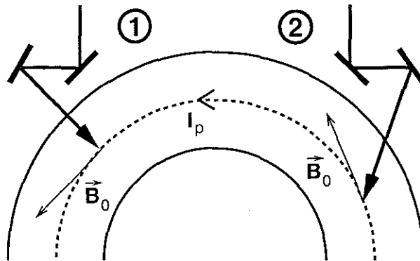
FIG. 2.12 – Principe du chauffage (situation (1)) et de la génération de courant (situation (2)) par utilisation d'un système de miroirs orientables pour l'injection des ondes cyclotroniques électroniques.
