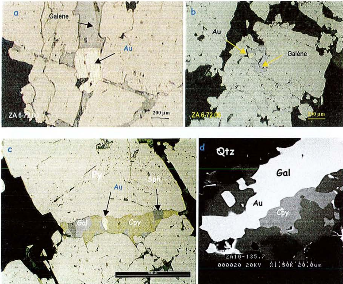
Planche III-25 : Relations entre or, galène et barytine observées dans les échantillons de La Zarza ; a et c (LR) Or associé à la galène et à la chalcopyrrite dans une microfissure dans la pyrite ; b) LR, Or et galène dans un porphyroclaste de pyrite ; d) relation or galène observée au MEB-EDS.
