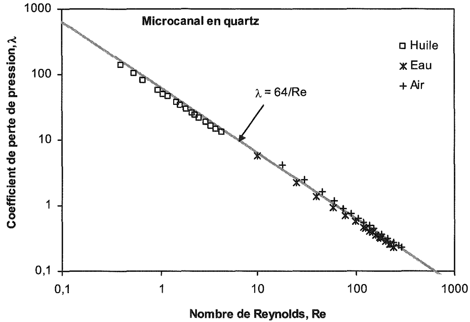
Figure 16 : Coefficient de perte de pression en fonction du nombre de Reynolds. Microcanal en quartz.
