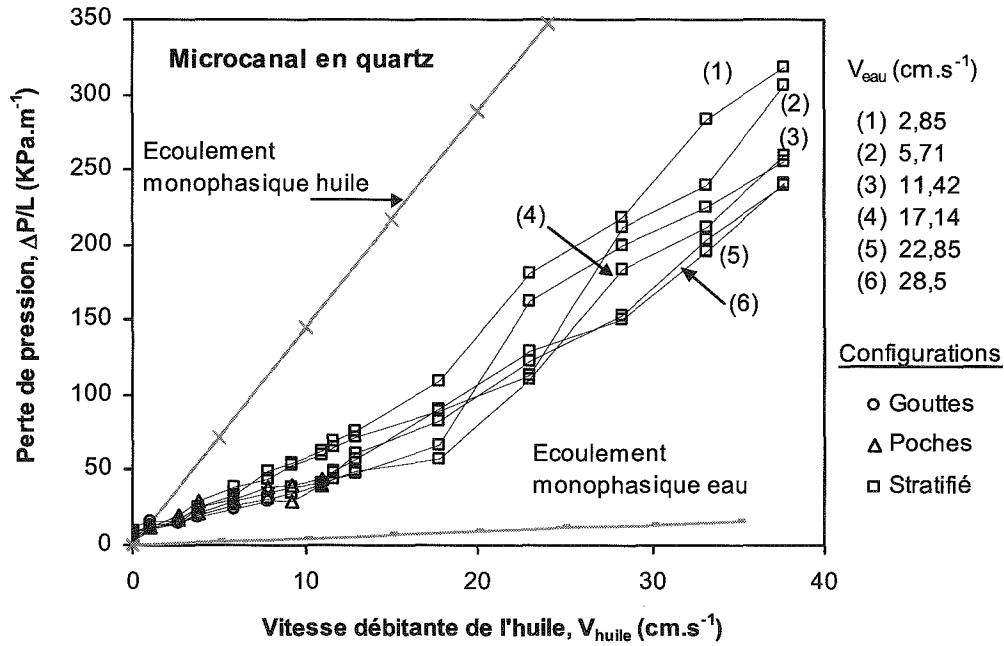
Figure 14: Perte de pression ( \Delta P/L ) en fonction de la vitesse débitante de l'huile ( V_{huile} ) pour l'ensemble des vitesses débitantes de l'eau ( V_{eau} ) étudiées. Microcanal en quartz.
