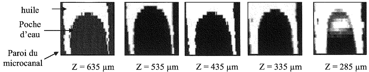
Figure 19 : Images négatives (64 x 64) des poches d'eau dans l'huile suivant les différents niveau Z du microcanal en verre.
