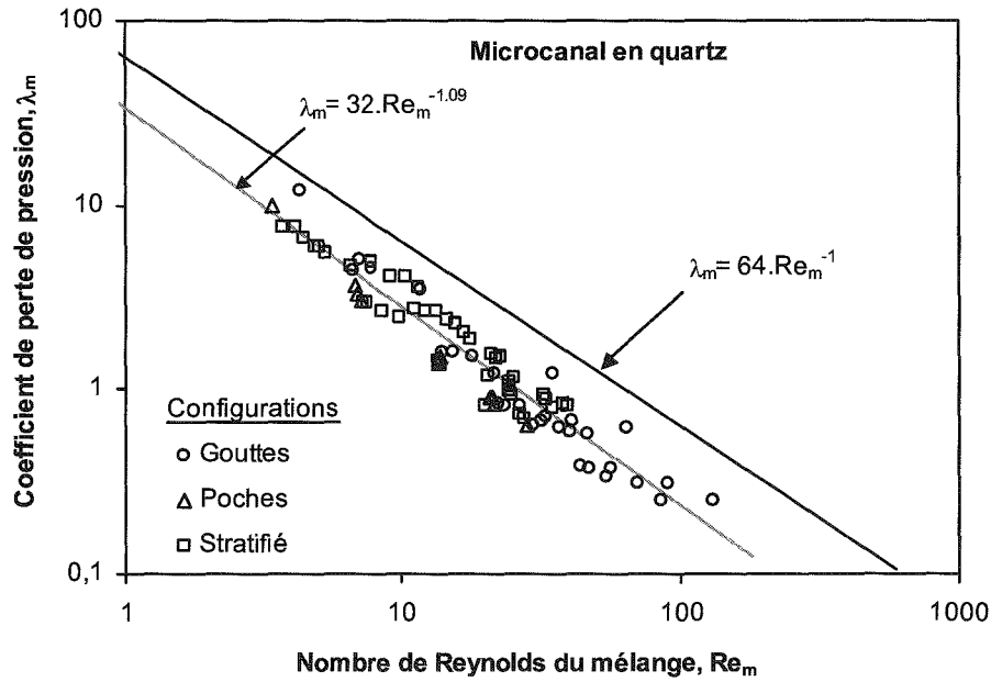
Figure 27 : Coefficient de perte de pression ( \lambda_m ) en fonction du nombre de Reynolds du mélange ( Re_m ). \mu_m est déterminée par la relation de Cicchitti et al. (1960). Microcanal en quartz.
