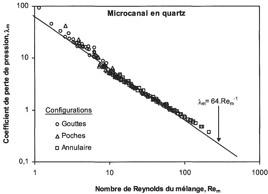
Figure 24 : Coefficient de perte de pression ( \lambda_m ) en fonction du nombre de Reynolds du mélange ( Re_m ). \mu_m est déterminée par la relation de Cicchitti et al. (1960). Microcanal en quartz initialement saturé en huile.
