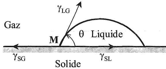
Figure 1 : Schématisation des forces en présence entre les trois phases en équilibre.
