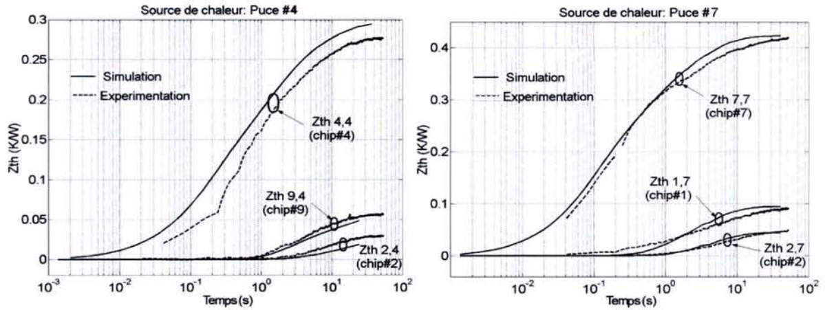
Fig.88: Résultats et corrélation entre calculs numériques et essais expérimentaux pour des impédances propres et mutuelles
