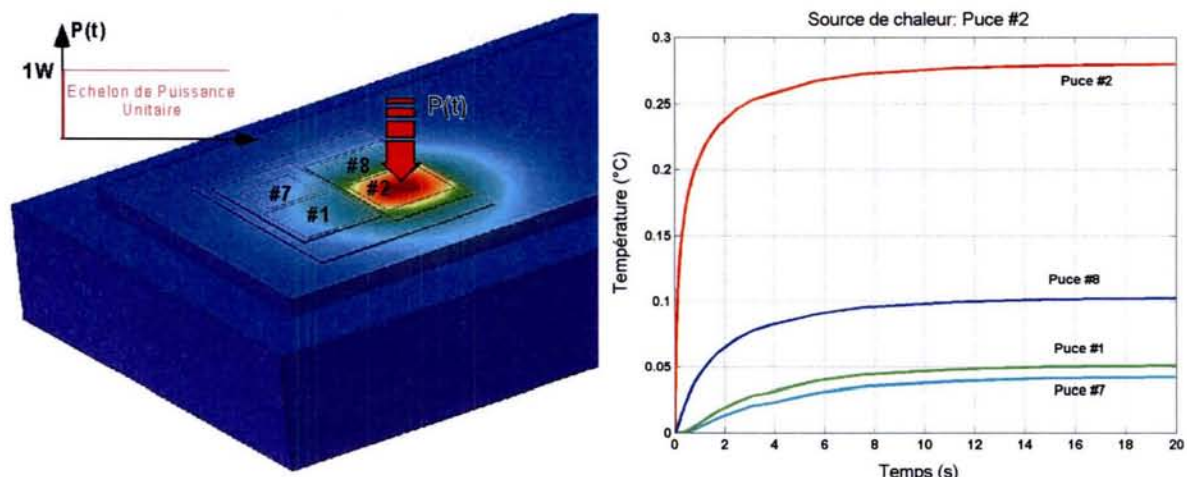
Fig.83: Résultats de simulation 3D, en dynamique, du comportement thermique du convertisseur multichip soumis à une puissance de 1 W sur une puce et avec T_{ref}=0^{\circ}\text{C}
