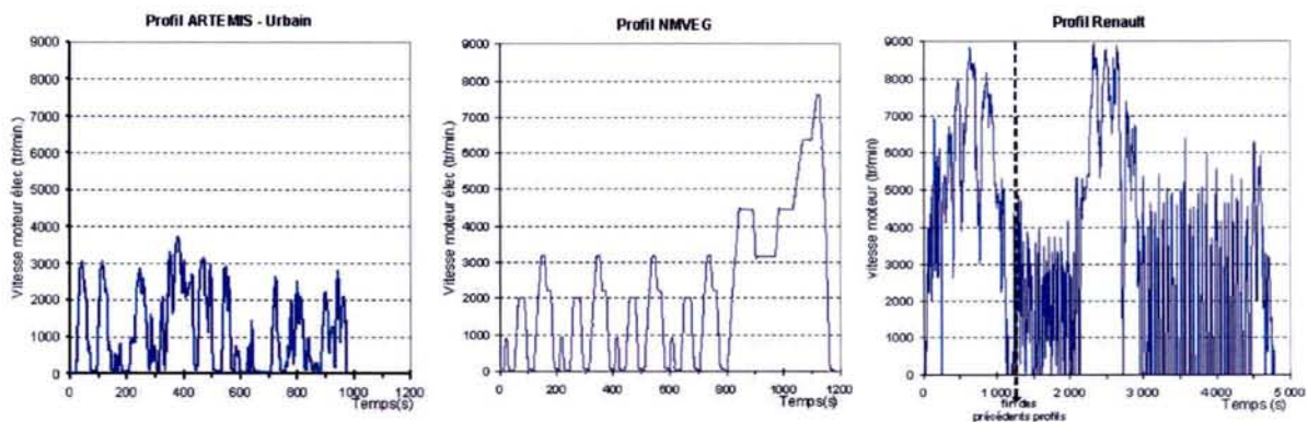
Fig.40: Régime moteur du véhicule électrique sur divers profils de mission
