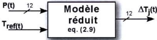
Fig.90: Schéma synoptique du modèle thermique réduit
