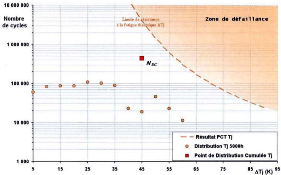
Fig.71: Corrélation graphique entre la courbe de résultat du Power Cycling Test et la distribution de température de T_j pour le profil de référence Renault
