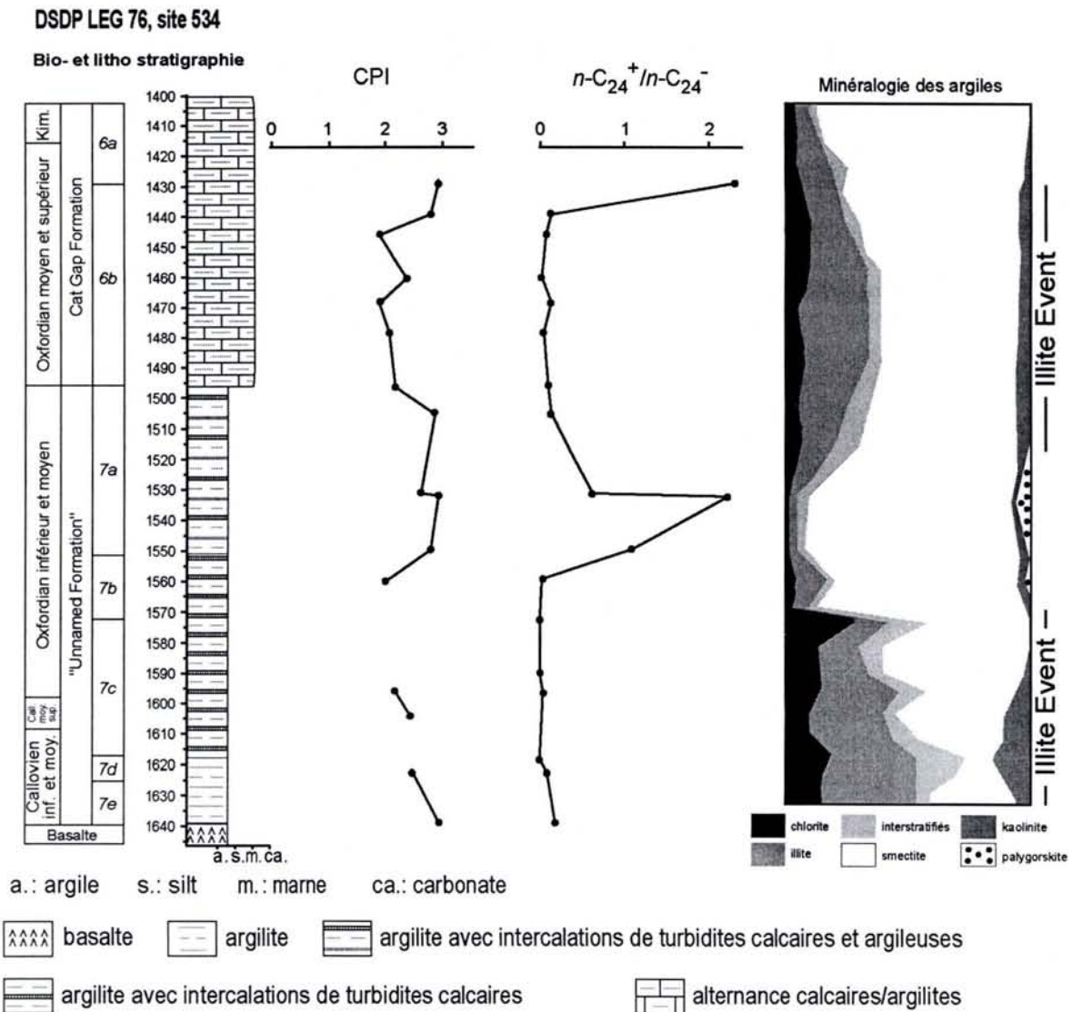
Figure VI.14. Evolution stratigraphique de l'indice CPI et du rapport n-C_{24}^+ / n-C_{24}^- pour le puits DSDP 534A. Les valeurs non calculées des CPI correspondent aux échantillons dont les n -alcanes à chaîne longue ( n-C_{24}^+ ) sont sous le seuil de détection.
