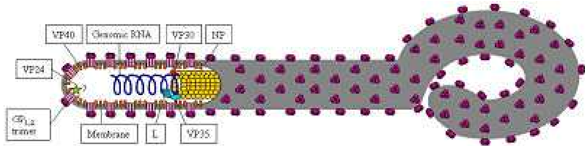
Figure 9 : Représentation schématique de la structure d' Ebolavirus . L représente l'ARN polymérase, GP correspond à la glycoprotéine, NP à la nucléoprotéine, et VP aux protéines virales structurales.
