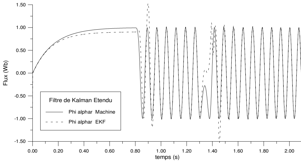
Figure 5.9 Evolution du flux rotorique ( composante alpha )
