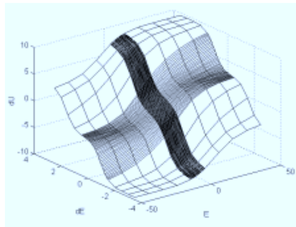
Figure 2.67 Résultat de l'apprentissage.
