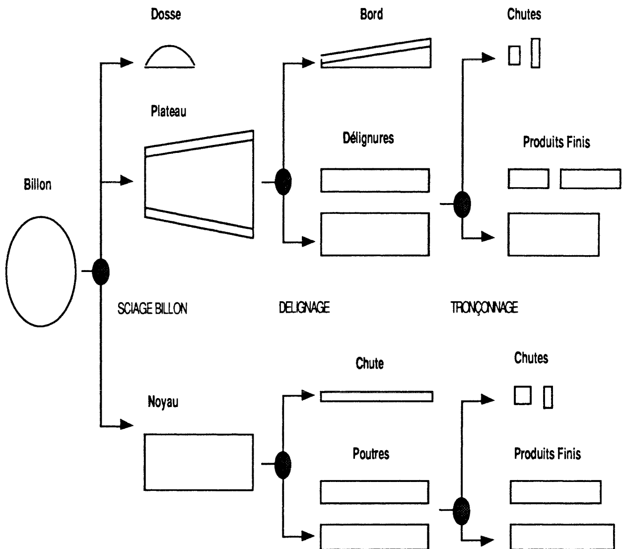
Figure 4.10. Les points de séparation des produits liés dans une scierie
