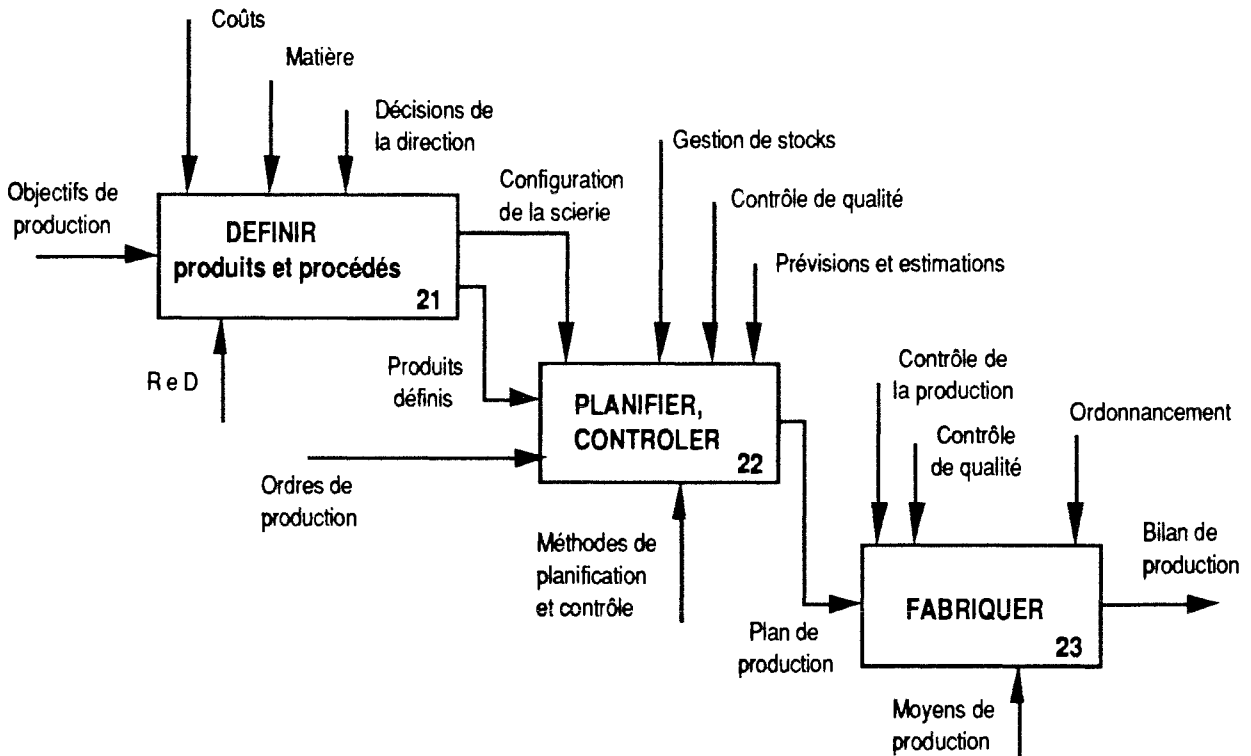
Figure 2.2. Diagramme A2: Produire
