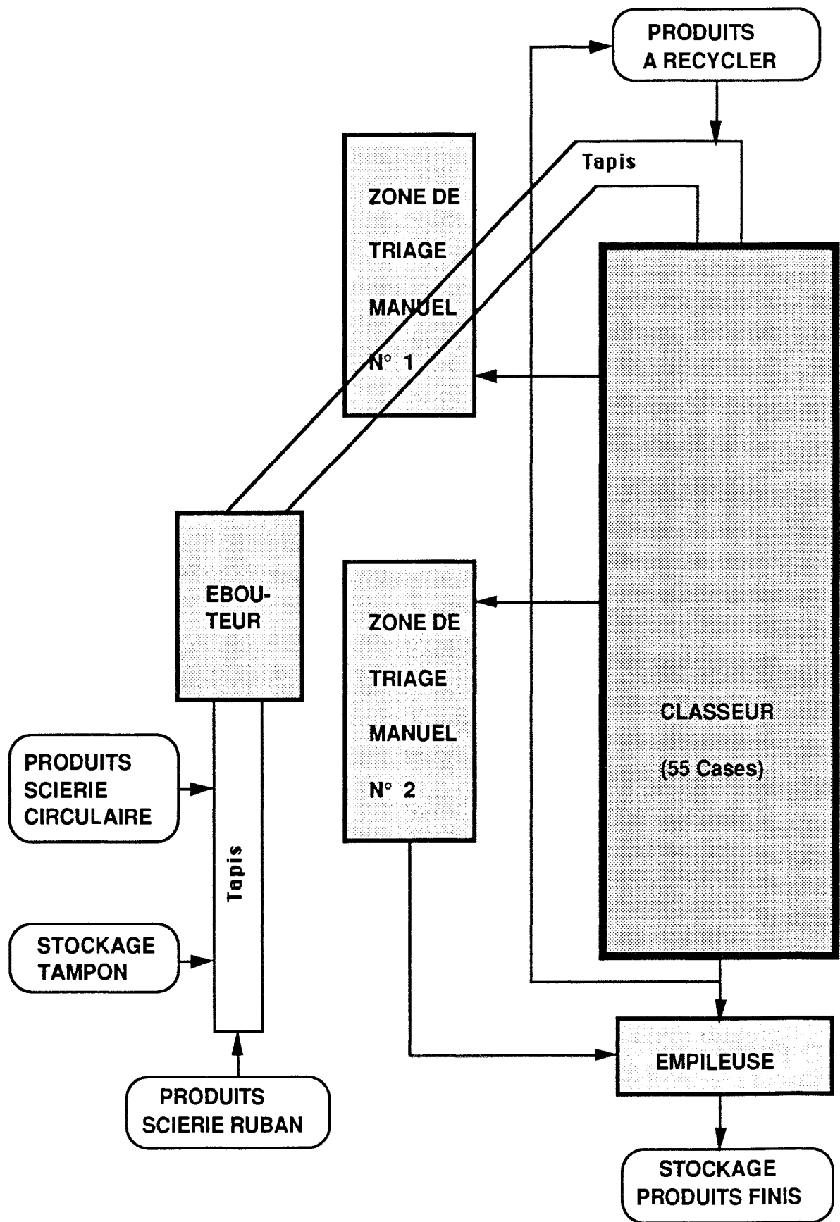
Figure 5.40. Le classeur automatisé
