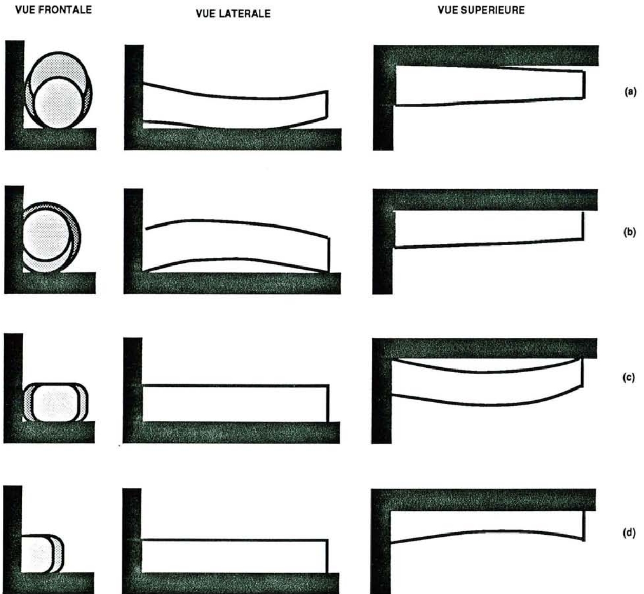
Figure A1.3. Positions du billon sur le chariot de la scie-de-tête
