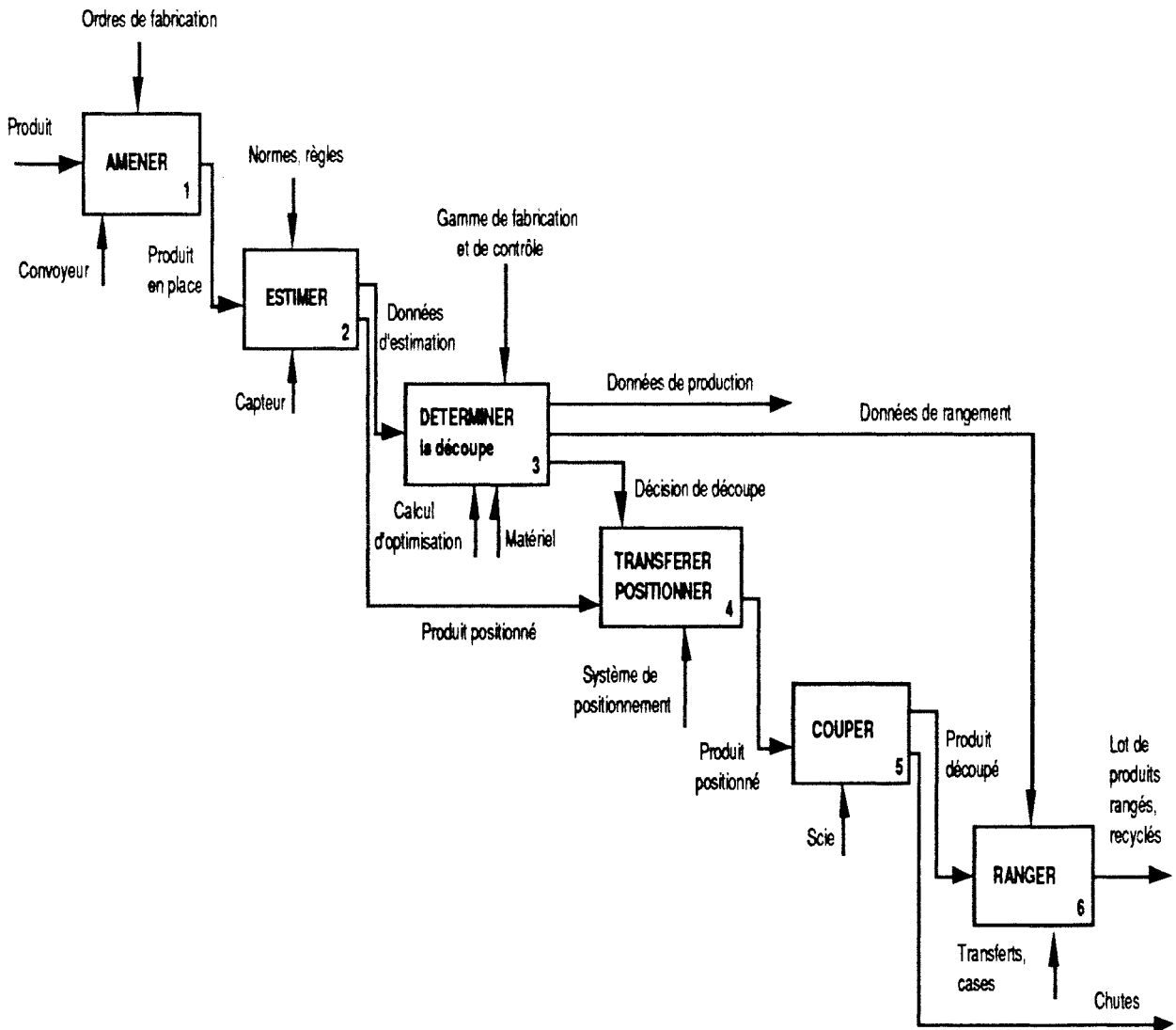
Figure 1.9. SADT de la fonction débit pour une ligne automatisée
