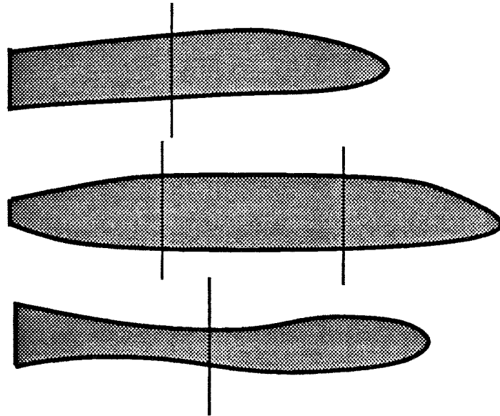
Figure 5.17. Possibilités de tronçonnage des dosses
