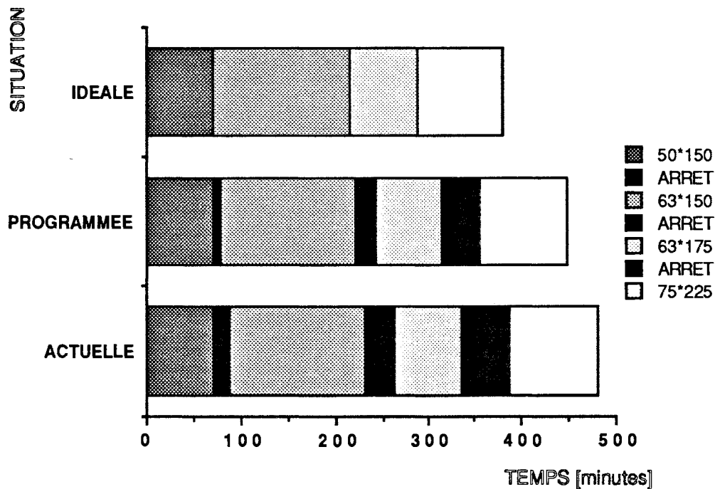
Figure 5.46. Temps de travail et d'arrêt du classeur pour plusieurs situations de fonctionnement
