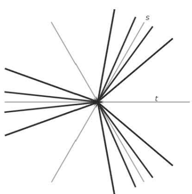
FIGURE 3 – Un autre exemple de décomposition vérifiant (H1)-(H7).
