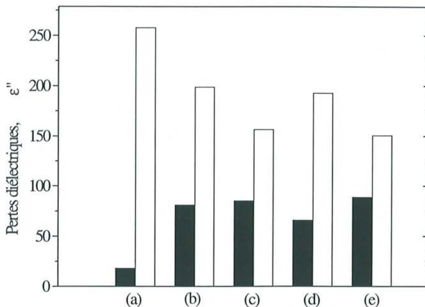
Figure III-13 : Comparaison des pertes diélectriques, \epsilon'' de la (■) solution basique initiale et (□) du système gel de silice - solution. Solution (a) NH 3 , (b) MeNH 2 , (c) EtNH 2 , (d) iBuNH 2 , (e) Et 3 N 10 -2 mol l -1 . Fréquence 10 MHz.
