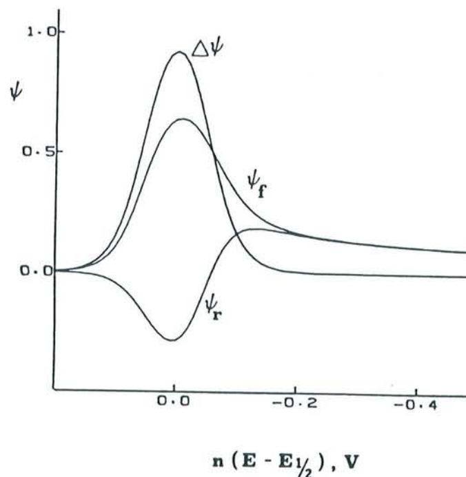
Figure II-16 : Voltampérogramme résultant d'une impulsion « ondes carrées ». \psi_f , \psi_r et \Delta\psi représentent respectivement, le courant aller, le courant retour et le rapport entre les deux courants \psi_f et \psi_r pour un couple Oxydant-reducteur, E_p = 50 \text{ mV} et E_s = 10 \text{ mV}
