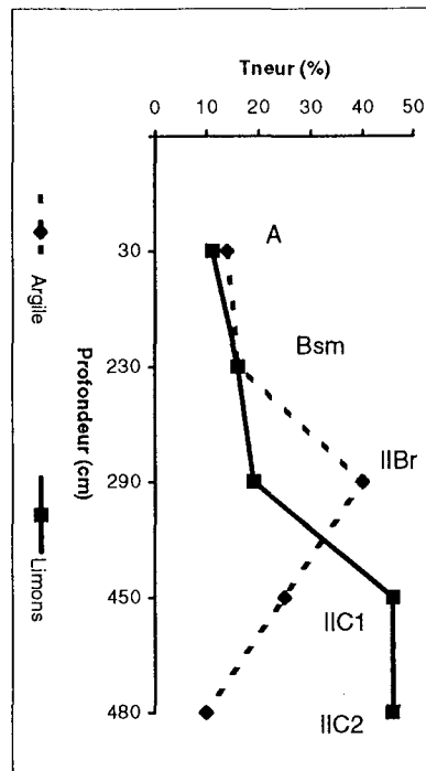
Analyses granulométriques
