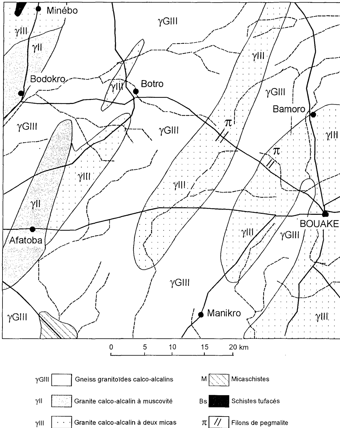
Figure I - 4 : Géologie de la région Centre (d'après Tagini 1969 )
