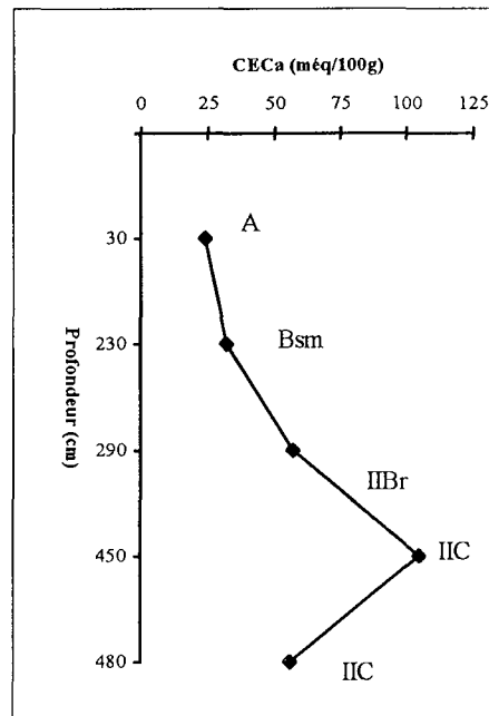
Capacité d'échange cationique de la fraction argileuse.
