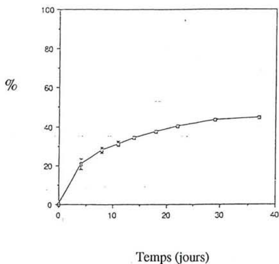
Figure 2.5. Minéralisation du naphthalène (%) présent à concentration de saturation dans des billes de silice microporeuses (d'après Ramaswami et Luthy, 1994)
