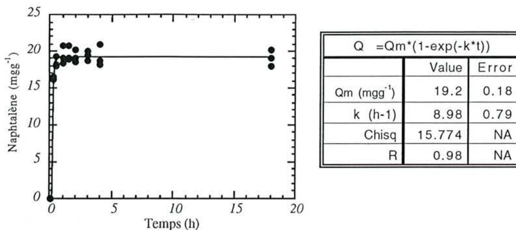
Figure 4.3. Cinétique de sorption du naphthalène sur 0,5gL -1 d'argile organique B34 . Modélisation du premier ordre - Ci=13,4mgL -1 - Agitation à 500rpm à 30°C
