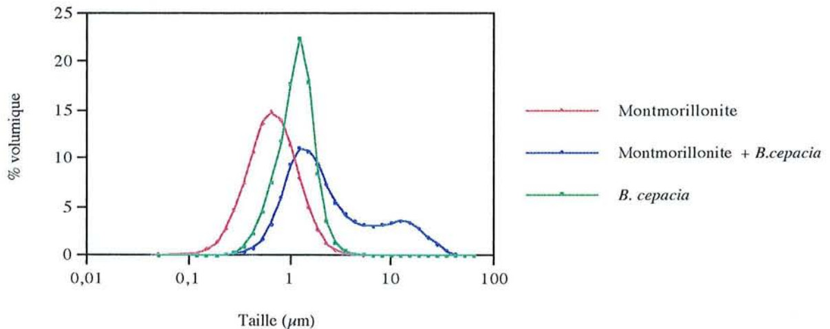
Figure 6.1. Taille des particules de montmorillonite, de montmorillonite avec Burkholderia cepacia et des bactéries mesurée en diffraction laser
