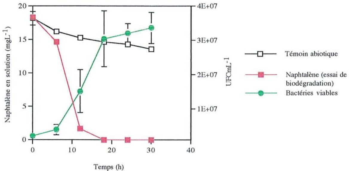
Figure 5.4. Evolution de la concentration en naphthalène dissous et de la concentration de Burkholderia cepacia (UFCmL -1 ) en fonction du temps
