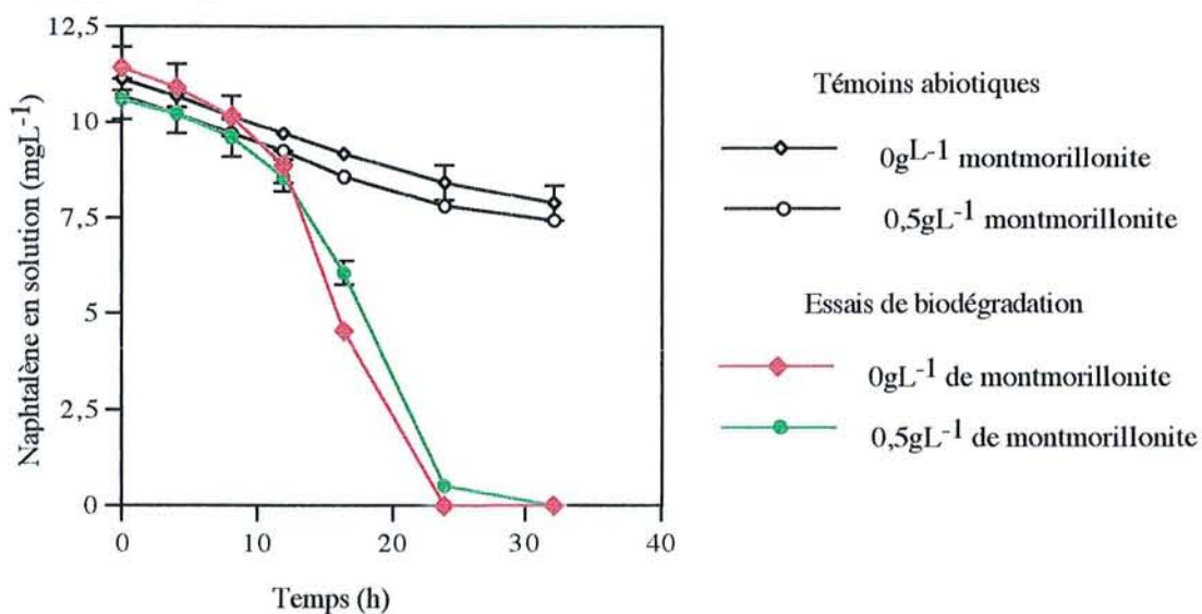
Figure 5.5. Evolution de la concentration en naphthalène avec 0\text{gL}^{-1} et 0,5\text{gL}^{-1} de montmorillonite sous agitation (500rpm) à 30°C pour les témoins abiotiques et en présence de 10^7\text{UFCmL}^{-1} ( n=2 )
