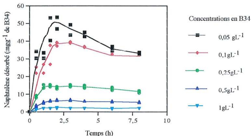
Figure 4.4. Cinétiques de désorption du naphthalène. Concentrations initiales en B34 comprises entre 0,05 et 1\text{gL}^{-1} - Agitation à 500\text{rpm} à 30^{\circ}\text{C} (Valeurs brutes en annexe 9)
