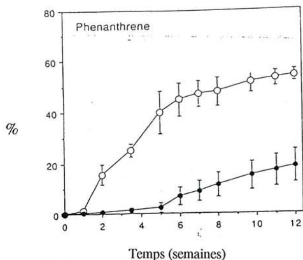
Figure 2.2. Comparaison du pourcentage de phénanthrène minéralisé dans de l'eau (●) et dans un système composé de sol et d'eau (○) (1:8g/mL). Chaque système a reçu le même inoculum capable de dégrader le phénanthrène (d'après Laha et Luthy, 1991)
