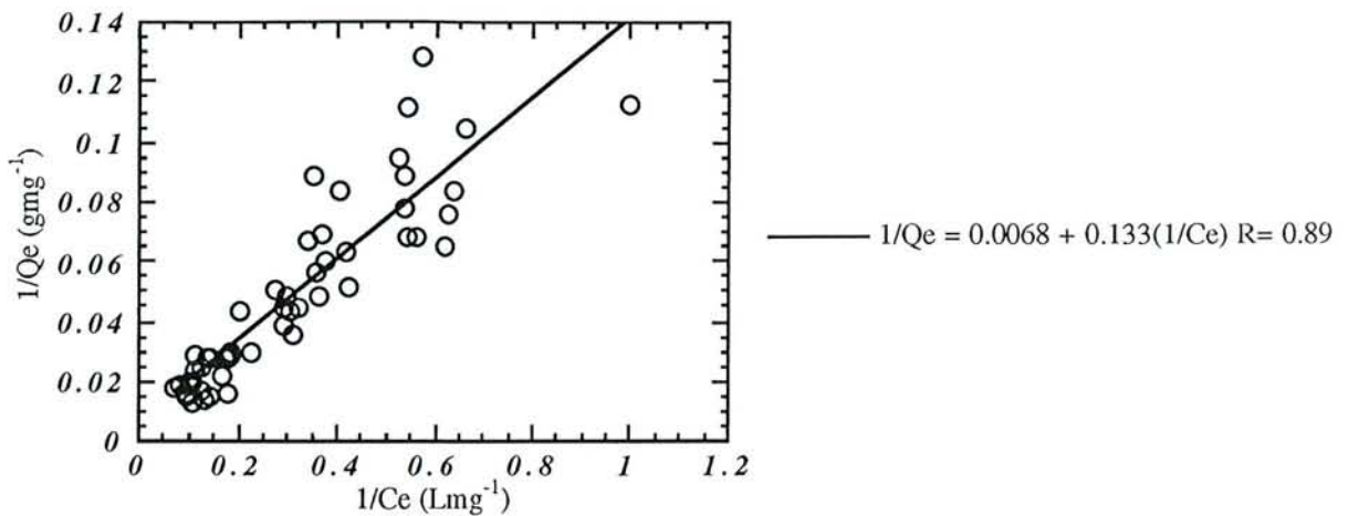
Figure 4.7. Isotherme de sorption du naphthalène sur l'argile organique B34 - Ajustement au modèle de Langmuir (tracé en double inverse) - Agitation à 500rpm à 30°C - Mesures à l'équilibre à t=12h et t=16h
