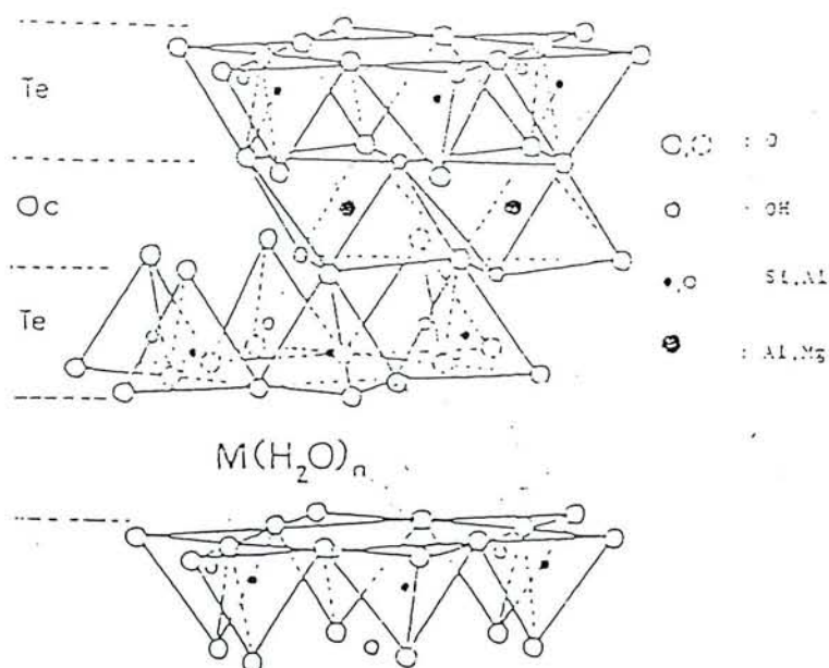
Figure 3.1. Représentation schématique d'un feuillet de montmorillonite constitué de 2 couches tétraédriques et d'une couche octaédrique (d'après Bruant, 1986)
