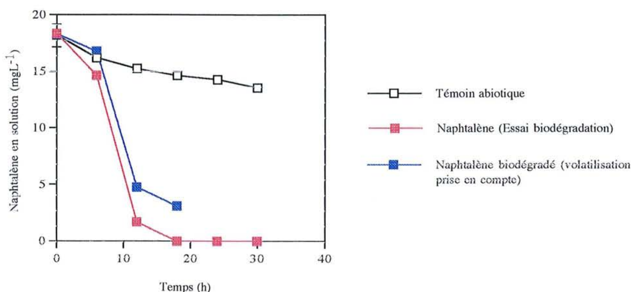
Figure 5.3. Evolution de la concentration en naphthalène en fonction du temps en présence de Burkholderia cepacia sous agitation magnétique (500rpm) à 30^\circ\text{C} : Témoin de volatilisation, valeurs brutes et valeurs corrigées de la volatilisation
