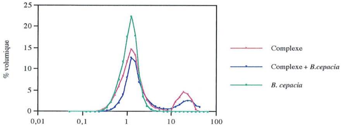
Figure 6. Granulométrie des particules de complexe montmorillonite/polyacrylamide, de Burkholderia cepacia et du mélange
