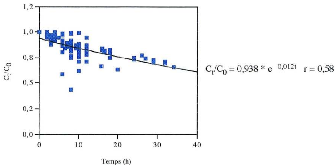
Figure 4.1. Evolution du rapport de la concentration en naphthalène au temps t=0 et de la concentration au temps t dans un milieu stérile contenu dans un flacon en Téflon 63 essais - Température de 30°C et agitation à 500rpm par barreaux magnétiques
