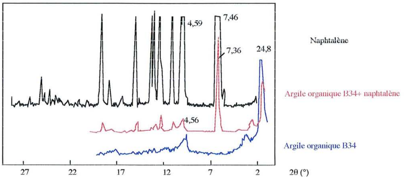
Figure 4.9. Spectre de diffraction X de l'argile organique B34, du naphthalène et de l'argile organique B34 gonflée par la présence de naphthalène
