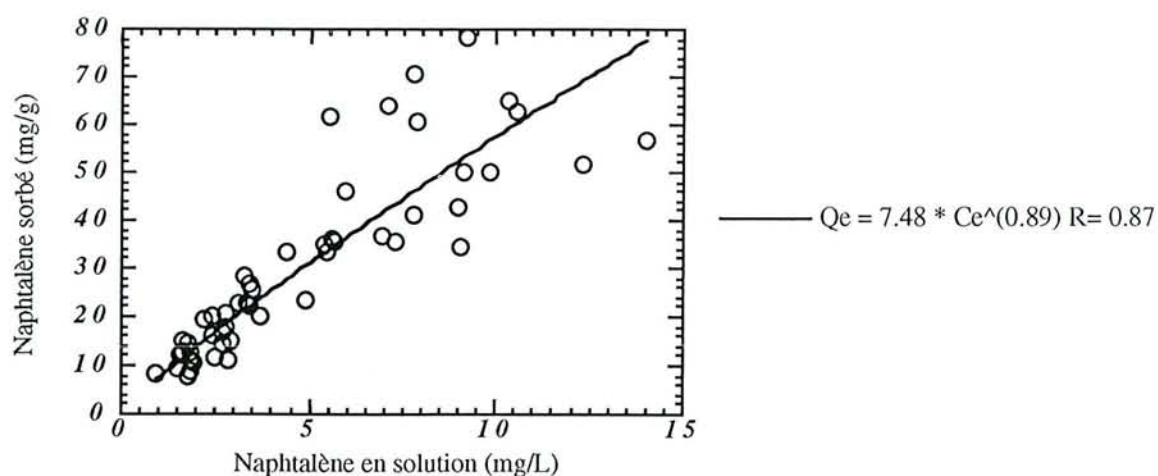
Figure 4.6. Isotherme de sorption du naphthalène sur l'argile organique B34 - Ajustement au modèle de Freundlich - Agitation à 500rpm à 30°C - Mesures à l'équilibre à t=12\text{h} et t=16\text{h}
