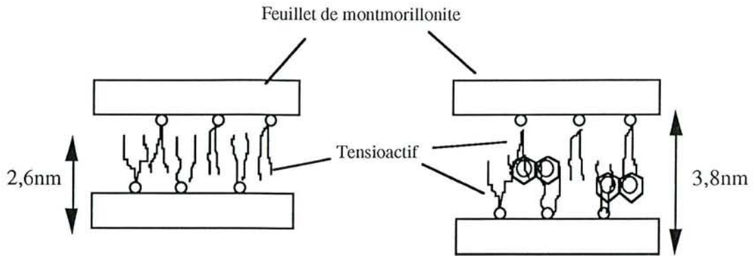
Figure 4.10. Agencement des molécules de tensioactif sur les feuillets de montmorillonite et augmentation de l'espace interfoliaire en présence de naphthalène
