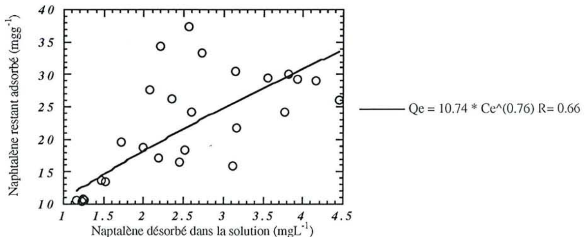
Figure 4.8. Isotherme de désorption du naphthalène à partir de l'argile organique B34 - Ajustement au modèle de Freundlich - Agitation à 500rpm à 30°C
