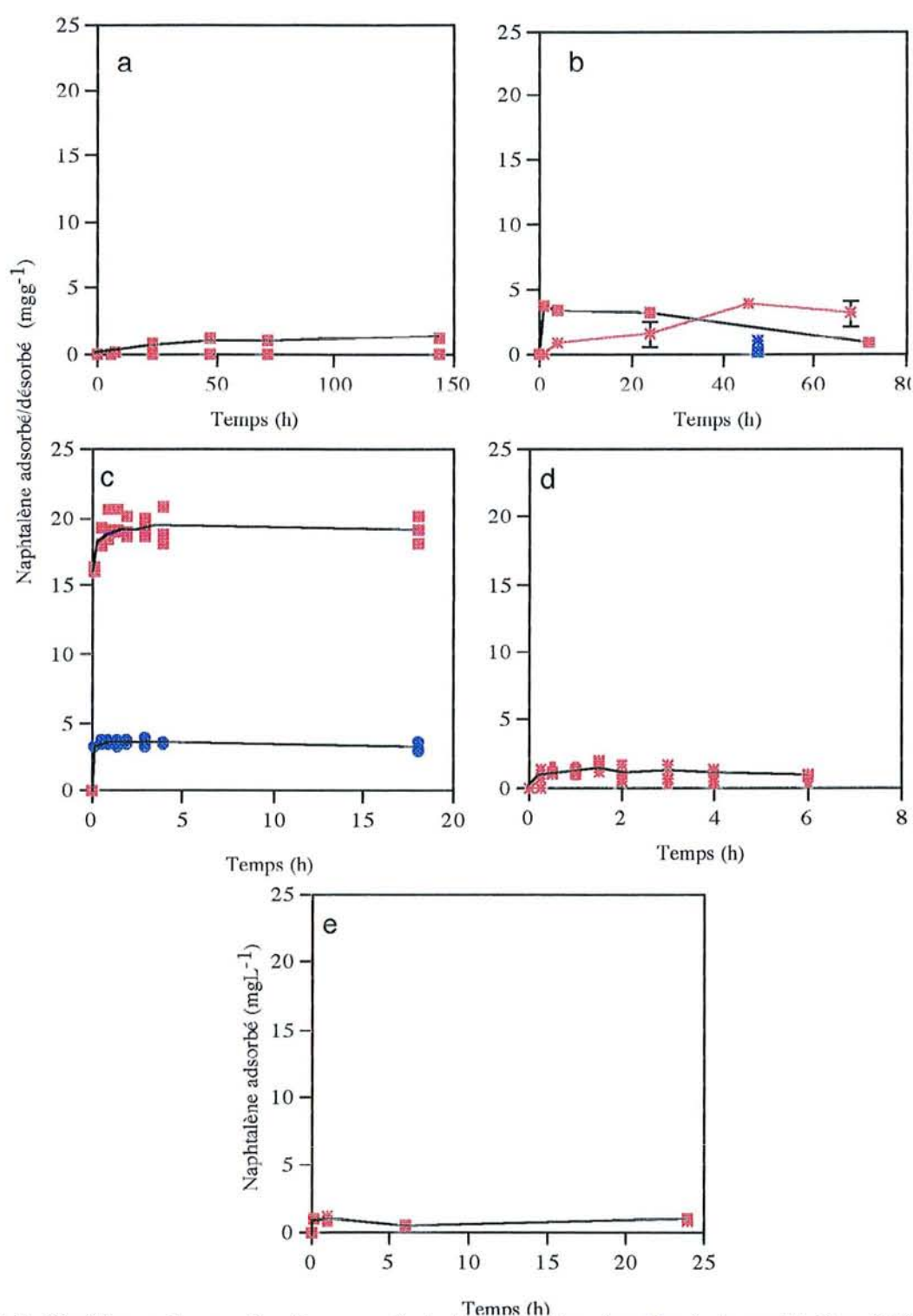
Figure 4.2. Cinétiques de sorption (en rouge) et de désorption (en bleu) du naphthalène à 30°C. a) Adsorption avec 0,5gL -1 de montmorillonite de sodium (triplicat sur trois concentrations initiales : 16,7; 11,6; et 5,9mgL -1 ); b) Adsorption (.....*.....) et désorption (■) avec 0,25gL -1 de complexe 44000 (duplicats sur Ci = 27,5mgL -1 ), Adsorption (—■—) et désorption (—*—) avec 0,25gL -1 de complexe 2,6.10 6 (duplicat sur Ci = 24,5mgL -1 ); c) Adsorption (—■—) et désorption (●) avec 0,5gL -1 de B34 (Tripliquat Ci = 13,4mgL -1 ); d) Adsorption (—■—) avec 1gL -1 de sédiment et (.....*.....) sédiment additionné de 40mgL -1 HgCl 2 (Duplicat Ci = 28,9mg/L); e) Adsorption sur la biomasse bactérienne Burkholderia cepacia (3.10 9 bactmL -1 ) (4 essais Ci = 15mgL -1 de naphthalène) stérilisation par autoclavage (—■—) et par ajout de 40mgL -1 de HgCl 2 (—*—)
