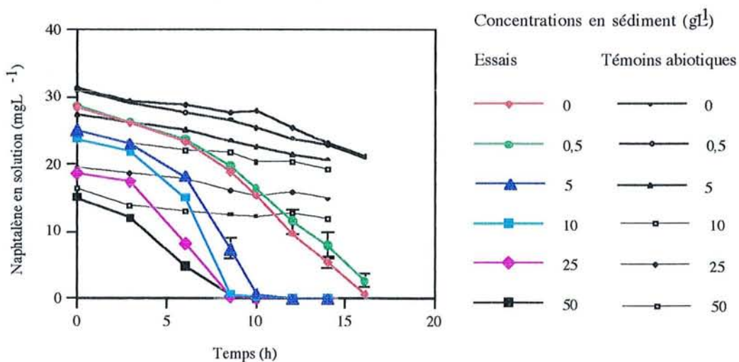
Figure 5.12. Evolution de la concentration de naphthalène en solution en présence de différentes concentrations de sédiment de rivière non stérile - Agitation à 500rpm à 30°C - Ajout de 10 6 UFCmL -1 de Burkholderia cepacia
