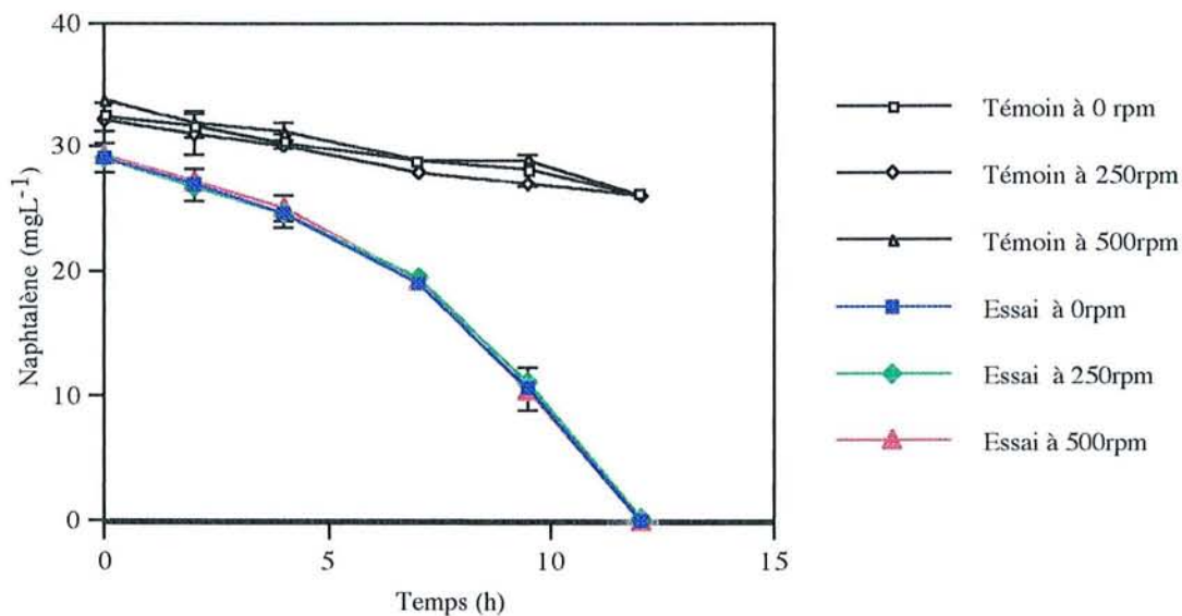
Figure 6.6. Biodégradation du naphthalène par Burkholderia cepacia dans une suspension de 0,5gL -1 de montmorillonite à une température de 30°C sous différentes vitesses d'agitation.
