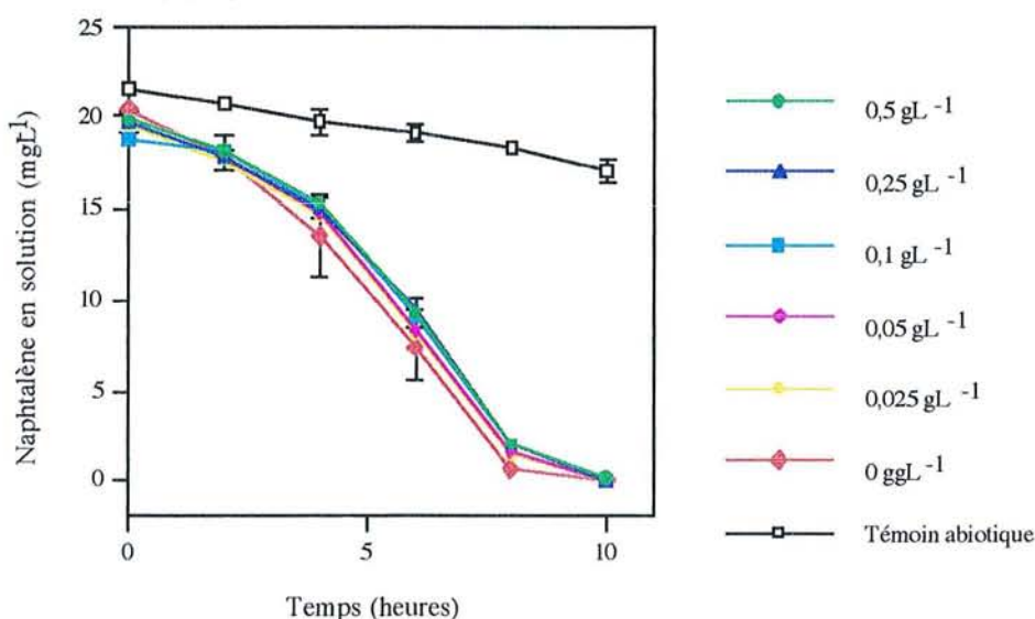
Figure 5.7. Evolution de la concentration en naphthalène en présence de différentes concentrations en complexe montmorillonite/polyacrylamide pour une concentration initiale en Burkholderia cepacia de 9,4 10 6 UFCmL -1 (Agitation à 500rpm à une température de 30°C) - Témoin abiotique pour 0gL -1 de complexe
