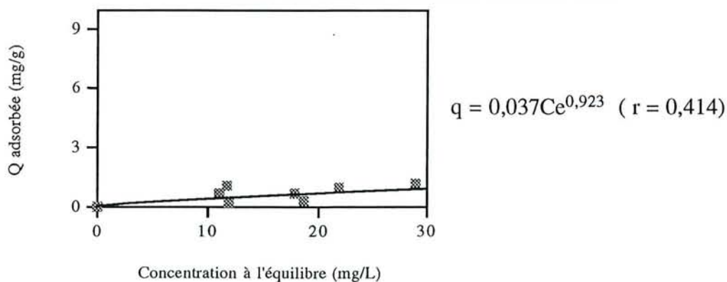
Figure 3. Isotherme d'adsorption du naphthalène sur le complexe - Ajustement à un modèle de Freundlich
