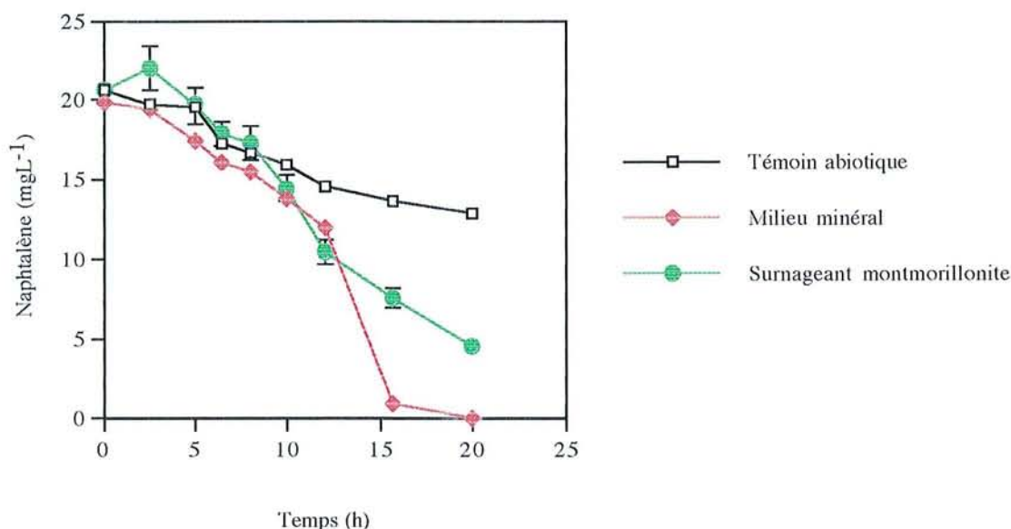
Figure 6.8. Evolution de la concentration en naphthalène dans un milieu minéral et dans un surnageant de montmorillonite en présence de 2,5 \cdot 10^7 \text{ UFC mL}^{-1} ( Burkholderia cepacia ) à 30°C sous agitation magnétique (500rpm) (n=3)
