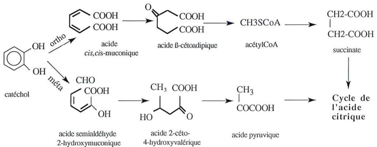
Figure 5.2. Clivages ortho ou méta du catéchol (d'après Barnsley, 1976 et Gottschalk, 1986)
