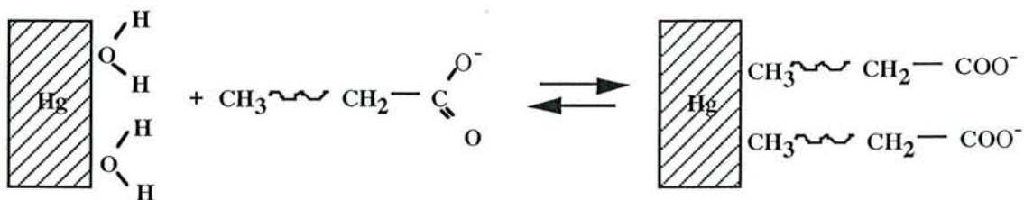
Figure 2.10. Interactions hydrophobes entre une chaîne d'hydrocarbure et une surface de mercure (d'après Ulrich et al. , 1988)
