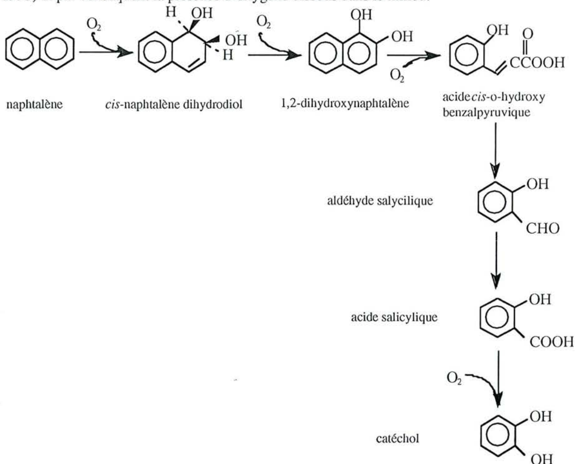
Figure 5.1. Voie d'oxydation du naphthalène en catéchol par des bactéries en milieu aérobie (d'après Kiyohara and Nagao, 1978)
