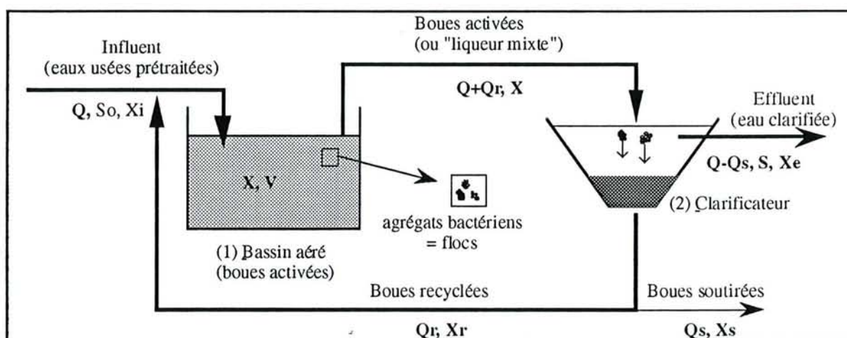
Figure I-1 : Schéma simplifié du traitement des eaux usées par le procédé à "boues activées". Q , Q_r , Q_s = débit respectivement de l'influent, des boues recyclées, des boues soutirées. X , X_i , X_s , X_e , X_r = concentration en matières sèches en suspension respectivement des boues activées, de l'influent, des boues soutirées, de l'effluent et des boues recyclées. S_o = concentration initiale en matière organique. S = concentration résiduelle en matière organique.
