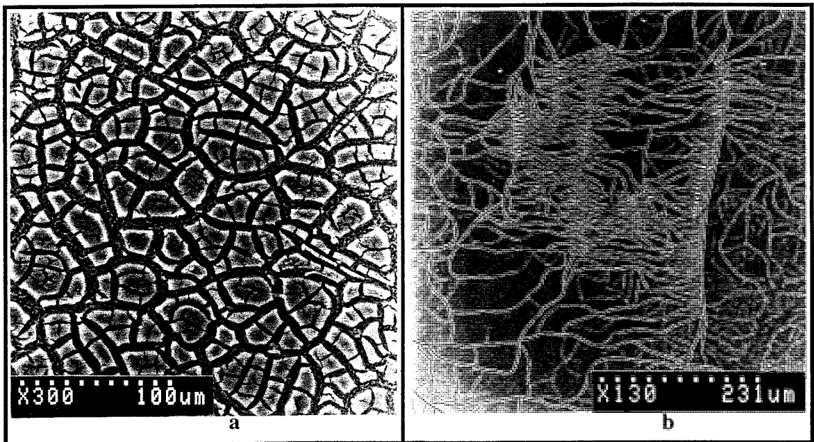
Figure C.7: micrographies montrant la morphologie d'une couche obtenue par anodisation d'un substrat Si de type p(111) et de résistivité \rho \approx 100 \Omega \cdot \text{cm} (fig.C.7.a) et d'une couche préparée par la même technique à partir d'un substrat de type n(100) avec \rho \approx 10^{-2} \Omega \cdot \text{cm} (fig.C.7.b). Les conditions de préparation sont identiques dans les deux cas: électrolyte composé de 50% HF/H 2 O + 50% C 2 H 5 OH, J = 10 \text{ mA/cm}^2 et durée de l'anodisation \Delta t \approx 20 \text{ min}
