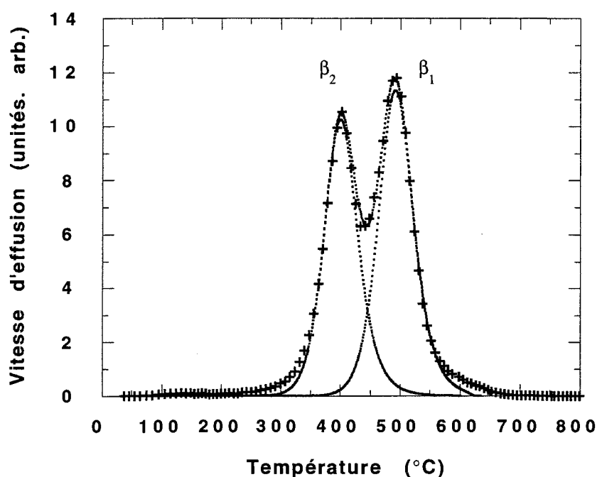
Figure C.12: spectre d'effusion de H_2 d'un échantillon de silicium poreux préparé dans les conditions suivantes: substrat Si de type p(111) abrasé, solution NaNO_2/HF (30 g/l), durée du trempage t = 12 min, \beta = 15 K/min. Le symbole + représente les points expérimentaux et les pointillés la simulation des pics \beta_2 et \beta_1
