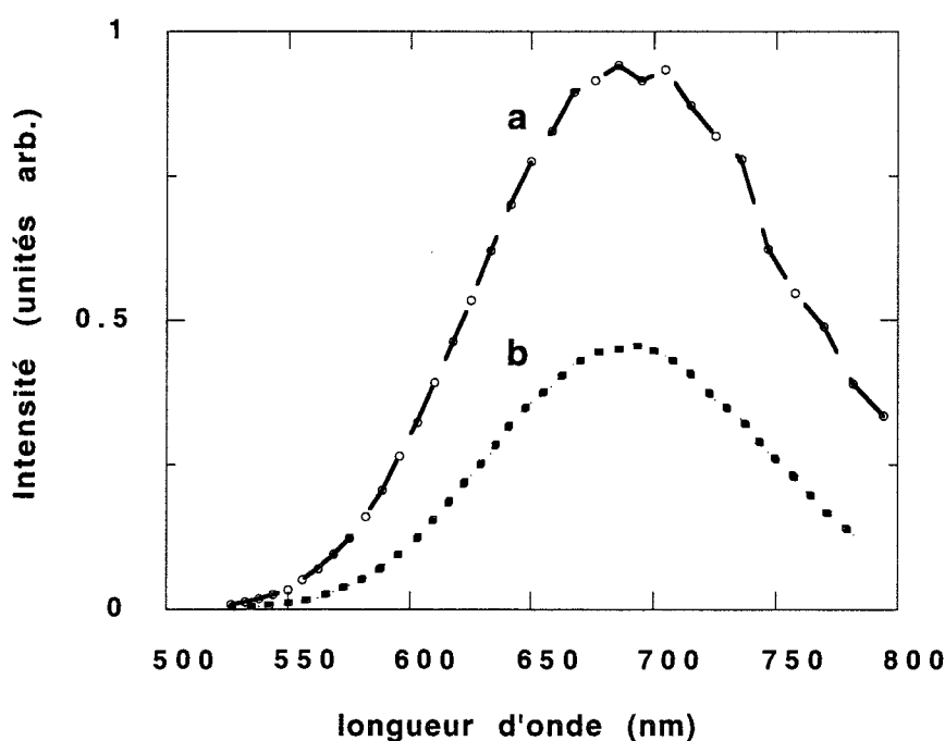
Figure C.10: comparaison entre les spectres de photoluminescence de deux échantillons poreux préparés par anodisation (a) dans un mélange HF/H 2 O/C 2 H 5 OH et par trempage chimique (b) dans NaNO 2 /HF
