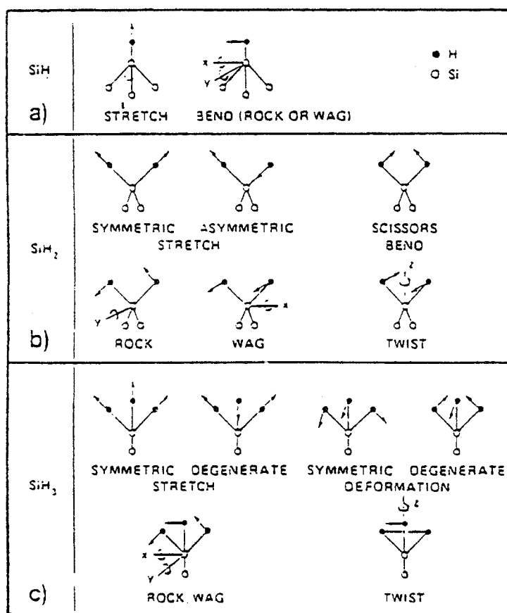
Figure B.38: déplacements des atomes H correspondant aux différents modes de vibration dans les groupes SiH (a), SiH 2 (b) et SiH 3
