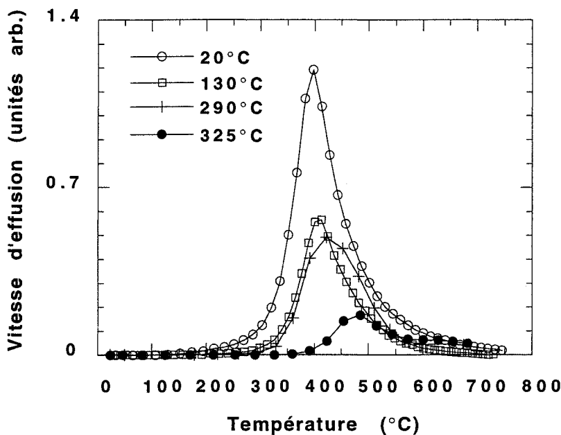
Figure B.26: influence de la température de substrat sur le spectre d'effusion de \text{D}_2 d'une couche a-Si:D. Paramètres de dépôt: e = 2000 \text{ \AA} , P_{\text{ECR}} = 200 \text{ W} , P_{\text{D}_2} = 4 \times 10^{-5} \text{ Torr}
