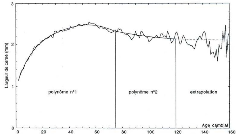
Figure 29 : Arbres de futaie. Accroissement moyen en fonction de l'âge exprimé en largeur de cerne annuelle et ajustements polynomiaux calculés entre 2 et 75 ans et entre 75 et 120 ans.
