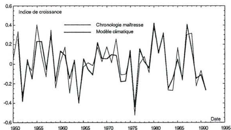
Figure 133 : Modèle FUT4. Reconstruction climatique de la chronologie de futaie avec prise en compte de l'autocorrélation sur un an.
