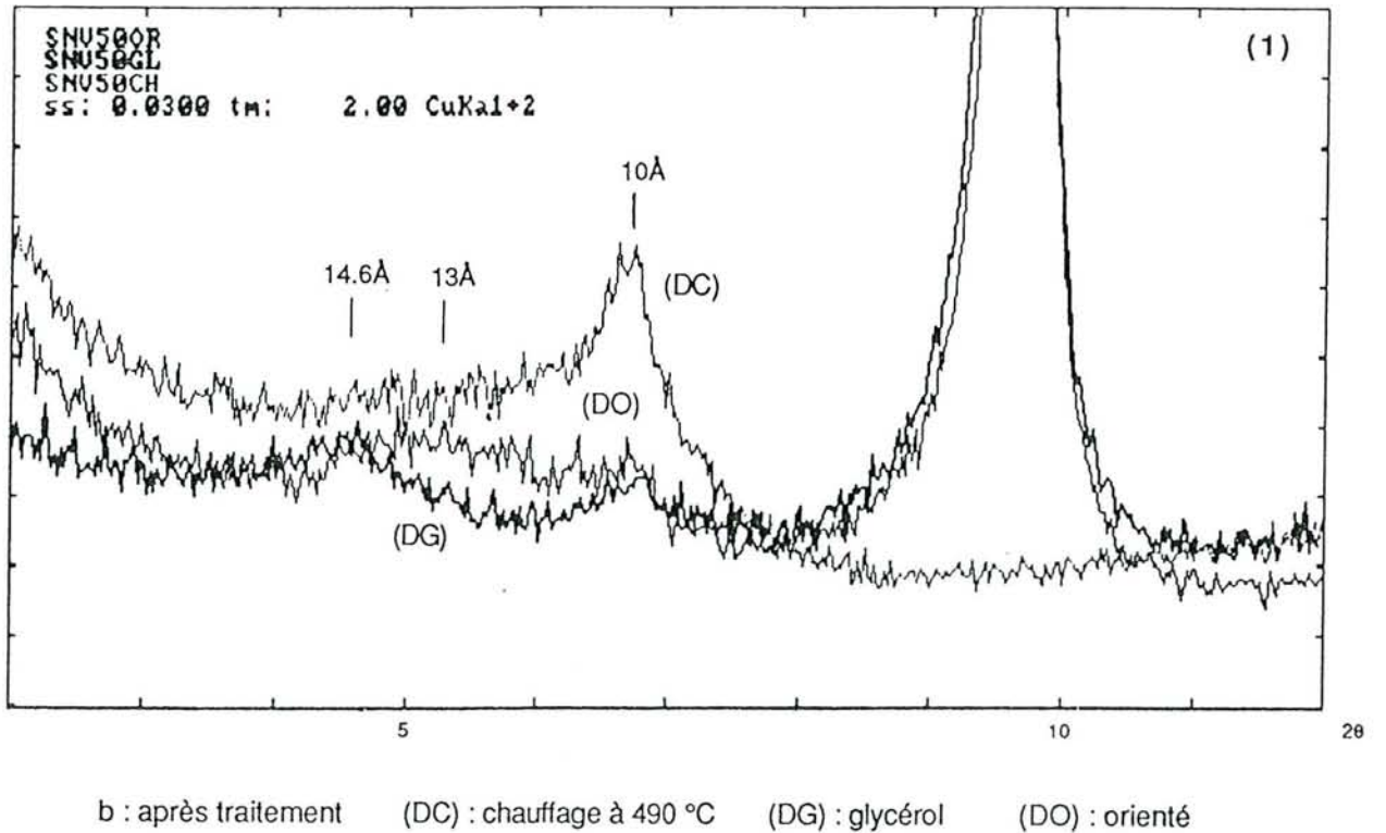
Figure VII-4 Diffractogramme RX des minéraux argileux
