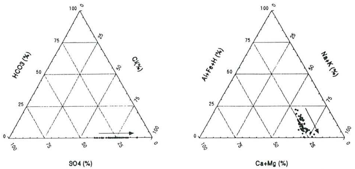
Figure VI-9 Composition chimique des eaux de surface du barrage de Djalakoun en fonction de leur niveau de concentration
