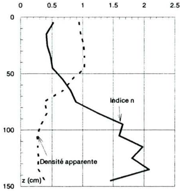
Figure VIII-4 Répartition de l'indice de maturation n et de la densité apparente sèche dans un sol sulfaté acide (tanne herbacé STH) du bas-fond de Djiguinoum
