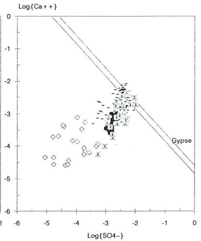
Figure VII-7 Diagramme d'équilibre du gypse
