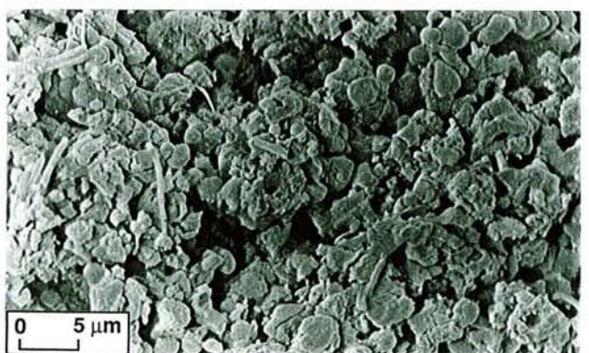
Rozénite
