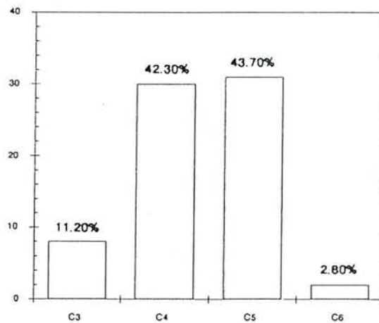
Figure VI-4 Répartition des échantillons d'eau de surface du barrage de Djilakoun dans les classes de conductivité électrique du diagramme USSLS: C3 (0.75 dS/m < CE < 2.25 dS/m), C4 (2.25 dS/m < CE < 5 dS/m), C5 (5 dS/m < CE < 20 dS/m), C6 (CE > 20 dS/m)
