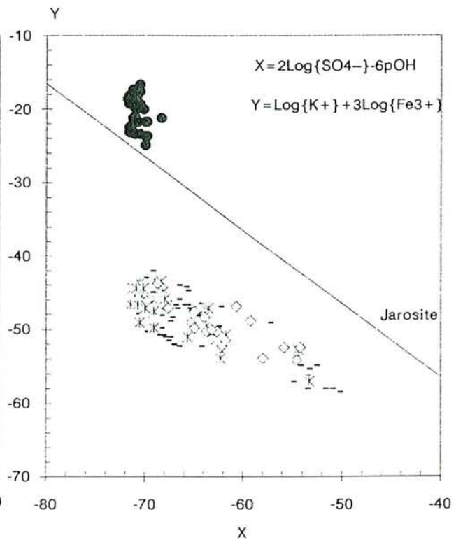
Figure VII-9 Diagramme d'équilibre de la jarosite
