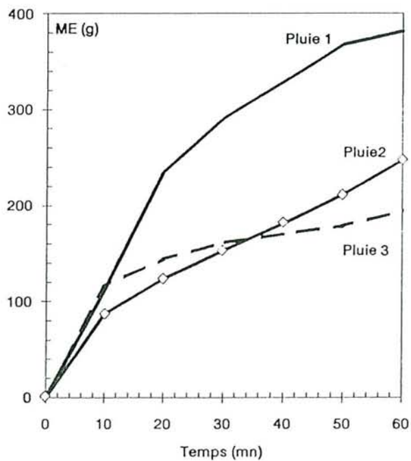
Figure VIII-12 Quantité de sel exporté de la parcelle de ruissellement au cours de la simulation de pluies sur un sol sulfaté acide (tanne vif STV) du bas-fond de Djiguinoum
