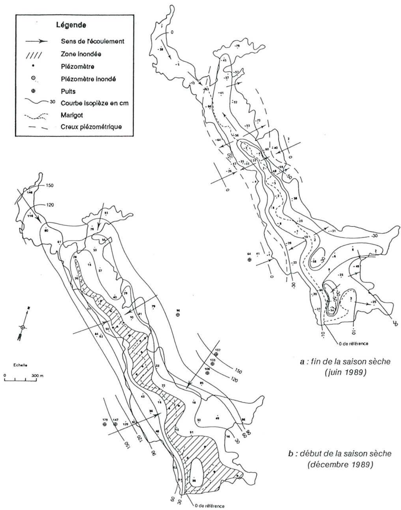
Figure V-9 Distribution spatiale des isopiètes de la nappe du bassin versant de Djiginoum à deux périodes de l'année
