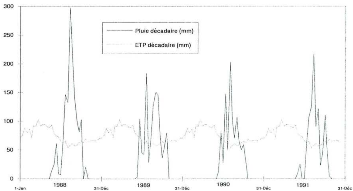
Figure II-8 Bilan climatique sur le bassin versant de Djiguinoum durant la période 1988-1991 (d'après ALBERGEL et al., 1991d) ( — Pluviométrie ---- Evapotranspiration potentielle Penman)
