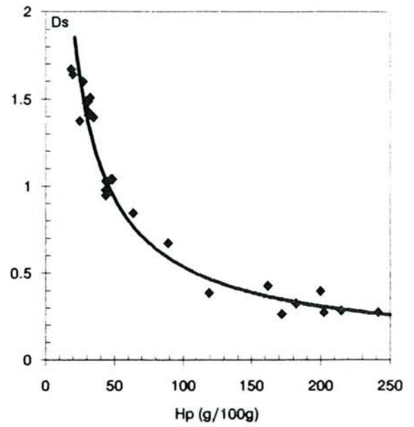
Figure VIII-5 Relation densité apparente sèche ( D_s ) - humidité pondérale ( H_p ) de deux sols sulfatés acides (tanne vif STV et tanne herbacé STH) du bas-fond de Djiguinoum
