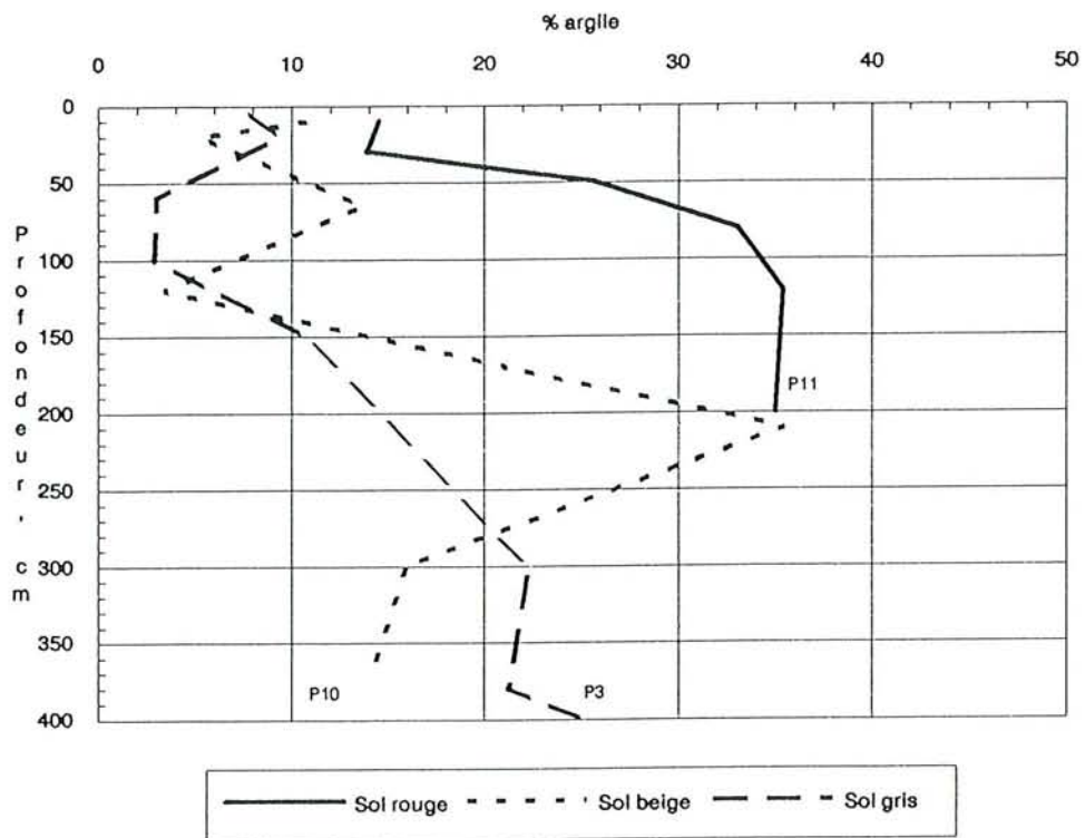
Figure III-6 Répartition de l'argile dans quelques sols de la toposéquence de Fégréom (voir la figure III-2 pour la localisation des sols)
