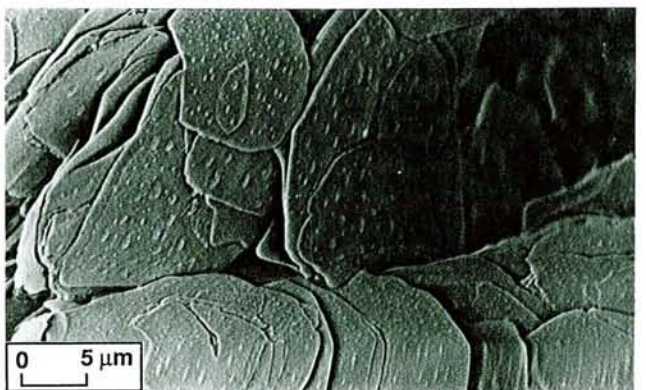
Tamarugite
