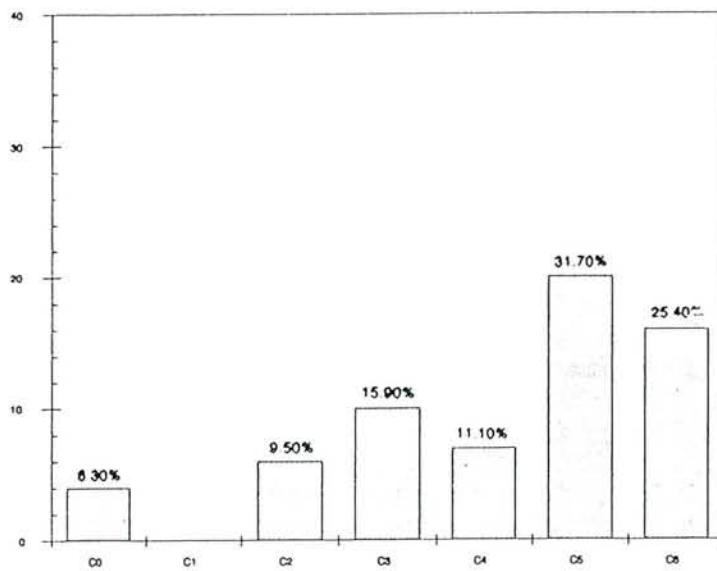
Figure VI-23 Répartition des échantillons d'eau de nappe au début de la saison sèche dans les classes de conductivité électrique du diagramme USSLS
