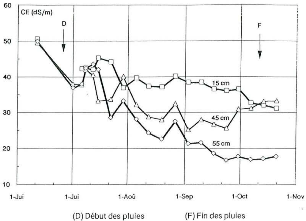
Figure VIII-7 Evolution temporelle de la salinité d'un sol sulfaté acide (tanne herbacé STH) du bas-fond de Djiguinoum au cours de la saison des pluies 1990
