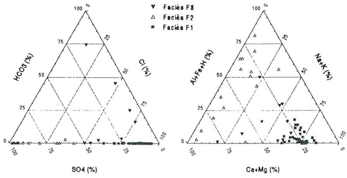
Figure VI-25 Composition anionique et cationique des eaux de nappe selon leur faciès chimique au début de la saison sèche
