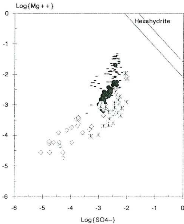
Figure VII-8 Diagramme d'équilibre de l'hexahydrate
