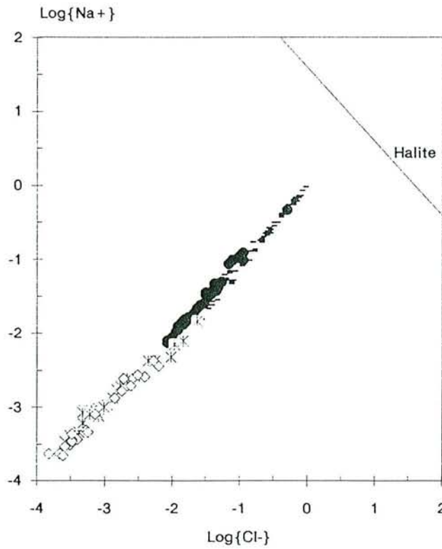
Figure VII-6 Diagramme d'équilibre de la halite
