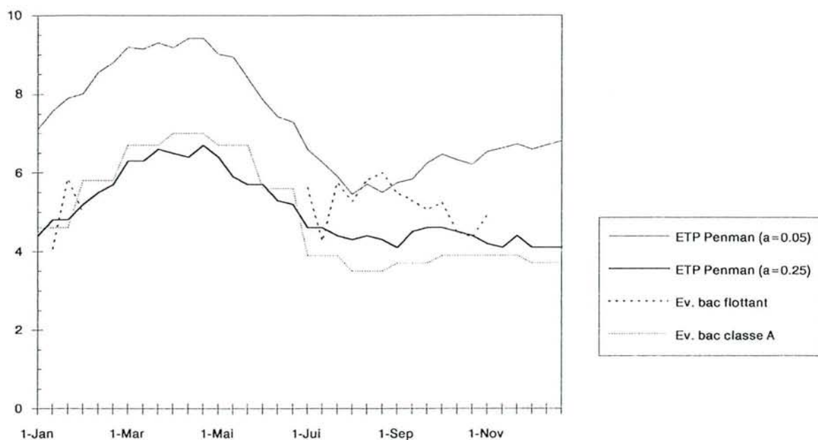
Figure II-7 ETP Penman et évaporation en bac journalières (mm /j) à l'échelle décadaire (d'après DACOSTA, 1989 ; MBAYE, 1991 ; ALBERGEL et al., 1991d)
