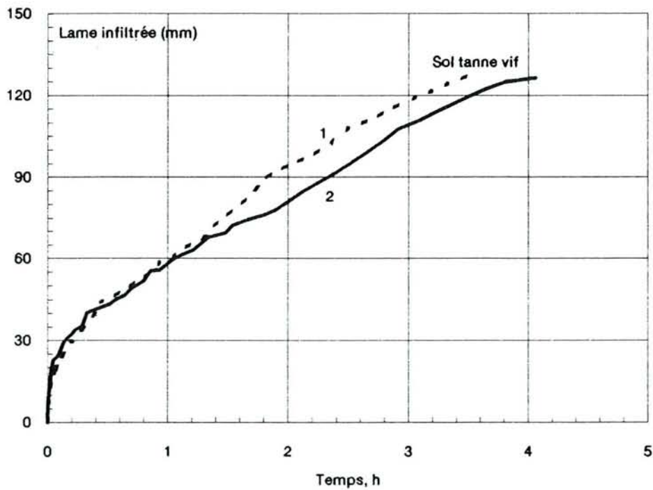
Figure VIII-6 Evolution temporelle de la lame infiltrée sous charge constante dans un sol sulfaté acide (tanne vif STV) du bas-fond de Djiguinoum
