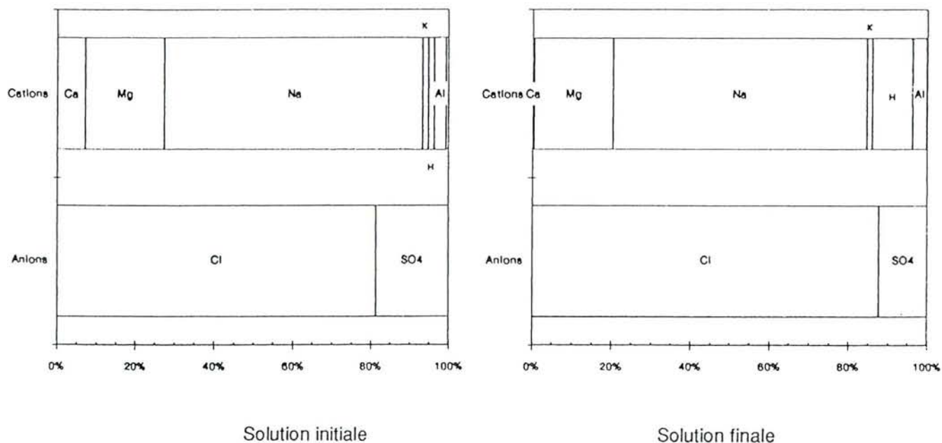
Figure VI-17 Faciès chimiques initial et final d'une eau de surface en évaporation contrôlée
