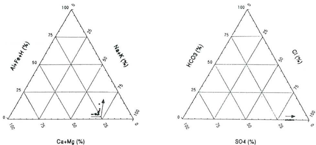
Figure VI-16 Evolution des compositions anionique et cationique d'une eau de surface en évaporation contrôlée
