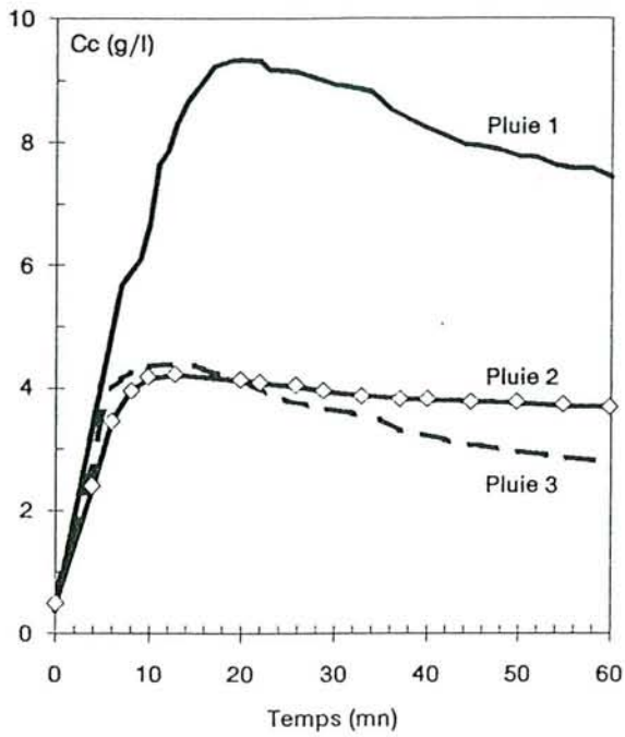
Figure VIII-10 Concentration des eaux de ruissellement au cours de la simulation de pluies sur un sol sulfaté acide (tanne vif STV) du bas-fond de Djiguinoum
