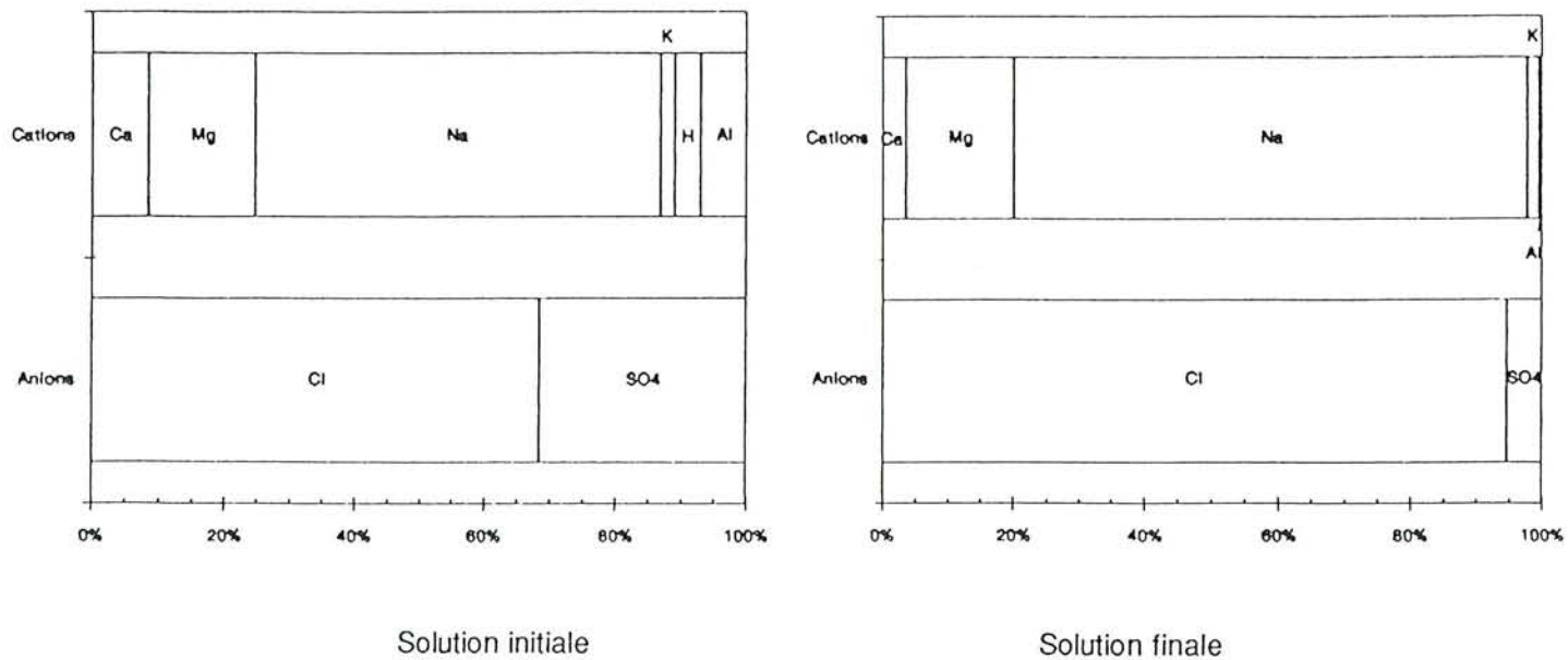
Figure VI-10 Faciès chimiques extrêmes des eaux de surface du barrage de Djalakoun
