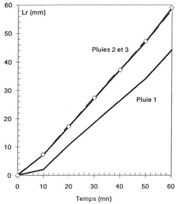
Figure VIII-11 Lame d'eau ruisselée au cours de la simulation de pluies sur un sol sulfaté acide (tanne vif STV) du bas-fond de Djiguinoum
