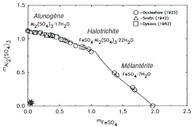
Figure VII-12 Diagramme d'équilibre dans le système FeSO 4 -Al 2 (SO 4 ) 3 -H 2 O à 25 °C (d'après PABALAN et PITZER, 1991)
