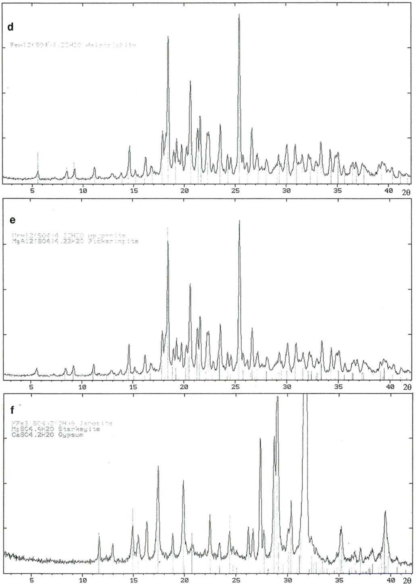
Figure VI-29 Diffractogrammes RX de l'halotrichite (d), de l'apjohnite-pickéringite (e) et de la jarosite-starkéyite-gypse (f)
