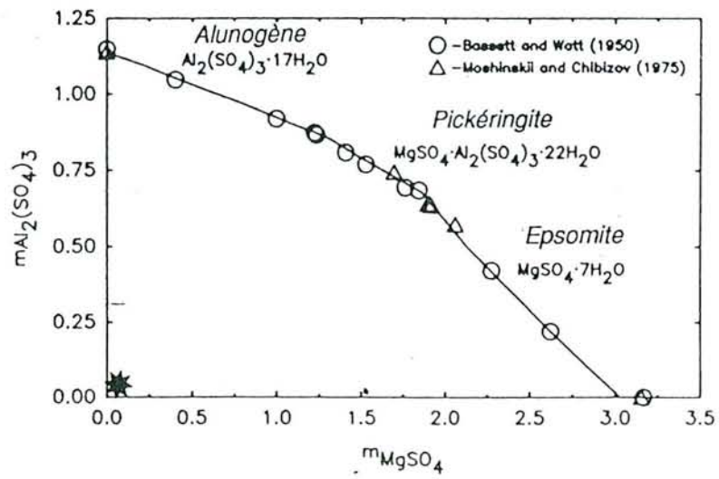
Figure VII-11 Diagramme d'équilibre dans le système \text{MgSO}_4\text{-Al}_2(\text{SO}_4)_3\text{-H}_2\text{O} à 25 °C (d'après PABALAN et PITZER, 1991)
