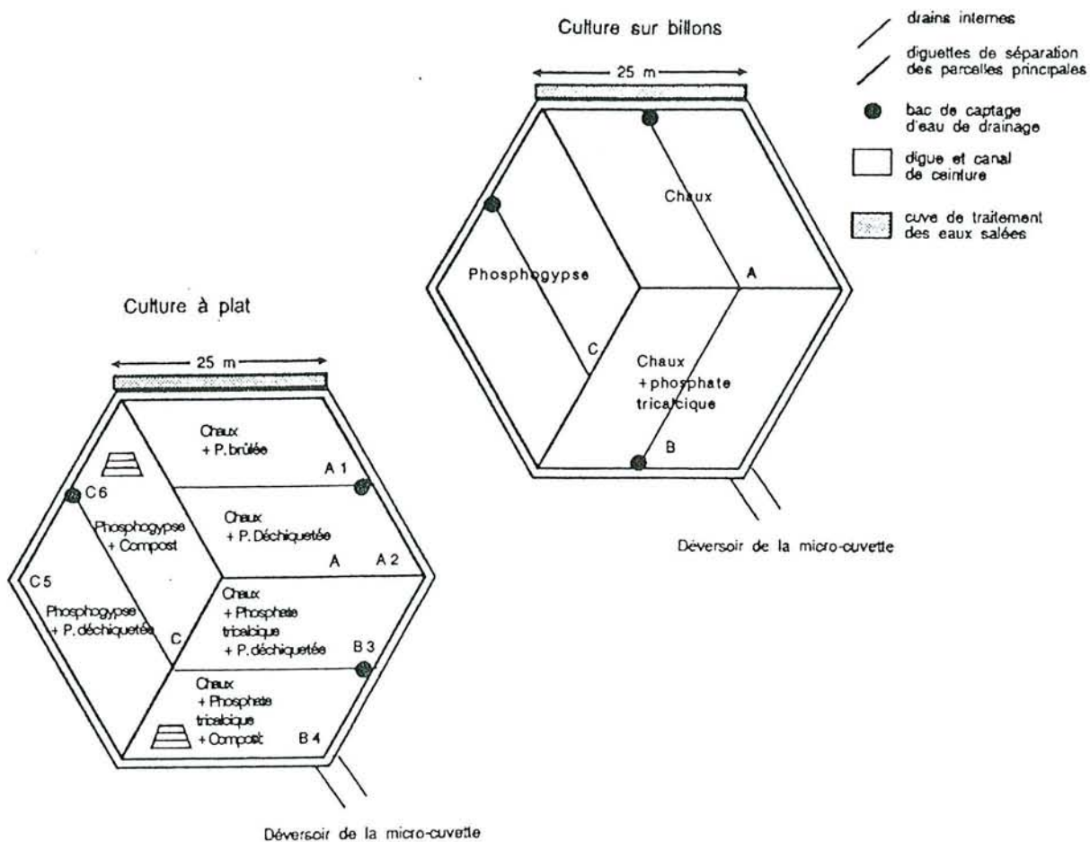
Figure IX-3 Essai agronomique sur un sol sulfaté acide du bas-fond de Djiguinour (d'après DOBOS et al., 1994)
