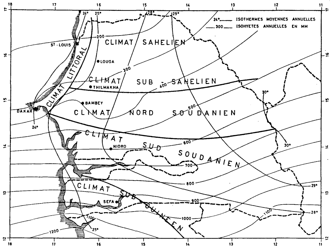
Figure 2 : Isohyètes correspondant à la période 1968-1987 pour Bambeý, Niouro et Séfa et 1972-1987 pour Thilmakha. Pluviométrie atteinte ou dépassée à la probabilité de 50 %. Isothermes annuelles et principaux climats d'après ADAMS et al (1965).
