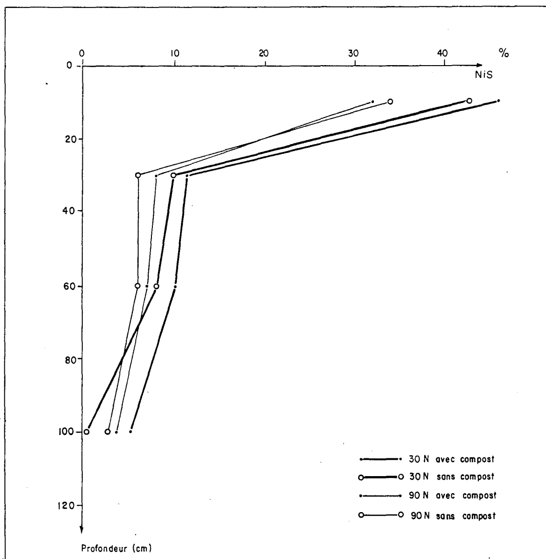
Figure 13 : Profil d'immobilisation de l'azote engrais dans le sol sous culture de mil. Dose urée 30 et 90 kg N ha -1 sans compost (A) et avec compost (B). Bambeu, essai au champ I.
