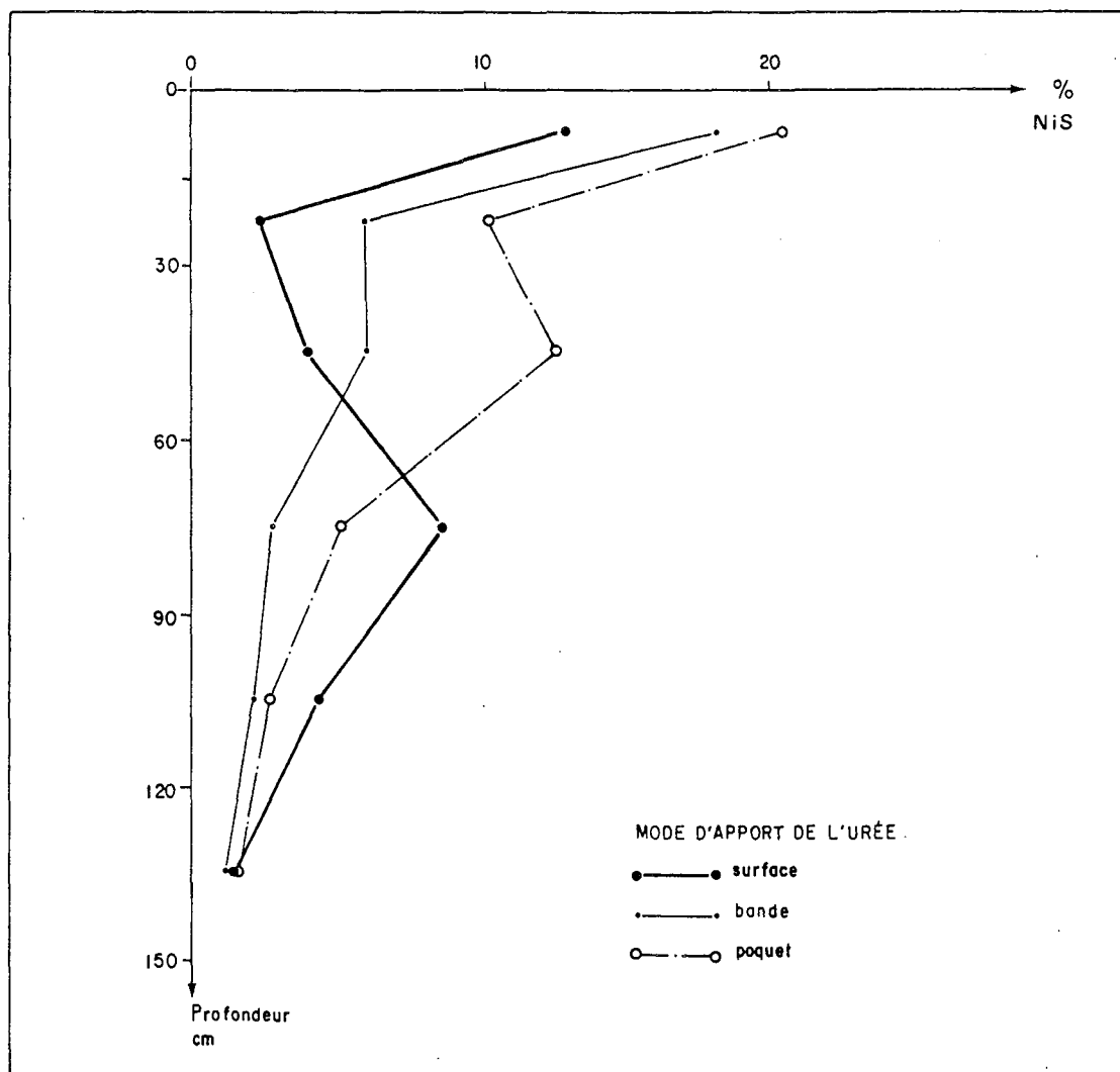
Figure 16 : Profil d'immobilisation de l'azote engrais dans le sol (NiS %) sous culture de maïs. Dose d'urée apportée 100 \text{ kg N ha}^{-1} . Séfa, essai au champ VI.
