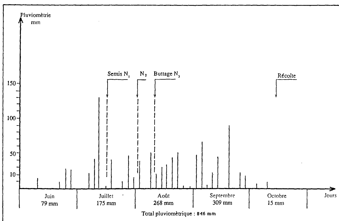
Figure 7 A : Pluviométrie à Séfa en 1985 et cycle végétatif du maïs. Pluie cumulée tous les trois jours. N 1 , N 2 et N 3 = apports urée marquée avec 15 N sur maïs. Essai au champ VII.
