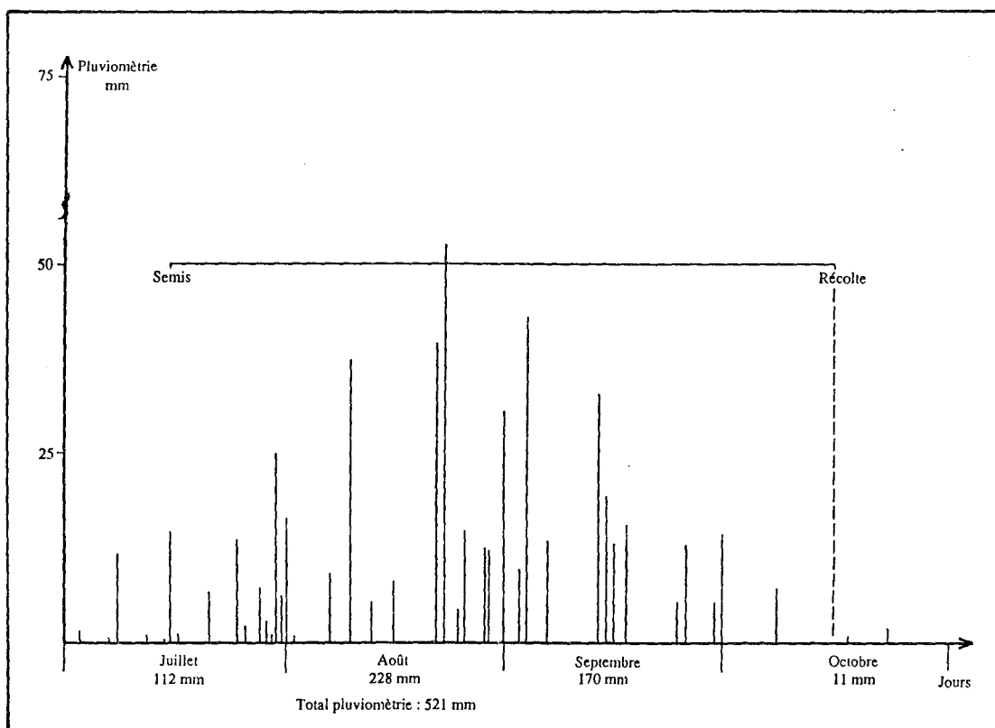
Figure 9 A : Pluviométrie de Bambeï en 1975 et cycle végétatif de l'arachide. Essai au champ XIII.
