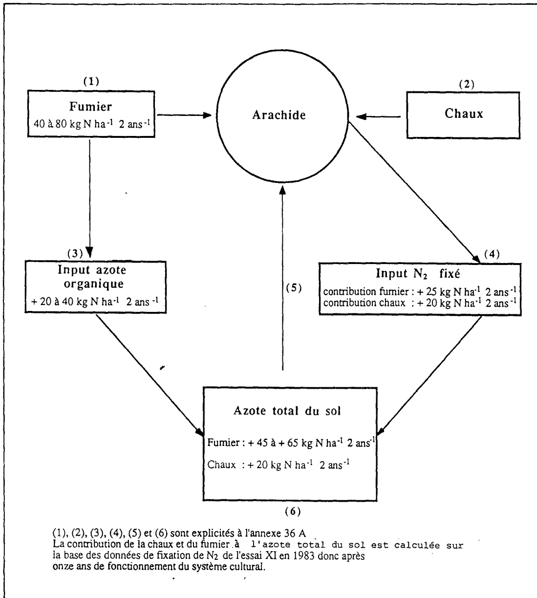
Figure 28 : Schéma d'interprétation des effets de la chaux et du fumier (respectivement 0,6 et 10 t ha -1 2 ans -1 ) sur la régénération de la fertilité azotée du sol. Thilwakha, essai au champ XI.
