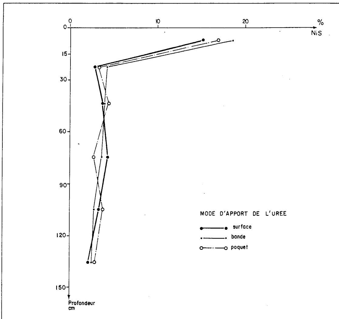
Figure 15 : Profil d'immobilisation de l'azote engrais dans le sol (NiS %) sous culture de maïs. Dose d'urée apportée 100 \text{ kg N ha}^{-1} . Séfa, essai au champ IV.
