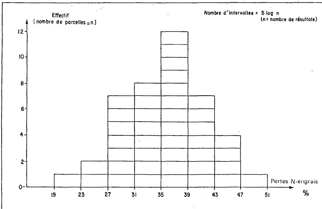
Figure 19 : Histogramme des pertes d'azote engrais hors du sol cultivé en maïs. Dose d'urée apportée 100 \text{ kg N ha}^{-1} . Niro, essai au champ IV.
