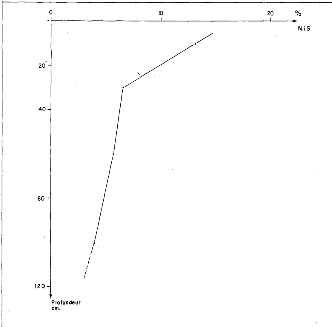
Figure 20 : Profil d'immobilisation de l'azote engrais dans le sol (NiS %) sous culture de maïs. Dose d'urée apportée 100 \text{ kg N ha}^{-1} . Nioro, essai au champ IV.
