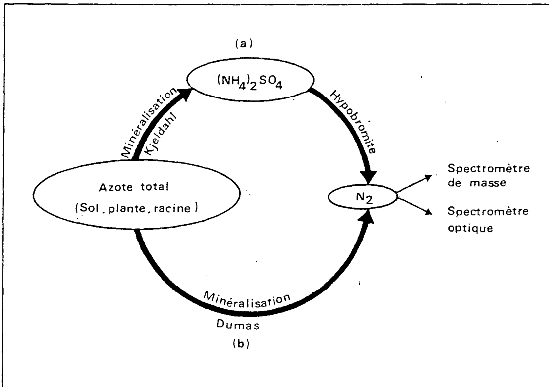
Figure 7 : Schéma montrant les deux méthodes de dosage de l'azote 15. D'après GUIRAUD (1984).
