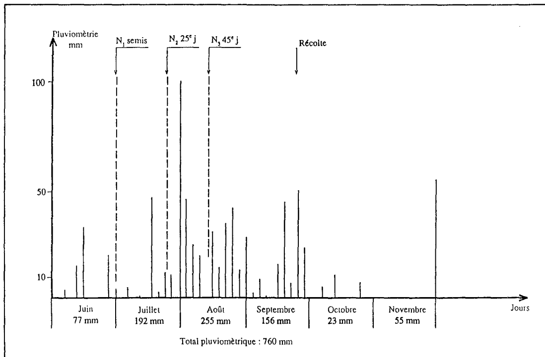
Figure 4 A : Pluviométrie à Niro en 1978 et cycle végétatif du maïs. Pluie cumulée tous les trois jours. N 2 et N 3 = apport urée marquée avec 15 N sur maïs. Essai au champ IV.
