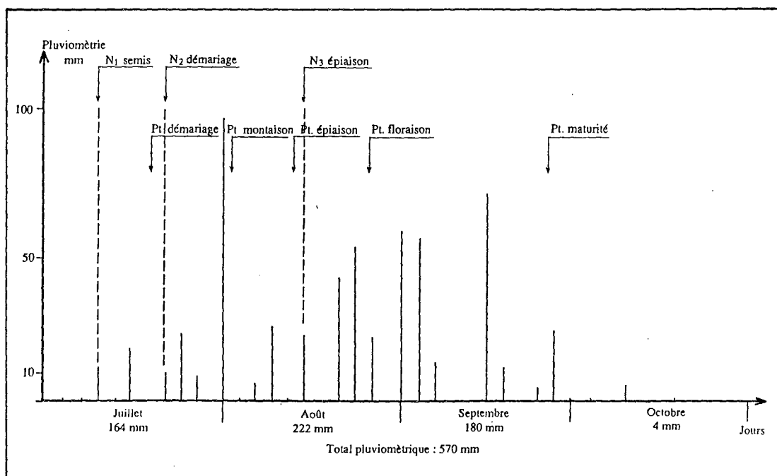
Figure 1 A : Pluviométrie de Bamby en 1975 et cycle végétatif du mil. Pluie cumulée tous les trois jours. Pt = prélèvement de plantes ; N 1 , N 2 et N 3 = apport urée marqué avec 15 N sur mil. Essai au champ I.
