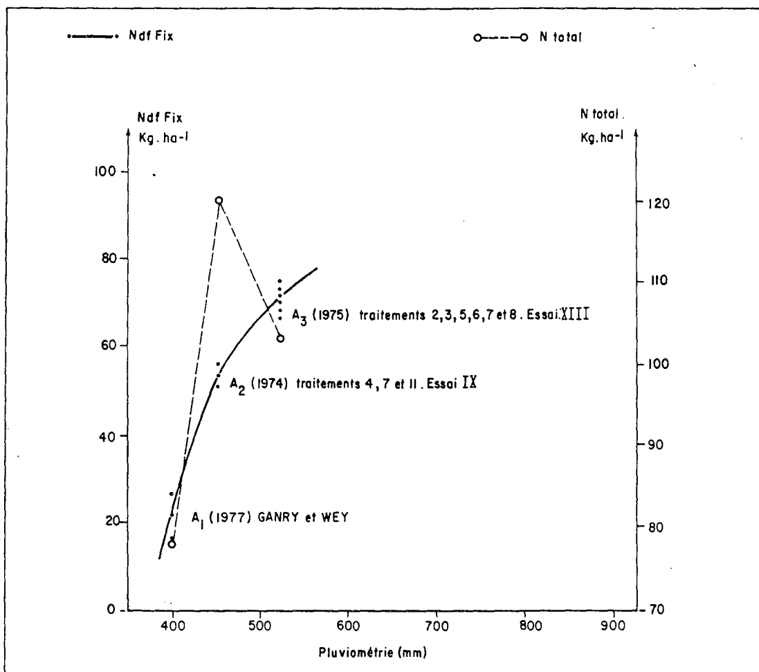
Figure 30 : Relation entre NdfFix de l'arachide ( \text{kg N ha}^{-1} ) et la pluviométrie ( \text{mm an}^{-1} ) (en trait interrompu variation concomitante de N total).
