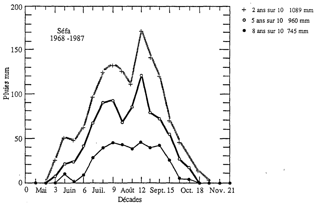
Figure 4 : Espérance de pluviométrie 2, 5 et 8 années sur 10. Stations de Niro et de Séfa. D'après DIAGNE et VANDERSCHMIDT (non publié).
