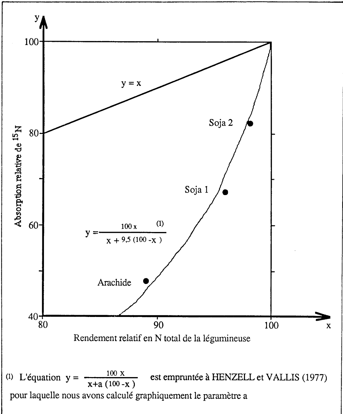
Figure 27 : Absorption relative d'azote ^{15}\text{N} par la légumineuse cultivée avec le mil. Bambeý, essai lysimètre X. Soja 1 : non inoculé, Soja 2 : inoculé.
