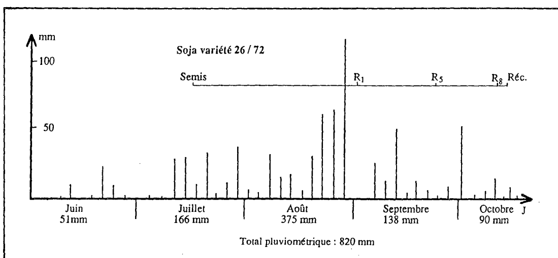
Figure 13 A : Pluviométrie de Séfa en 1982 et cycle végétatif du soja. Pluie cumulée tous les trois jours. Essai au champ XIV.
