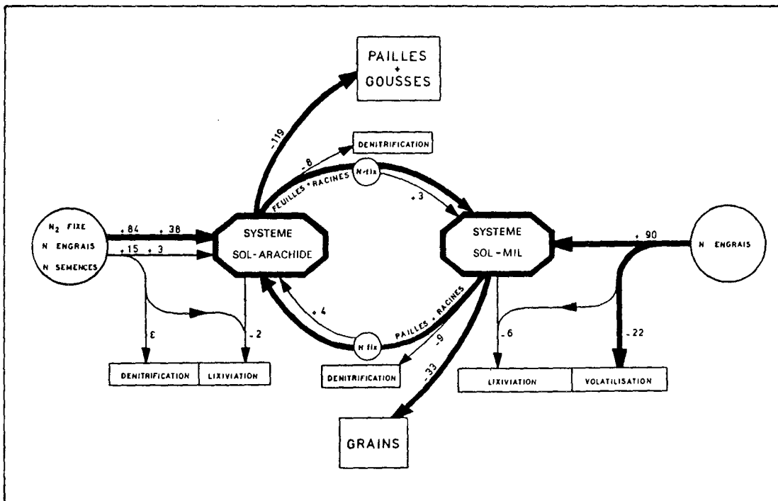
Figure 34 : Schéma montrant les principaux inputs, outputs et transferts azotés dans un système cultural arachide-mil amélioré à Bamboey. Essais I et XIII en 1975.
