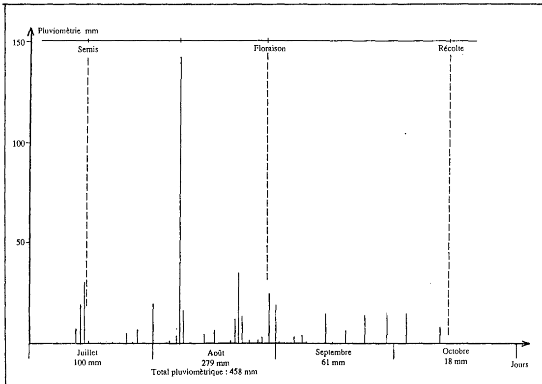
Figure 10 A : Pluviométrie de Banbey en 1974 et cycle végétatif de l'arachide. Essai au champ IX.
