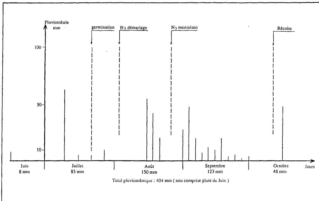
Figure 2 A : Pluviométrie de Bambeï en 1977 et cycle végétatif du nil. Pluie cumulée tous les trois jours. N 2 et N 3 = apport urée marquée avec 15 N sur nil. Essai au champ II.
