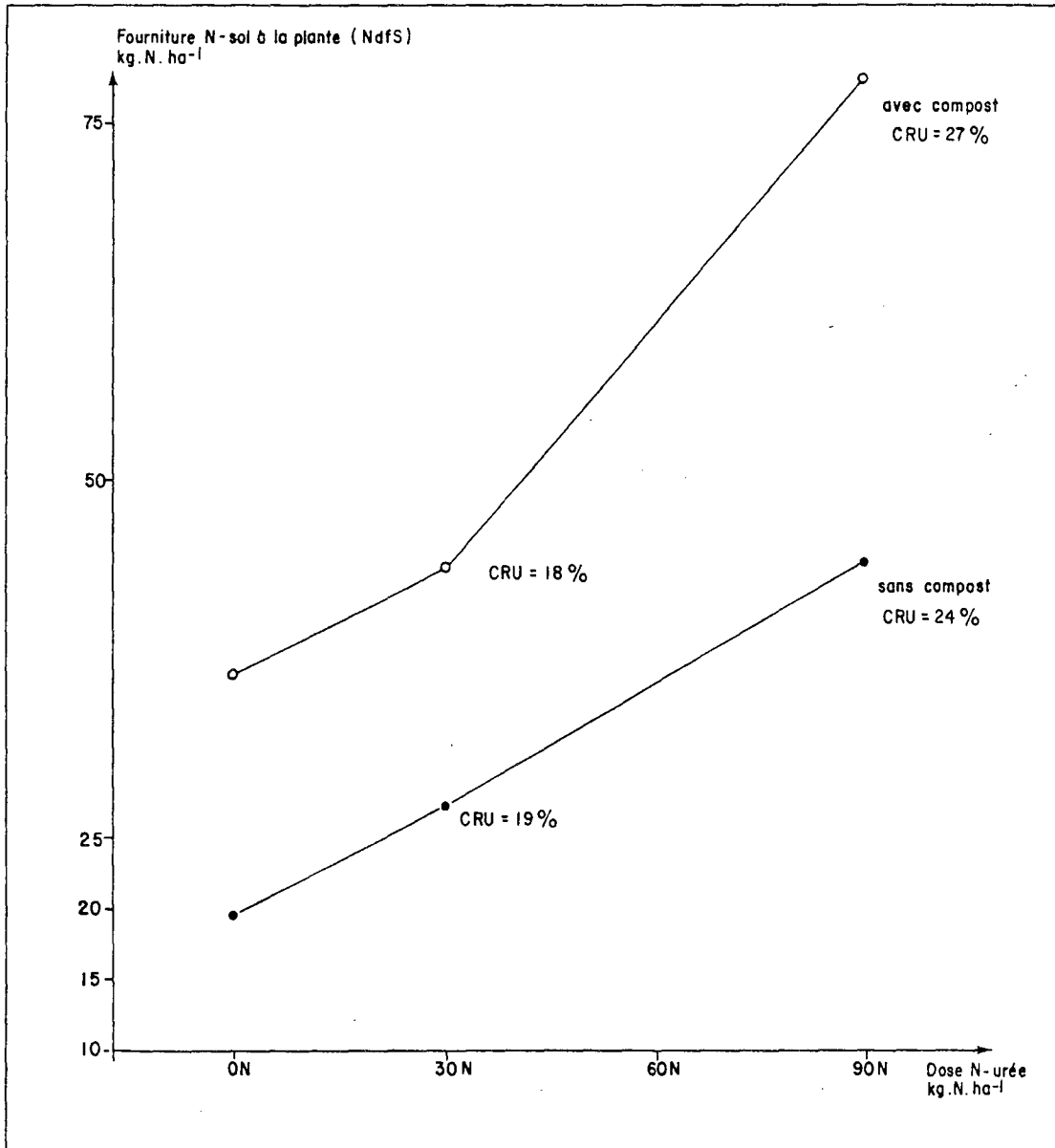
Figure 23 : Valeur de Ndfs du mil sous l'action du compost et de l'urée. Bambeý, essai au champ I.
