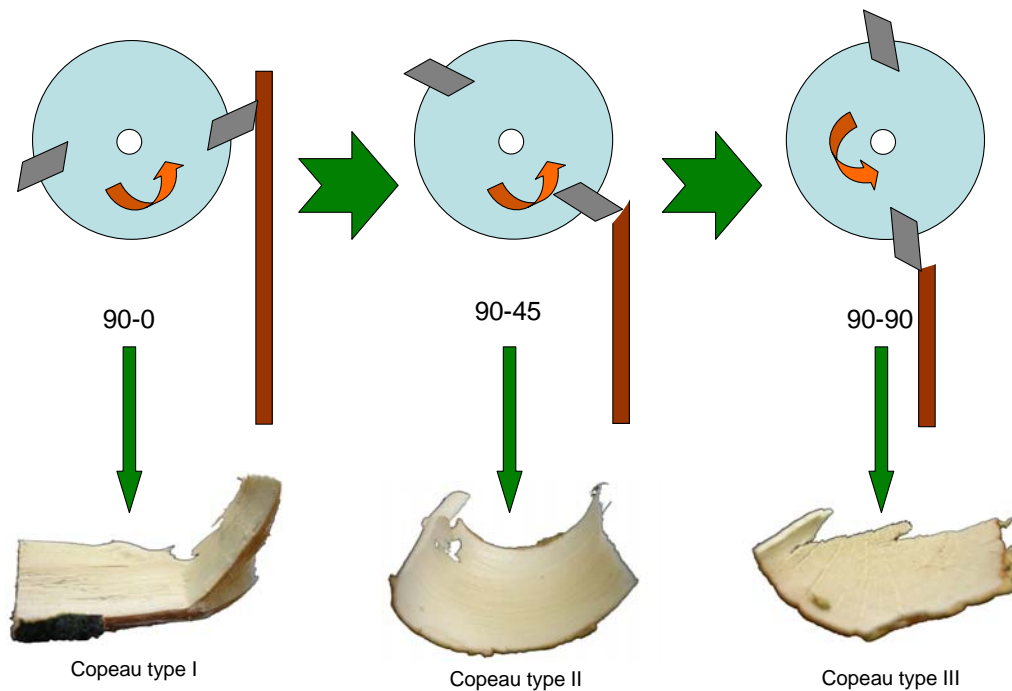
Figure 137 : Types de copeaux rencontrés durant les différentes étapes de l'usinage d'une branche
