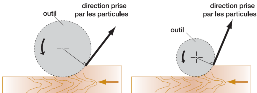
Figure 103 : Variation de la direction de projection en fonction du diamètre d'outil (prise de passe constante)
