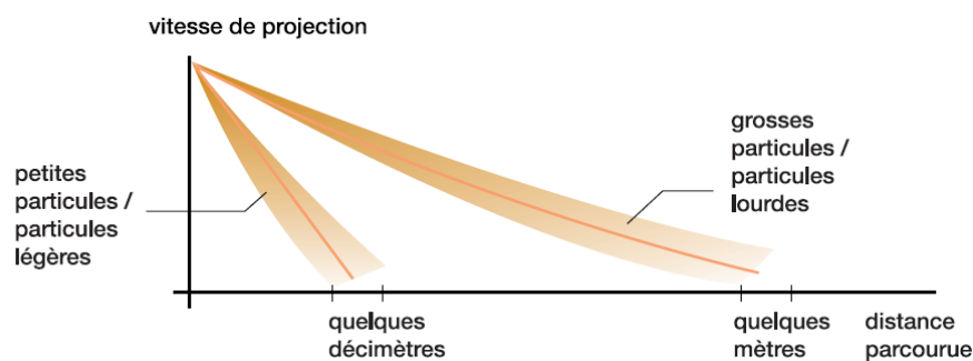
Figure 101 : Distance parcourue par les particules pour une vitesse de coupe donnée [75]
