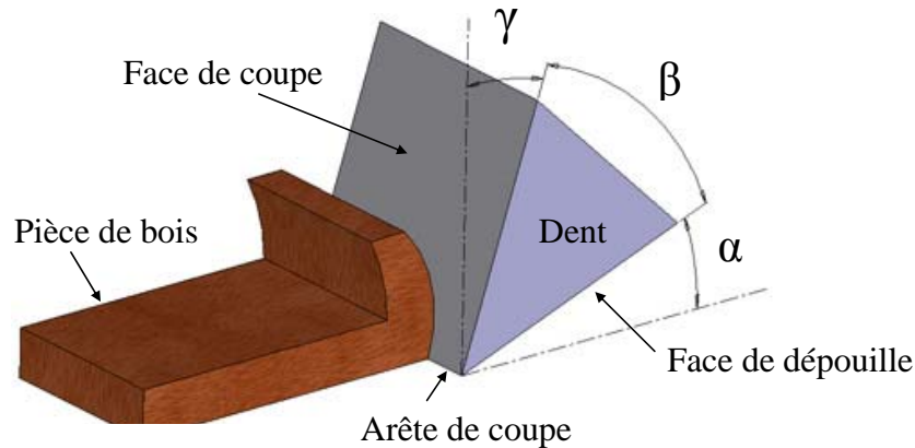
Figure 51 : Définition des angles [NF E 66-502 et 504 ;42 et 43], composition fonctionnelle de la dent
