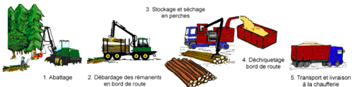
Figure 19 : Production de plaquettes sur bord de route et flux direct
