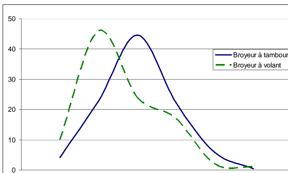
Figure 41 : Comparaison des allures granulométrique entre les broyeurs à tambours et à disque
