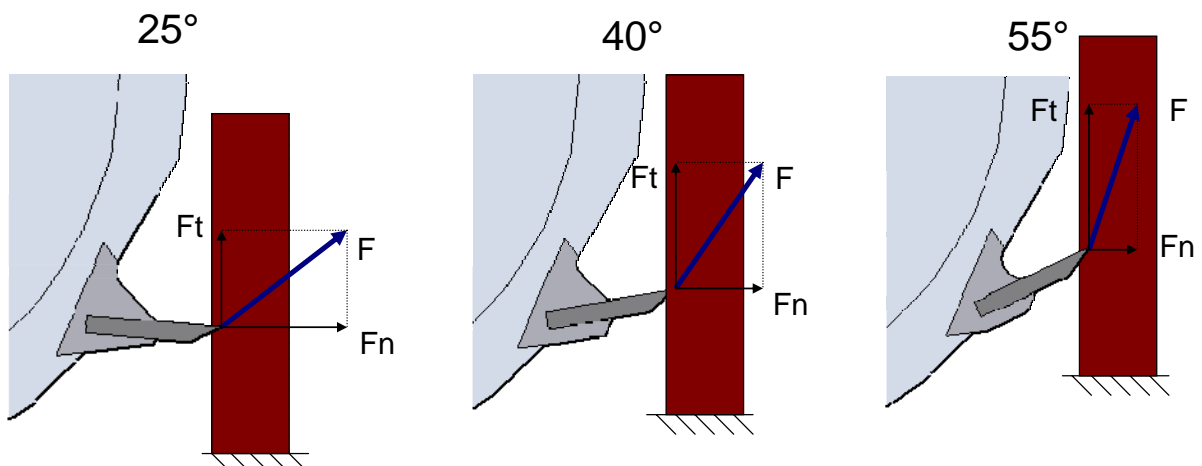
Figure 138 : Variation de la direction d'effort de coupe en fonction de l'angle d'attaque
