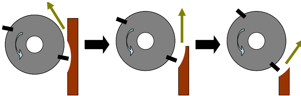
Figure 105 : Variation de la direction de projection des copeaux au cours de l'usinage
