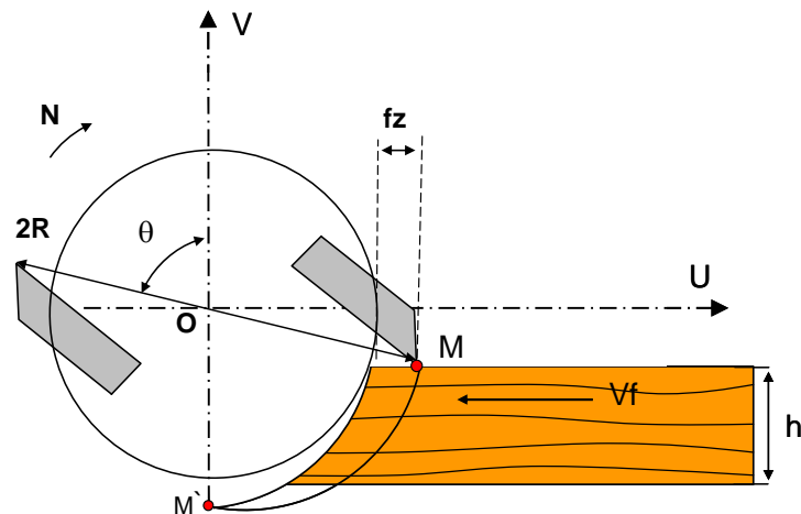
Figure 72 : Récapitulatif des paramètres de coupe influant sur la formation des plaquettes en déchetage par broyeurs à tambour
