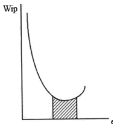
Figure 64 : Courbe du travail spécifique en fonction de l'épaisseur moyenne de copeaux
