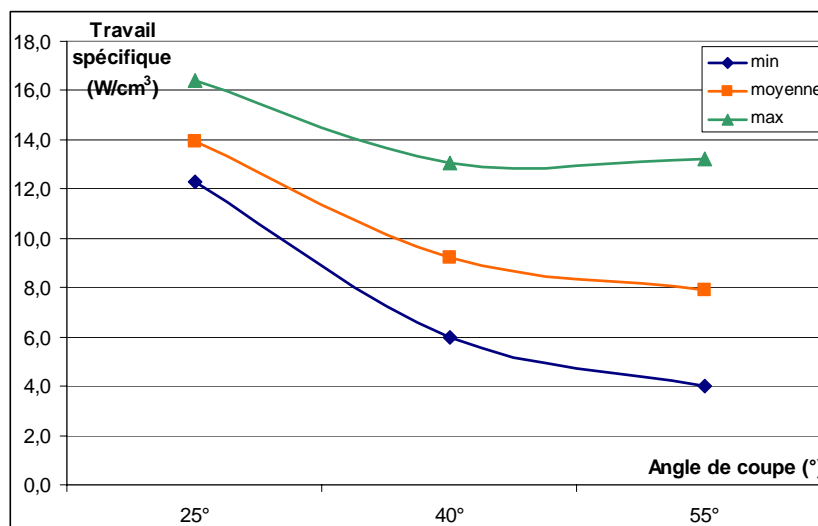
Figure 132 : Travail spécifique mesuré sur tous les essais en fonction de l'angle de coupe des couteaux
