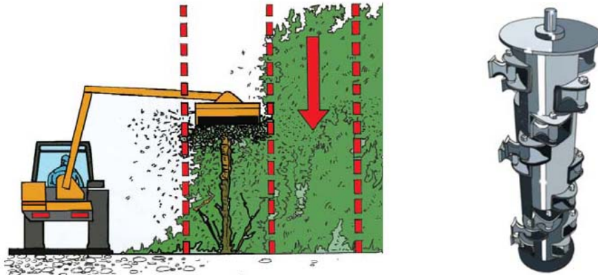
Figure 13 : première solution : le groupe de débroussaillage monté avec un rotor à marteaux (NOREMAT)
