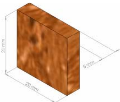
Figure 35 : Dimensions idéales d'une plaquette pour chaudière de particulier [HARGASSNER]
