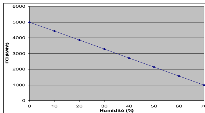
Figure 32 : Evolution du PCI d'un combustible avec son humidité
