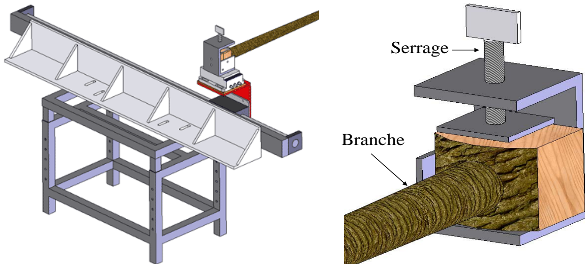
Figure 113 : Vue d'ensemble du système d'aménagement et fixation de la branche sur l'aménagement
