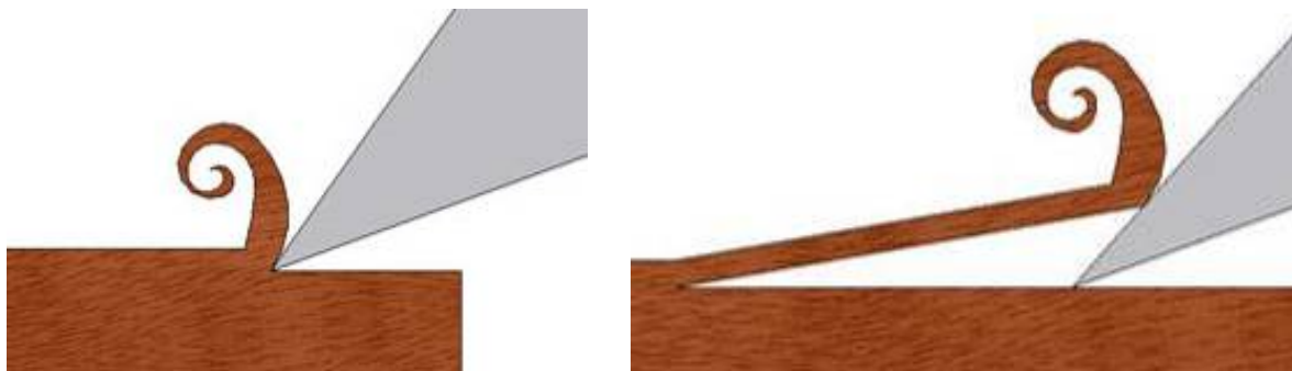
Figure 54 : A gauche : Première phase, recourbement du copeau et à droite : rupture
