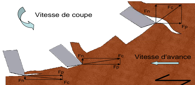
Figure 58 : Formation du copeau en coupe rotative en opposition adapté de BOUCHER [49]
