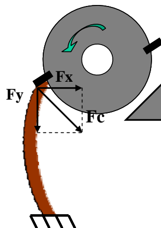
Figure 100 : Effort de coupe mis en jeu lors d'un usinage d'une branche en avalant
