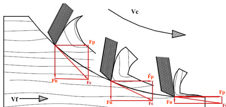
Figure 74 : Formation du copeau en coupe rotative et travail en avalant
