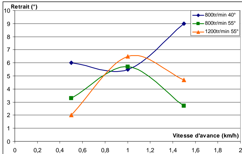
Figure 134 : Evolution du retrait des branches en fonction de la vitesse d'avance pour trois essais différents
