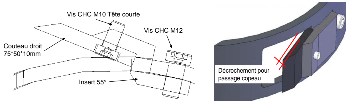
Figure 145 : Schéma de montage des copeaux par les inserts, vue de dessus (à gauche) et vue d'ensemble (à droite).
