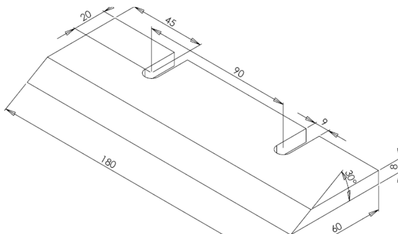
Figure 91 : Schématisation des couteaux utilisés
