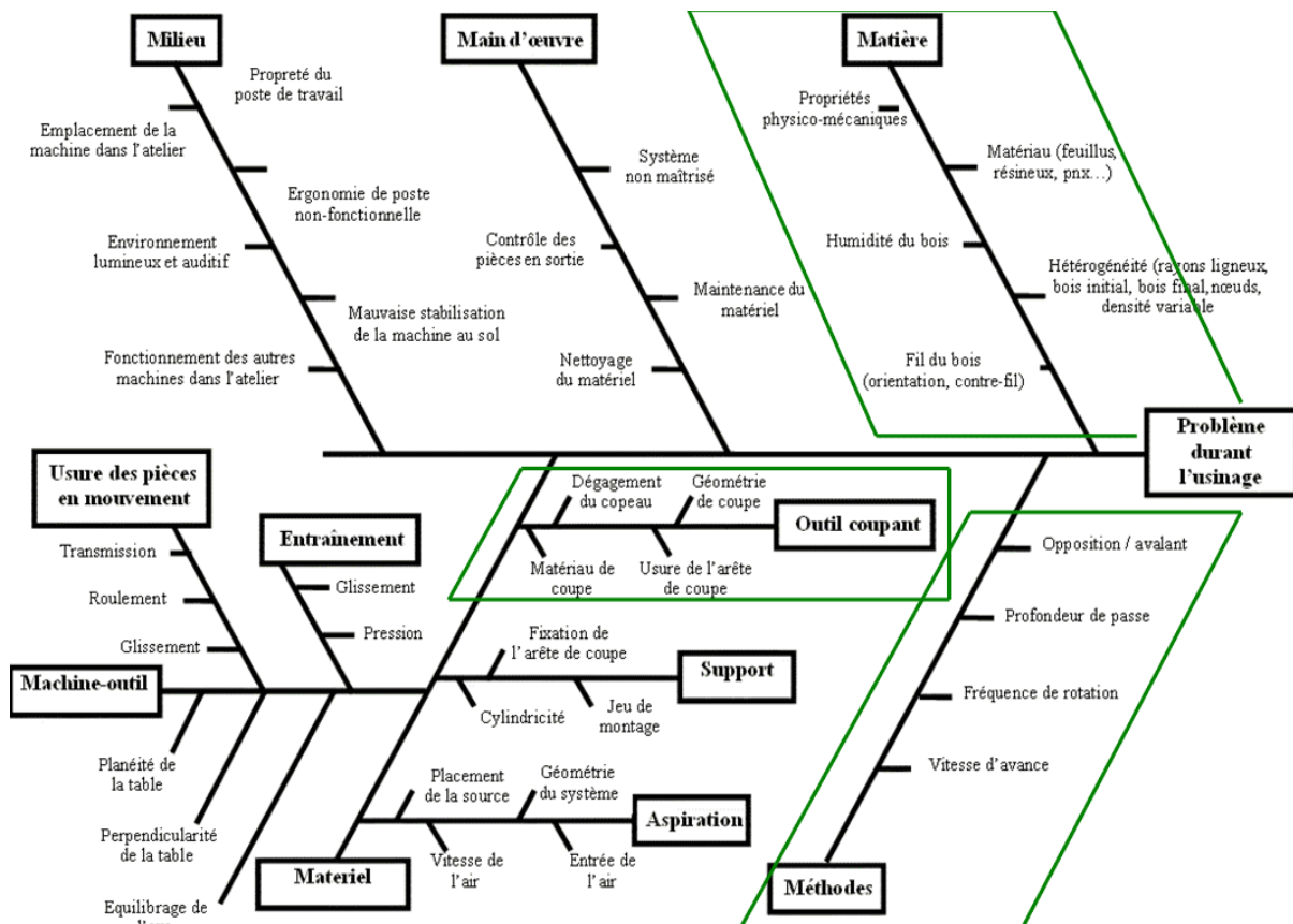
Figure 59 : Diagramme causes-effet recensant les causes possibles des problèmes pouvant intervenir en usinage bois [BOUCHER ;49]
