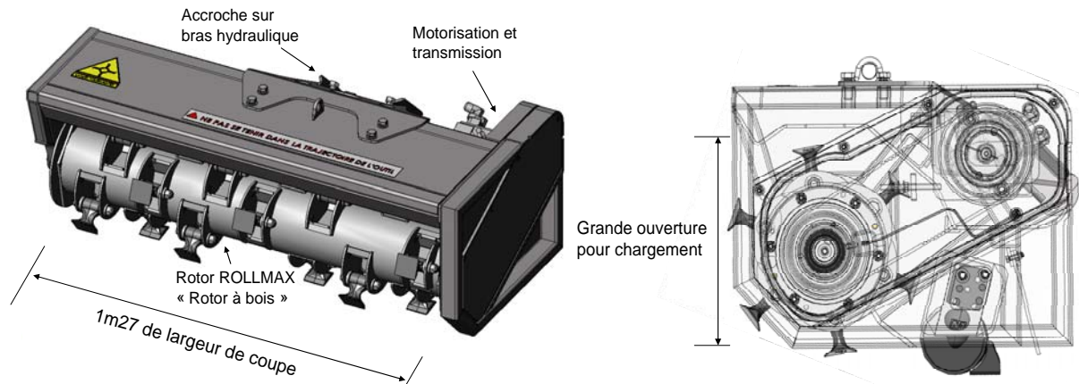
Figure 140 : Présentation du ROLL MAX (rotor actuellement utilisé) et du groupe FOREST BROYEUR de chez NOREMAT
