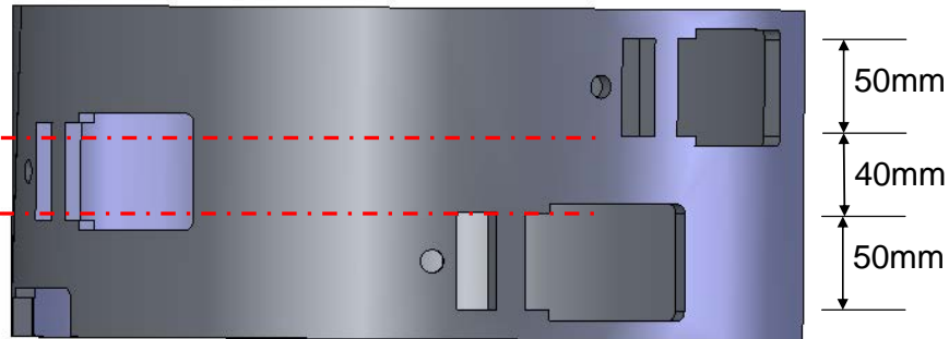
Figure 143 : Recouvrement des zones de coupe
