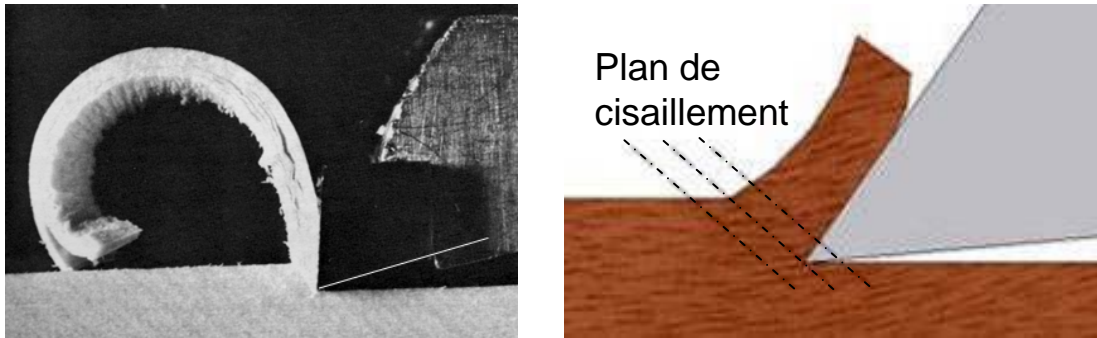
Figure 56 : Copeau de Type 2, « à compression faible » photo (KOCH) et schéma
