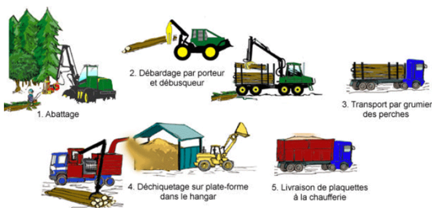
Figure 20 : Production de plaquettes sur plate-forme et flux indirect
