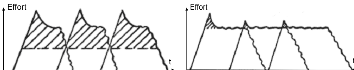
Figure 67 : A gauche, effort de coupe pour un outil droit, à droite pour un outil hélicoïdal [STEWART ;55]
