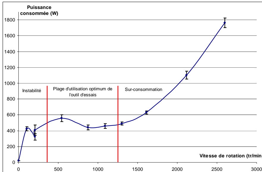
Figure 116 : Evolution de la puissance électrique consommée pour la rotation simple de l'outil
