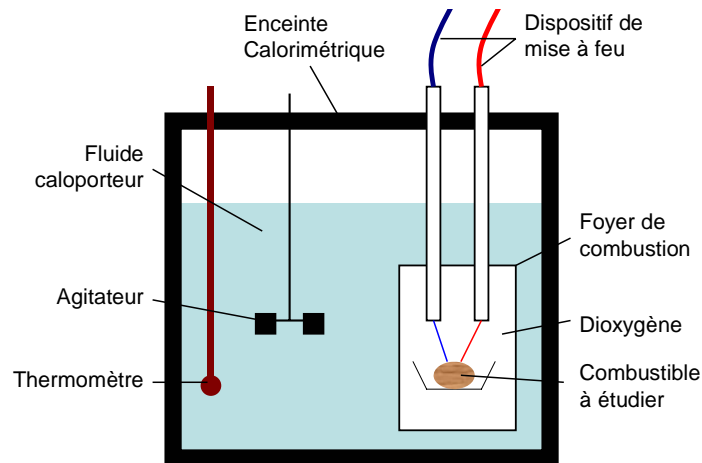
Figure 31 : Schéma de fonctionnement d'une bombe calorimétrique
