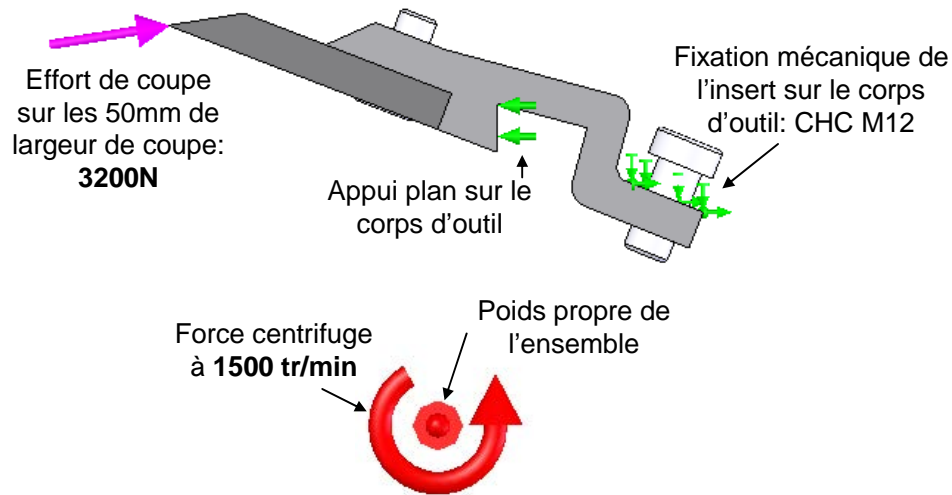
Figure 146 : Chargement du système lors de la coupe d'une branche
