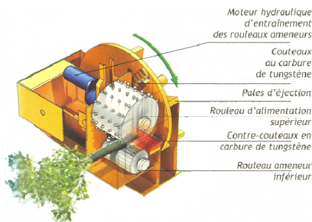
Figure 38 : Broyeur à disque (NOREMAT)
