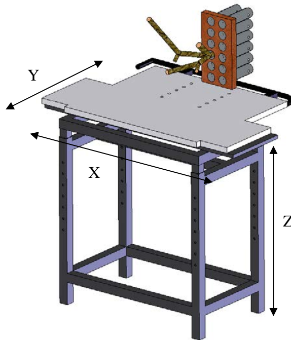
Figure 43 : Dispositif d'aménagement réglable
