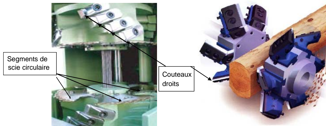
Figure 77 : A gauche le canter profileuse de chant et à droite le canter latéral
