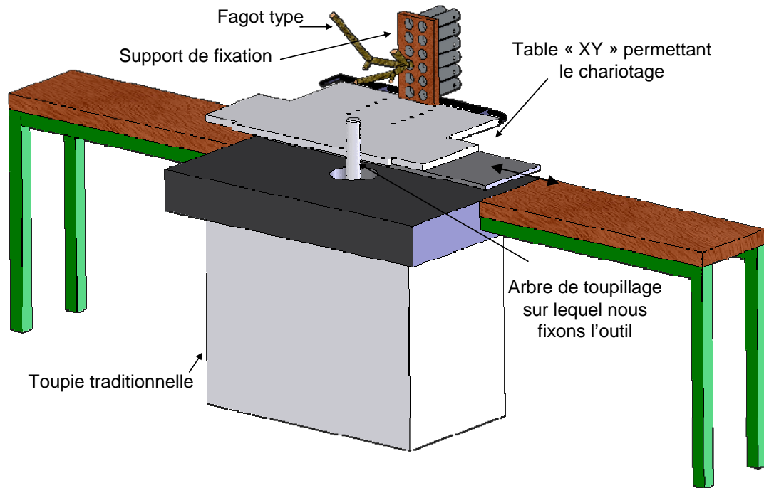
Figure 48 : Dispositif de montage pour tester le rotor à couteau
