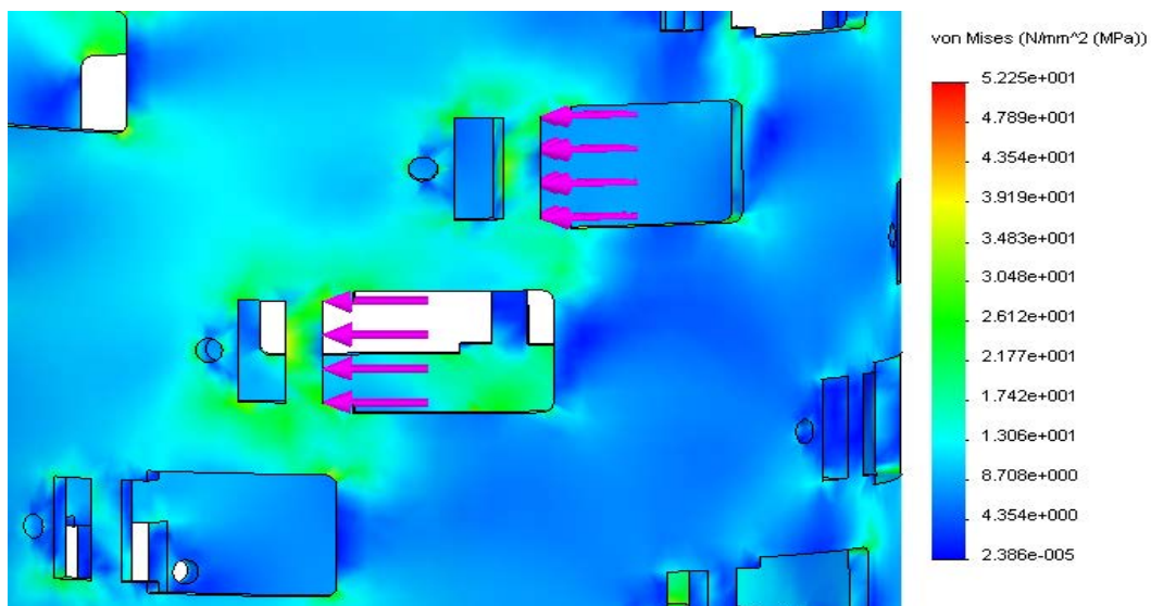
Figure 149 : Répartition des contraintes autour des ouvertures sur le corps d'outil
