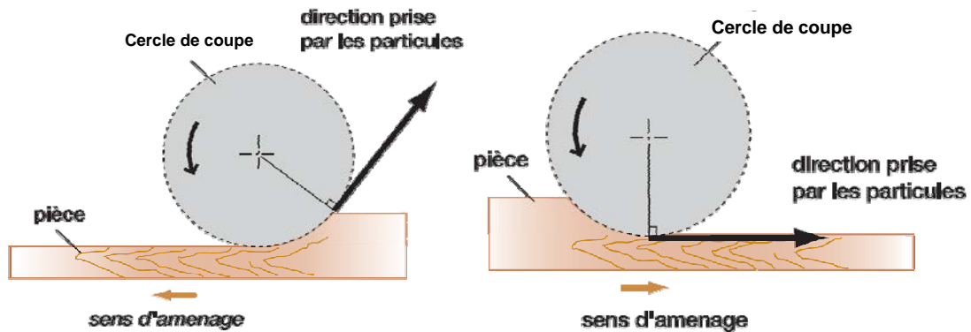
Figure 102 : A gauche, direction de projection lors d'un travail en opposition et à droite, en avalant [75].
