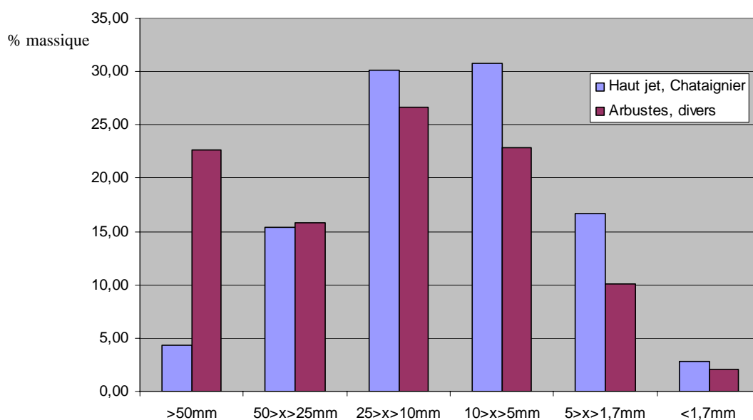
Figure 160 : Comparaison granulométrique entre de coupe d'arbres de haut jet et la coupe d'arbustes.
