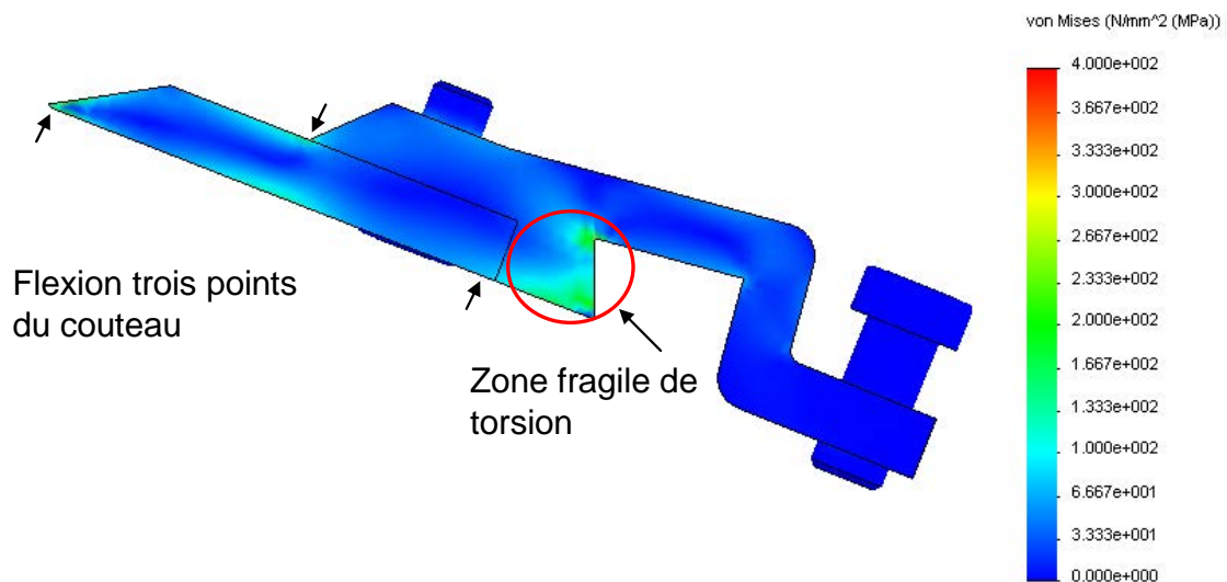
Figure 147 : Contraintes résultantes dans l'ensemble {couteau+insert+vis}
