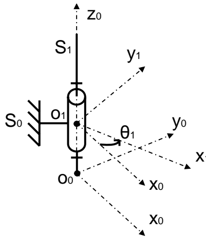
Figure 92 : Schéma cinématique de l'outil d'essais
