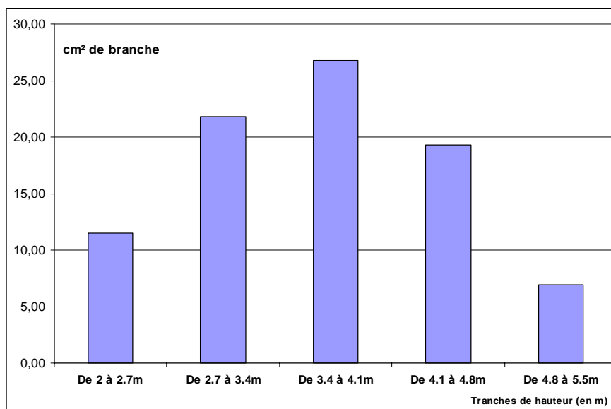
Figure 41 : Densité de surface de coupe exprimée en cm 2 de surface de coupe par m 2 de haie
