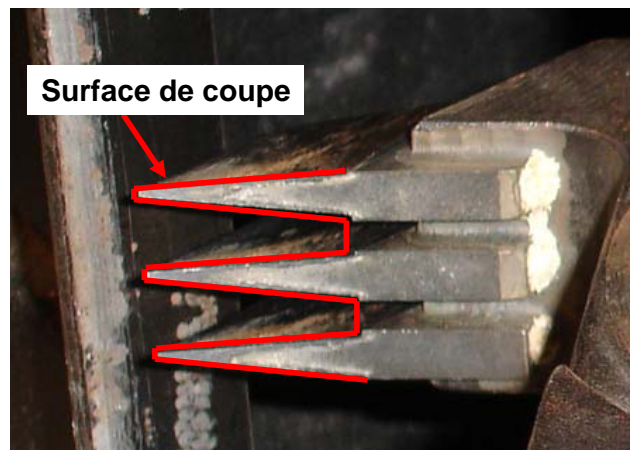
Figure 57 : Déplié de la surface de contact bois/outil
