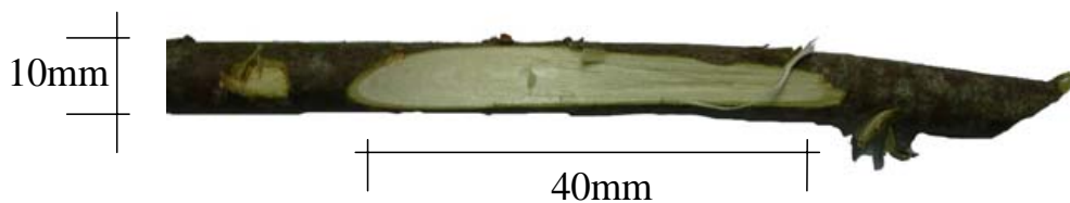
Figure 122 : Etat de surface d'une branche de 10mm de diamètre amenée à 3km/h et coupée à 400tr/min
