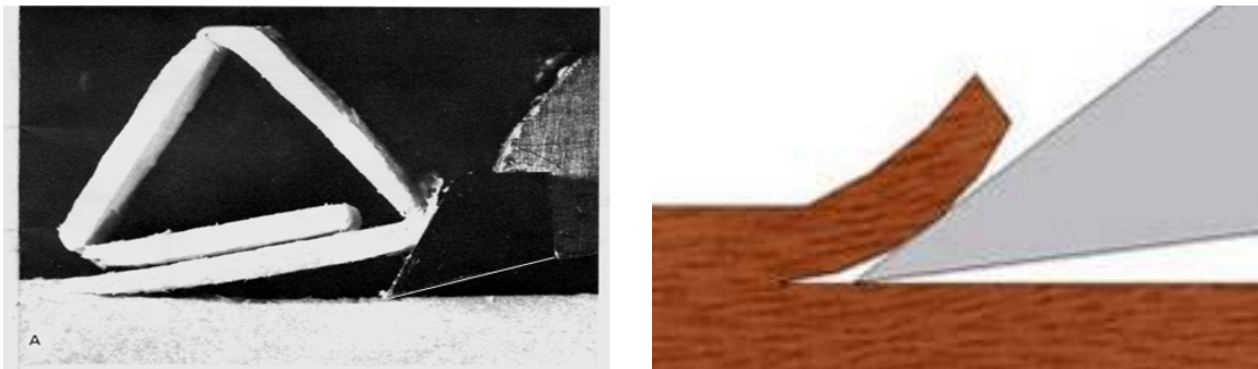
Figure 55 : Copeau de Type I, « continu » photo (KOCH) et schéma
