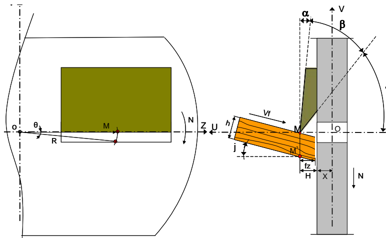
Figure 70 : Récapitulation des paramètres de coupe influant sur la formation des plaquettes en déchiquetage par broyeur à disques.
