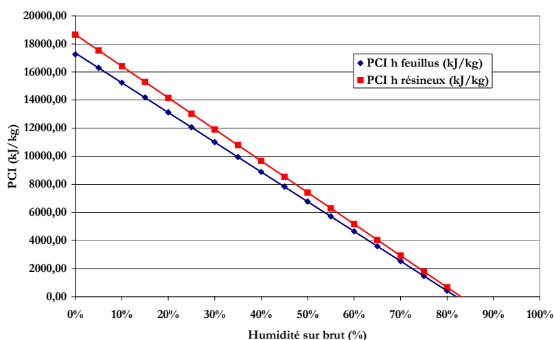
Figure 30 : Evolution du pouvoir calorifique inférieur des plaquettes en fonction de l'humidité sur brut
