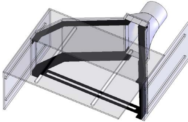
Figure 114 : Module d'aspiration de copeaux
