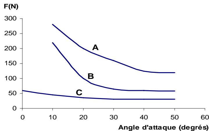
Figure 50 : Variation de l'effort de coupe suivant les modes A, B ou C pour du Hêtre à 12% d'humidité, copeau de 0.2mm d'épaisseur, outil usé à 50% [MARTIN ;38]
