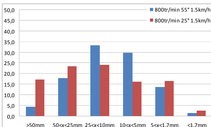
Figure 127 : Répartition granulométrique de deux usinages identiques avec deux angles de coupe différents.
