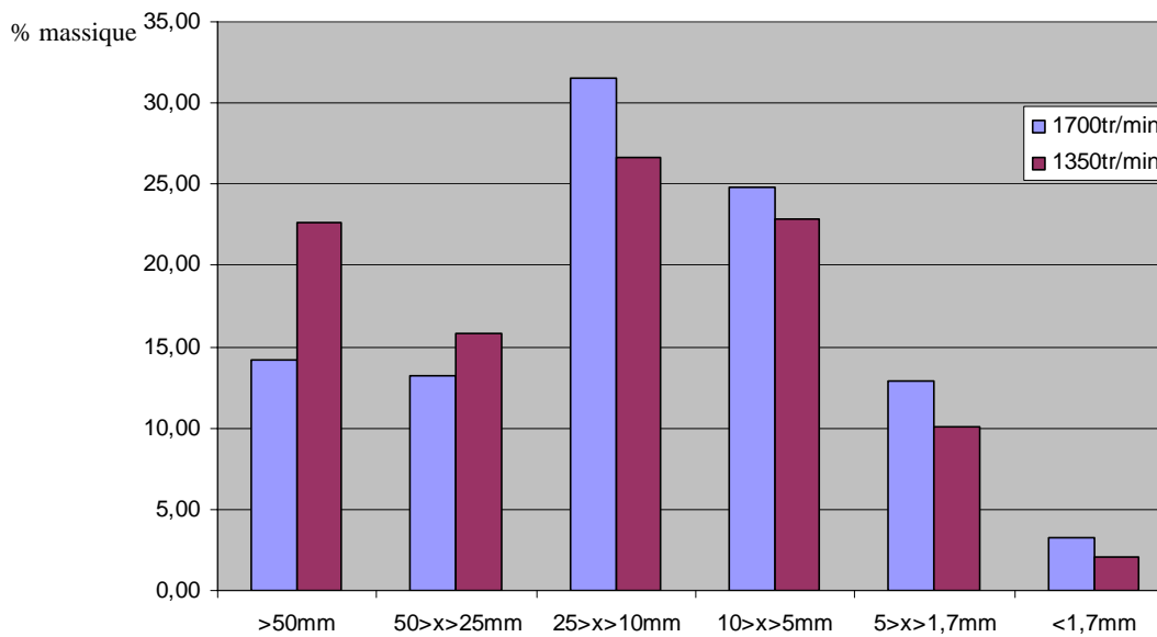
Figure 159 : Comparaison granulométrique entre deux vitesses de rotation de l'outil
