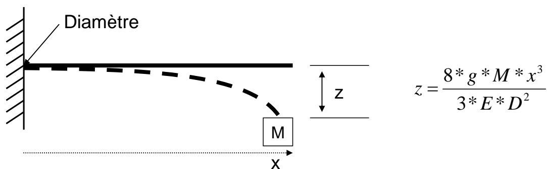
Figure 34 : Schéma de principe des essais de flexion et formules consacrées
