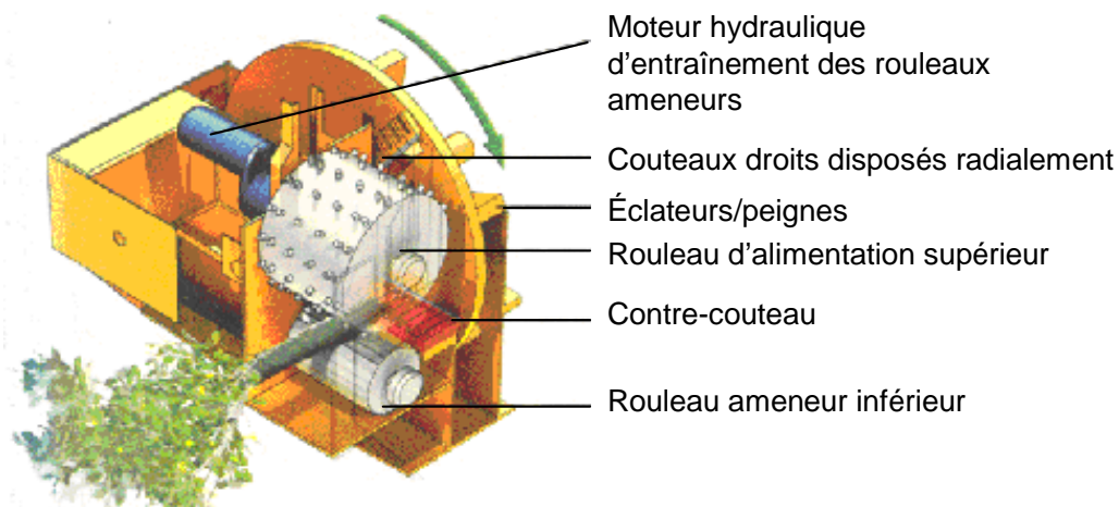
Figure 69 : Principe de fonctionnement d'un broyeur à disque (NOREMAT)
