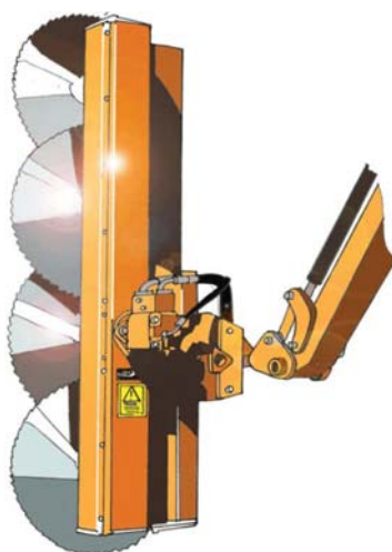
Figure 16 : deuxième solution : le lamier, ici à 4 lames
