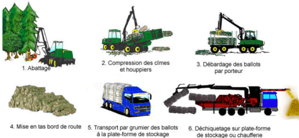
Figure 21 : Production de plaquettes sur plate-forme à partir de houppiers compactés
