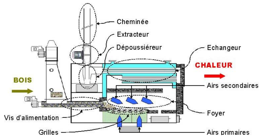
Figure 15: Présentation générale d'une chaudière à bois automatique
