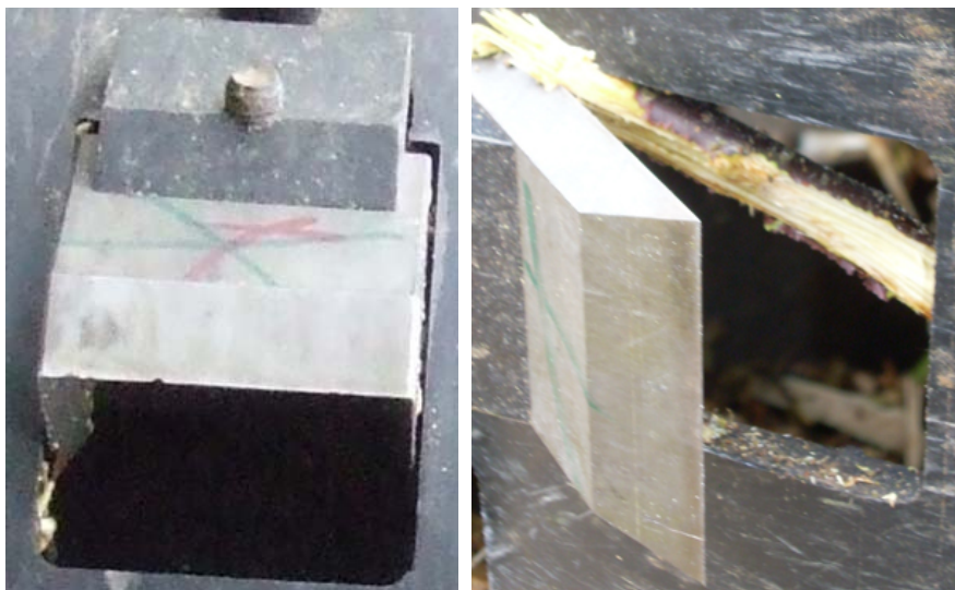
Figure 157 : à gauche couteau en U propre et à droite branche coincée dans un couteau droit
