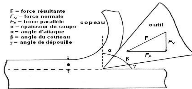
Figure 53 : Géométrie de coupe et composantes des forces de coupe [KOCH ;45]
