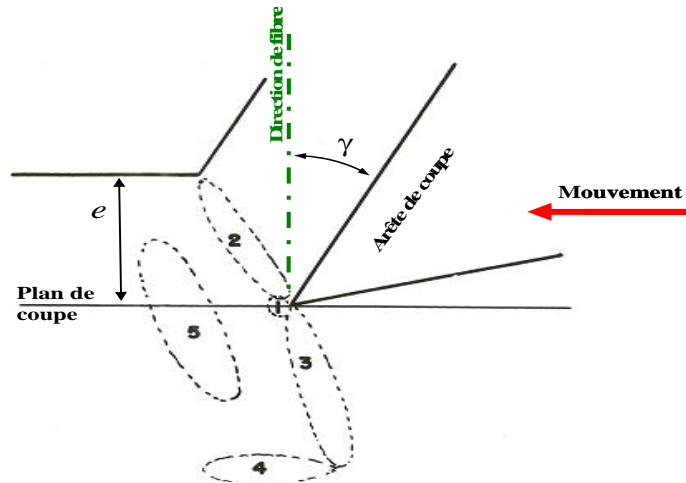
Figure 75: Les zones de rupture potentielle en mode de coupe A.
