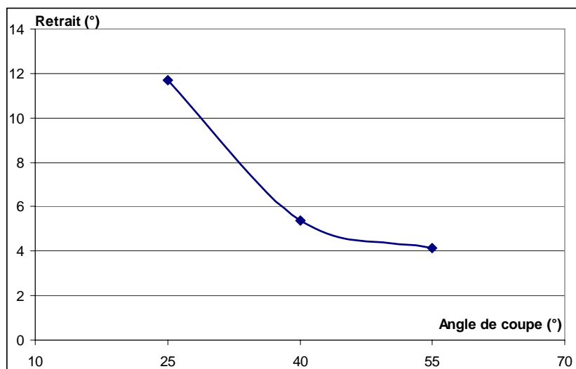
Figure 135 : Evolution du retrait de la branche face à l'outil en fonction de l'angle de coupe, moyenne effectuée sur toutes les mesures
