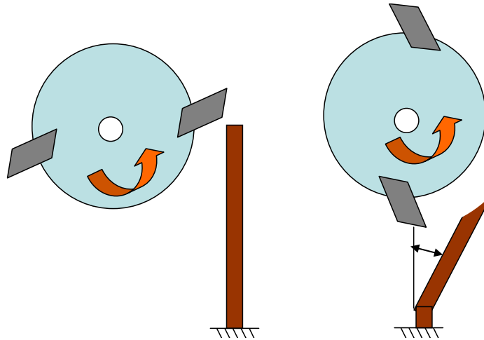
Figure 119 : Représentation de l'angle d'effacement de la branche devant l'outil
