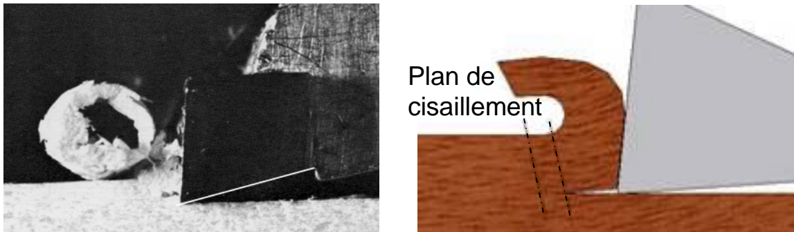
Figure 57 : Type 3, « à compression forte » photo (KOCH) et schéma
