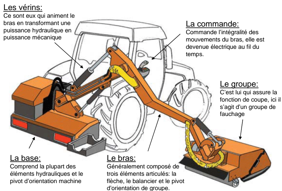
Figure 12 : Schéma de fonctionnement général d'un bras hydraulique NOREMAT
