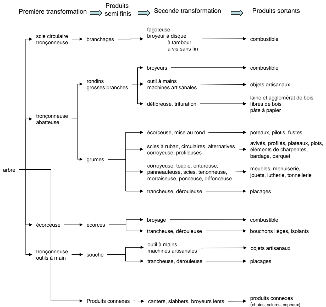
Figure 18 : Détail non exhaustif des machines et process dans la première et seconde industrie du bois, adapté de MARTIN [12]
