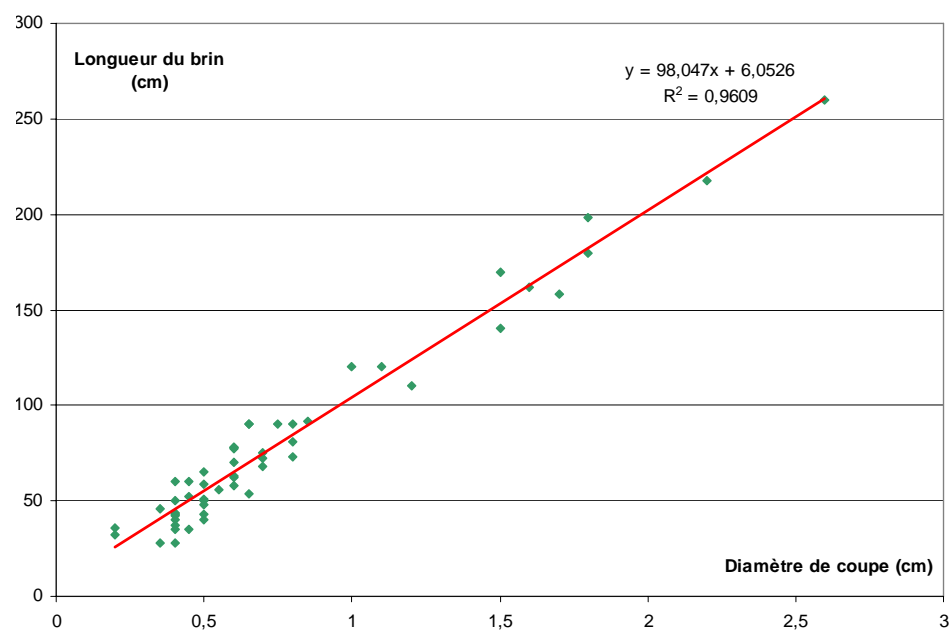
Figure 28 : Longueur du brin coupé en fonction du diamètre de coupe, courbe de régression linéaire
