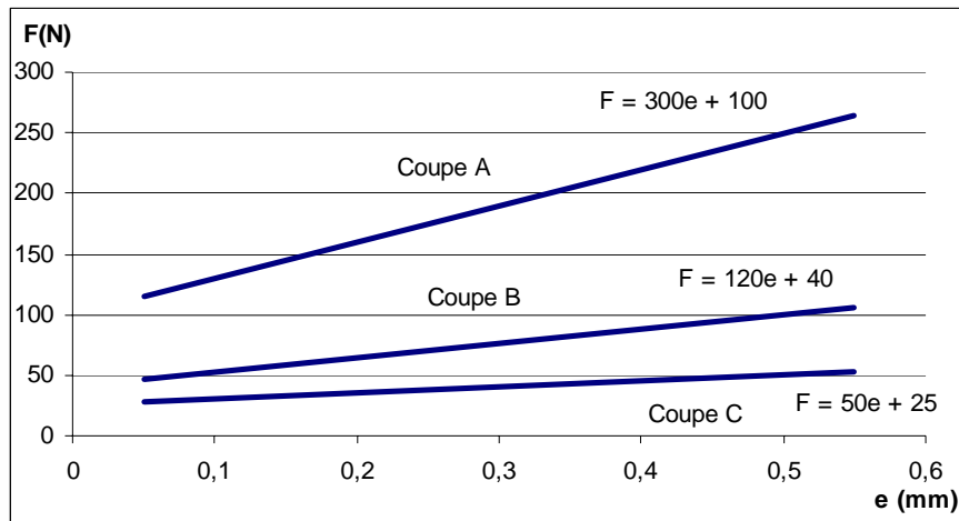
Figure 63 : Force nécessaire à la coupe (largeur : 1cm) en fonction de l'épaisseur du copeau suivant les directions de coupe (hêtre à 12% et \gamma=30^\circ ) [MARTIN;38]
