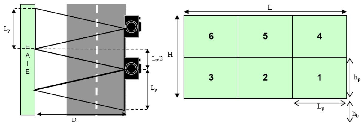
Figure 37 : A gauche, prise de photos, vue de dessus et à droite vue de face
