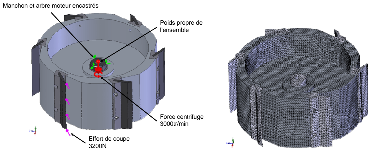
Figure 94 : A gauche, chargement du système lors de la coupe d'une branche de 5 cm et à droite maillage du système.
