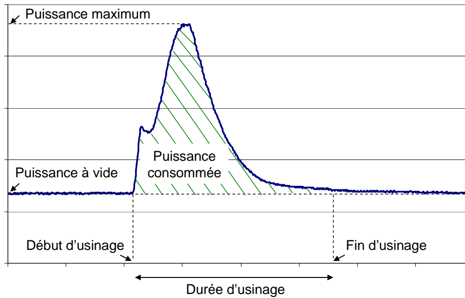
Figure 117 : Description des critères de traitement d'un signal de puissance
