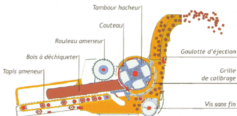
Figure 39 : Broyeur à tambour (NOREMAT)
