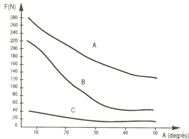
Figure 65 : Influence de l'angle de coupe \gamma suivant les modes de coupe A, B et C (cas du hêtre à 12% d'humidité, copeau de 0.2mm, outil usé à 50%)
