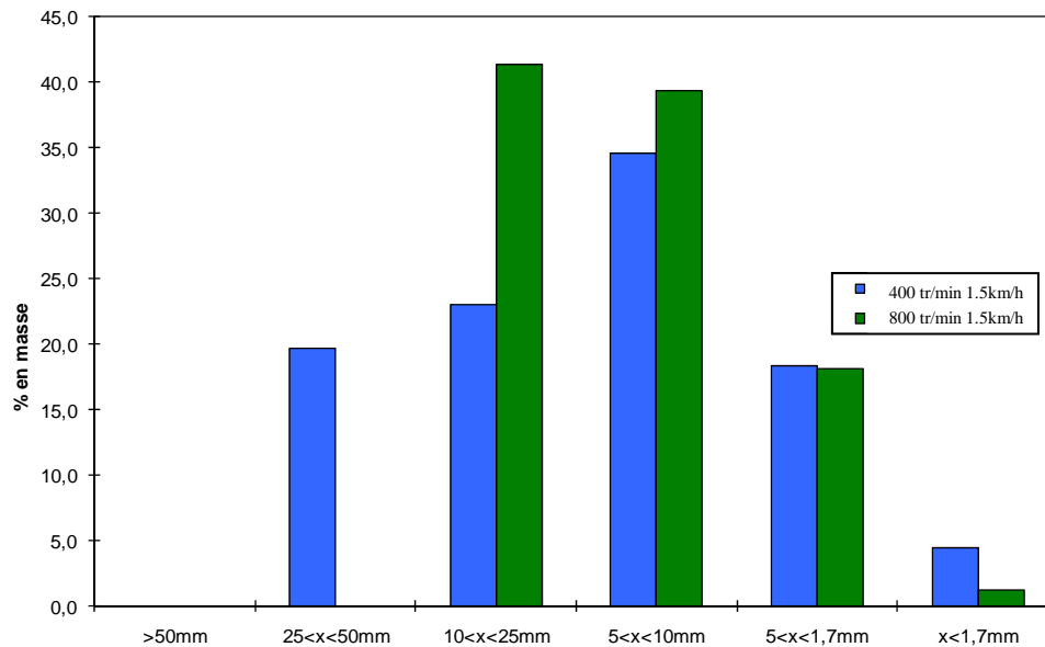
Figure 125 : Comparaison granulométrique entre un usinage à 400 tr/min et à 800tr/min
