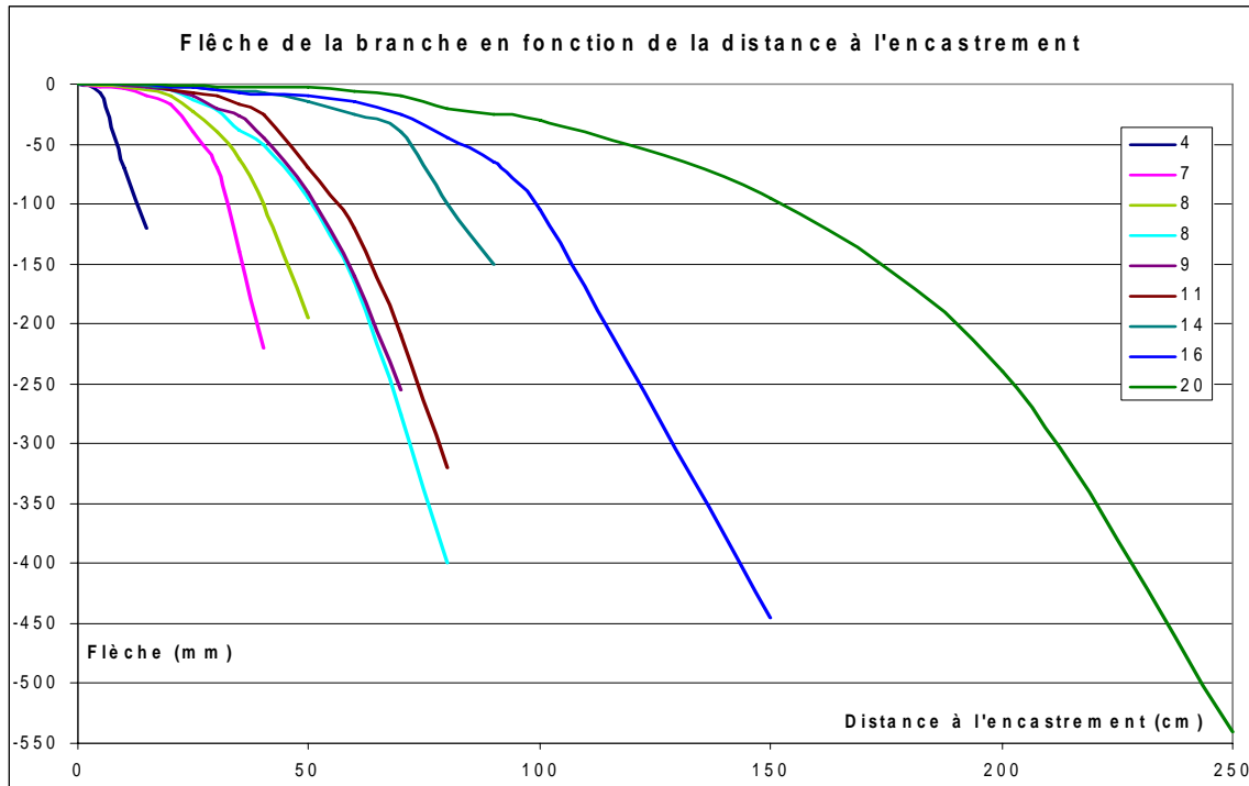
Figure 35 : Résumé des données de flexion obtenues en fonction des différents diamètres
