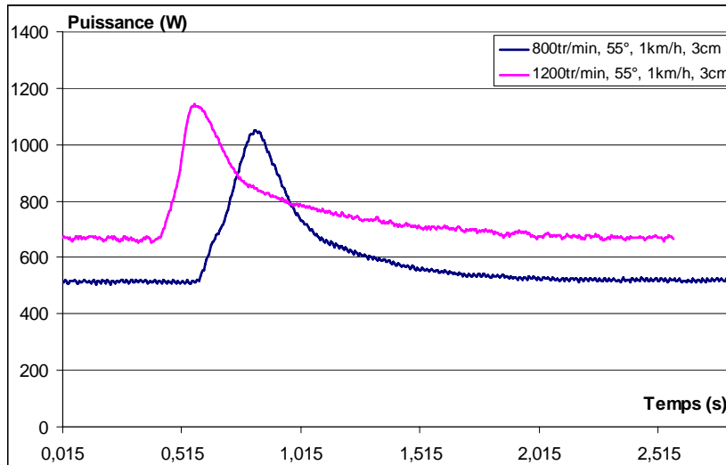
Figure 131 : Evolution de la puissance électrique consommée pour deux usinages aux conditions identiques mais avec une vitesse de rotation différente
