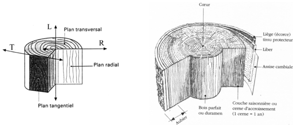
Figure 47 : A gauche : direction d'anisotropie, à droite : structure par cernes du bois
