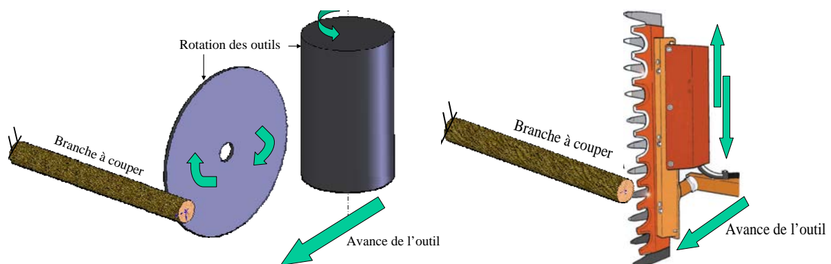
Figure 45 : à gauche principe des outils de rotation et à droite celui des translations orthogonales.
