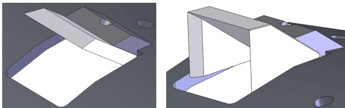
Figure 156 : à gauche, couteau droit élargi et à droite couteau en U à trois arêtes de coupe.
