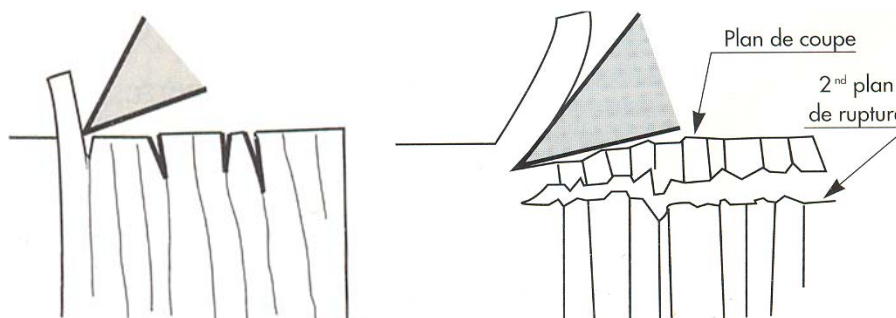
Figure 76 : propagation des fissures lors du passage de l'outil avec, à gauche un bois de bonne cohésion et, à droite, un bois de plus mauvaise cohésion.
