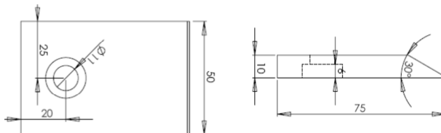
Figure 144 : Vue de dessous et de côté des couteaux droits utilisés
