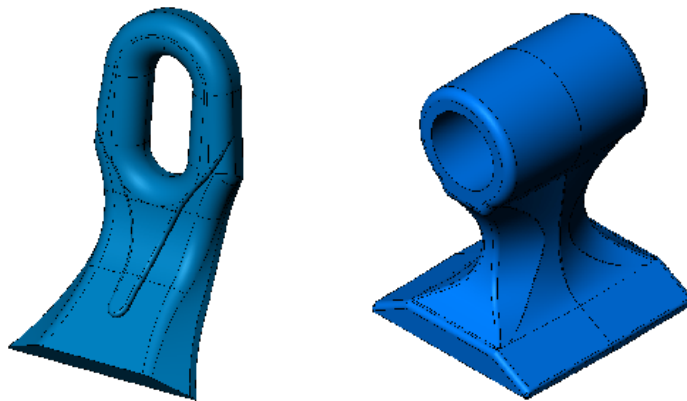
Figure 14 : A gauche : fléau pour les faibles diamètres de branches (max 2cm) et à droite : marteau pour les diamètres plus importants (pièces NOREMAT)
