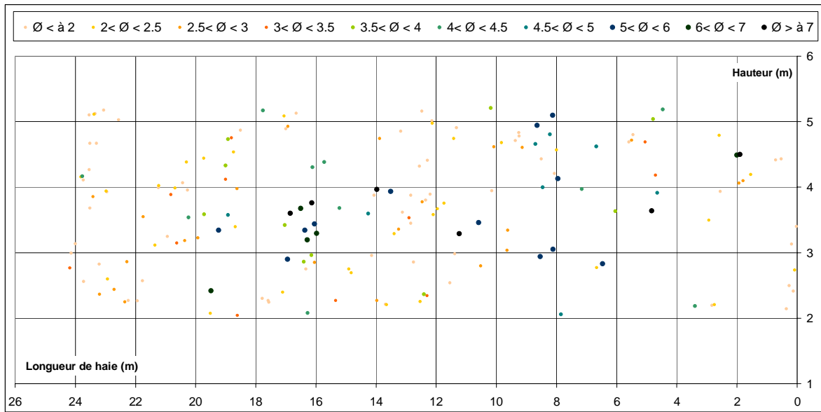
Figure 39 : Position des différentes classes de diamètre de branche (cm) sur une haie de bord de route.
