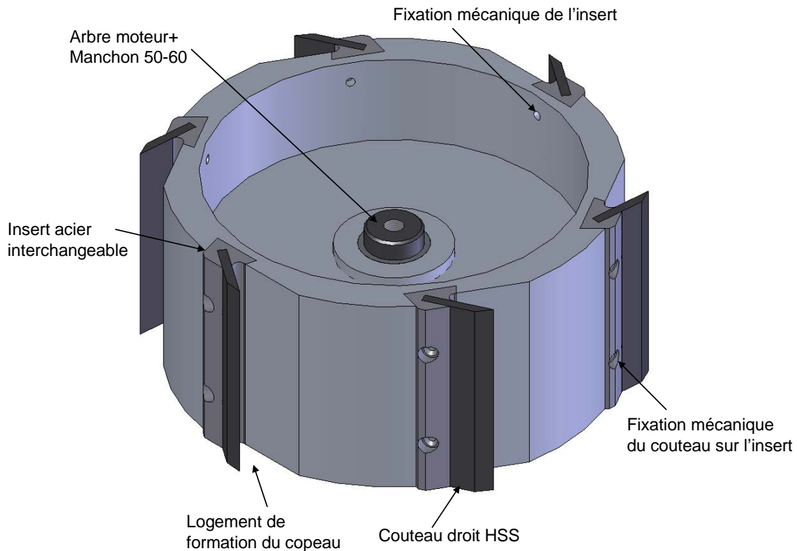
Figure 87 : Présentation de l'outil de laboratoire.
