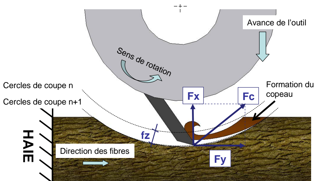
Figure 98 : Description de la coupe et mise en place des efforts de coupe (vue de dessus)
