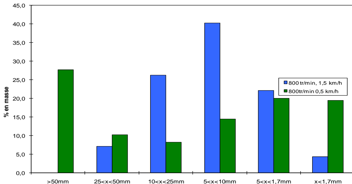
Figure 126 : Comparaison granulométrique de deux usinages identiques avec deux vitesses d'avance différentes
