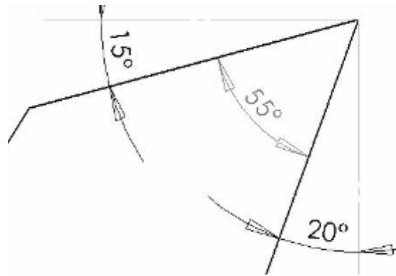
Figure 56 : Angles de coupe utilisés sur l'outil à enturer
