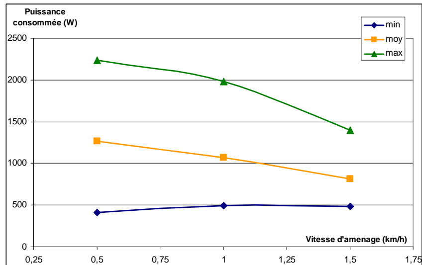
Figure 130 : Puissance consommée de tous les tests en fonction de la vitesse d'amenage
