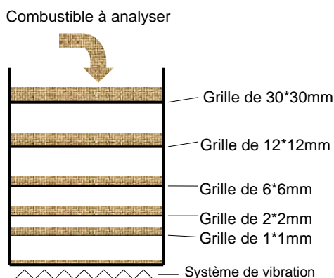
Figure 34 : Schéma de principe de la mesure granulométrique par tamis horizontal vibrant
