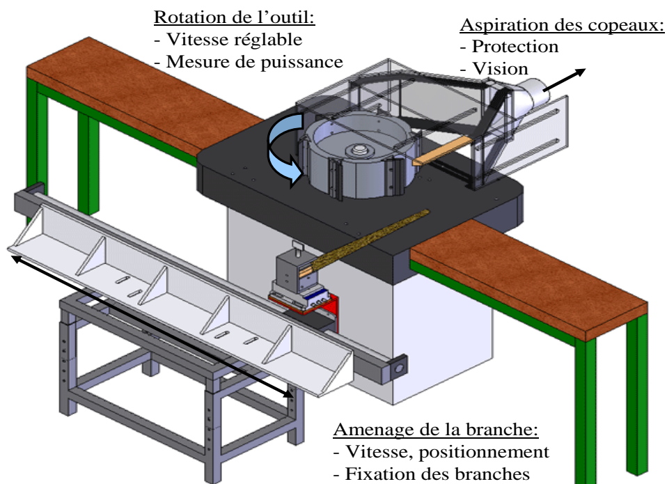
Figure 112 : Dessin CAO de la partie coupe du banc d'essais avec descriptif des différents organes présents.
