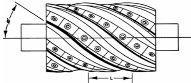
Figure 66 : Porte outil hélicoïdal type outil de raboteuse avec \Phi l'angle d'hélice [STEWART 55]
