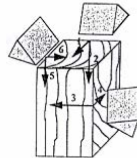
Figure 49 : Définition des modes de coupe par MC KENZIE [41]
