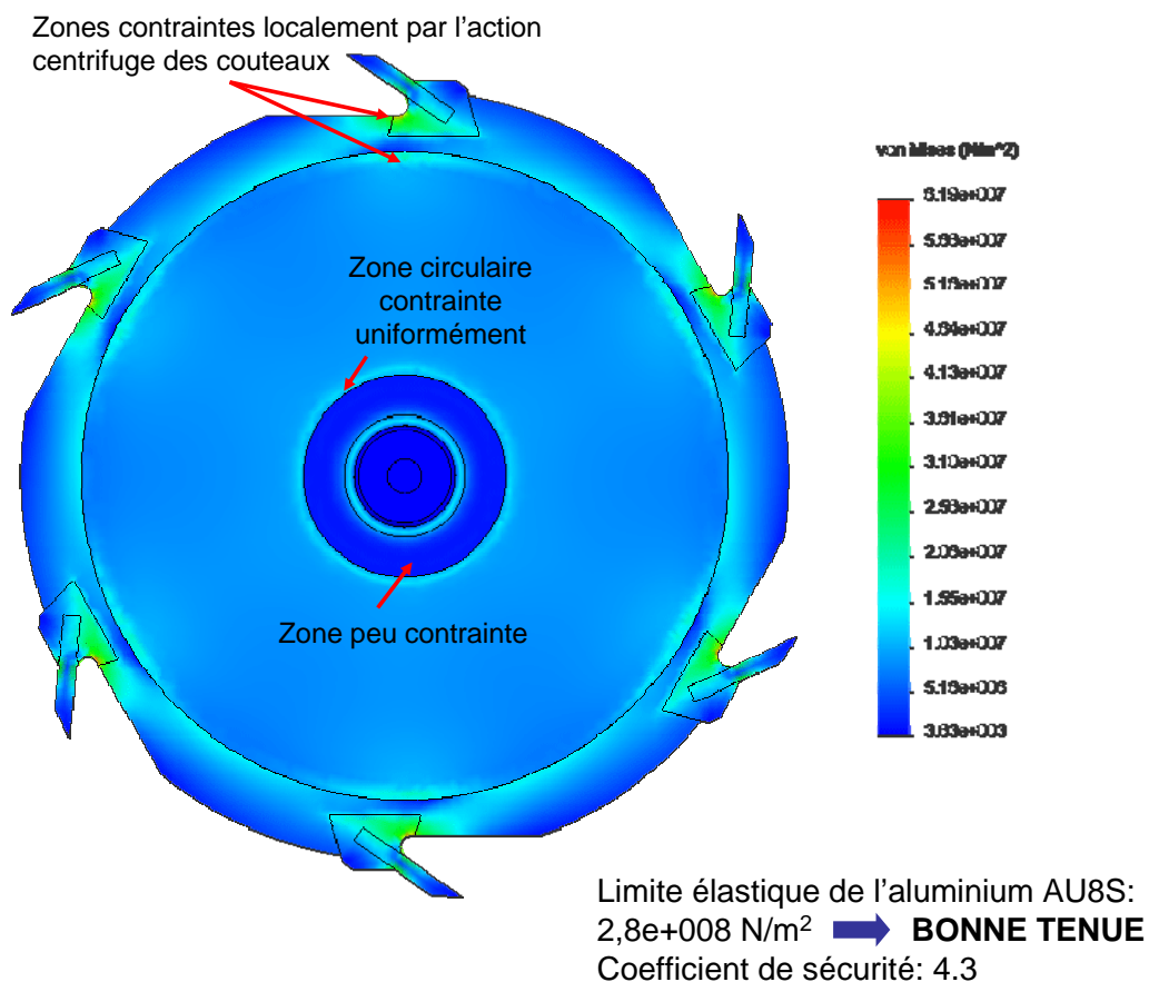
Figure 95 : Répartition des contraintes dans l'outil lors de l'usinage
