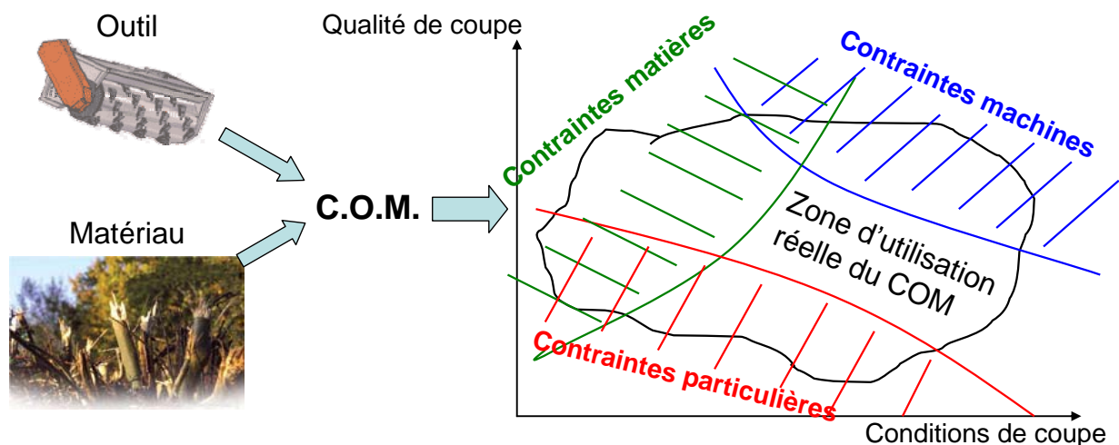
Figure 4 : Principe de fonctionnement du Couple {Outil-Matière} [adapté de NORME E66-520-1 ;6]
