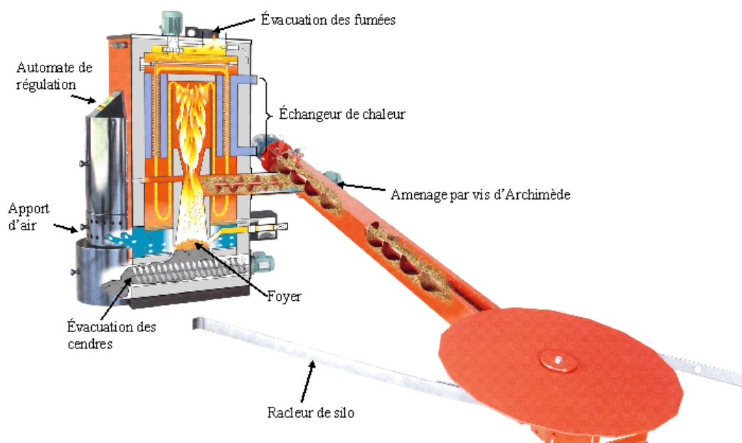
Figure 42 : Schéma de fonctionnement d'une chaudière automatique à plaquettes (source : HARGASSNER)
