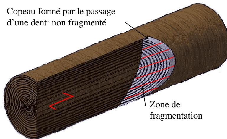
Figure 78 : Copeau non fragmenté retiré par une dent de slabber (à couteaux hachoirs) [HOUZIAUX ;63]
