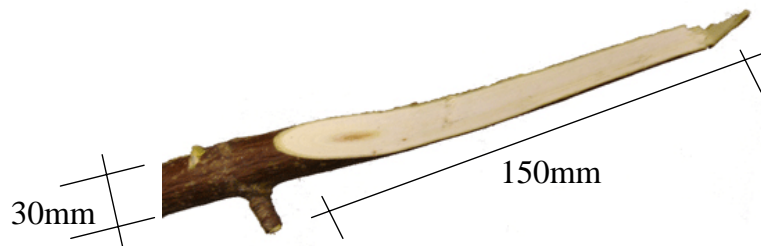
Figure 120 : Etat de surface d'une branche de 30mm de diamètre de coupe amenée à 3km/h et coupée à 400 tr/min.
