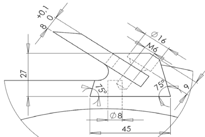
Figure 90 : Vue de dessin de l'assemblage {corps d'outil+insert 55^\circ +couteau}, forme du roule copeau
