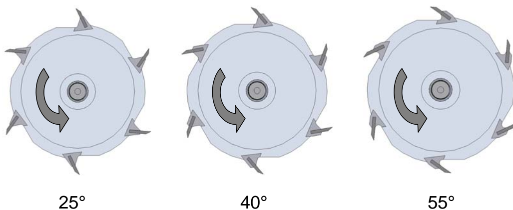
Figure 89 : Vue de dessus de l'outil : différentes configuration d'angles de coupe
