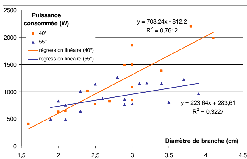
Figure 133 : Puissance consommée en fonction du diamètre de coupe pour deux angles de coupe
