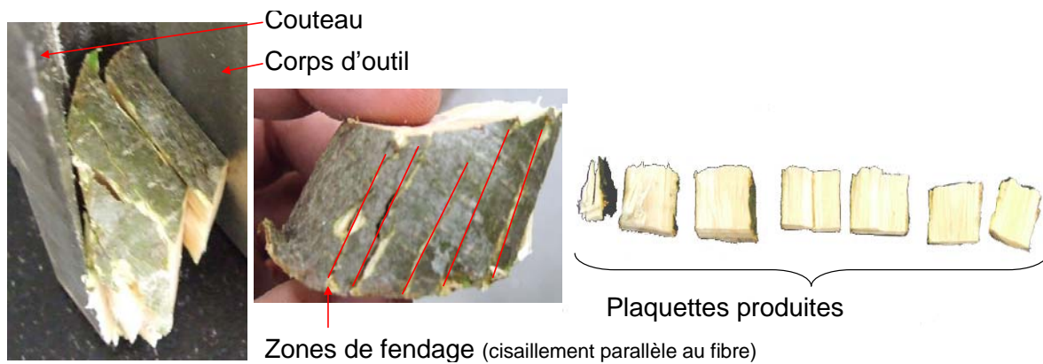
Figure 129 : photos représentant la formation de plaquettes par fendage, effectué à 400tr/min, angle de coupe de 55°, avance 1.5km/h
