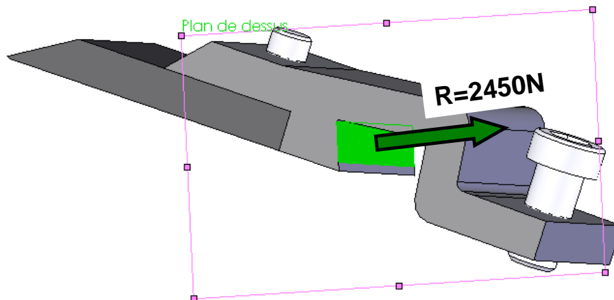
Figure 148 : Représentation de la force résultante à appliquer sur le corps d'outil
