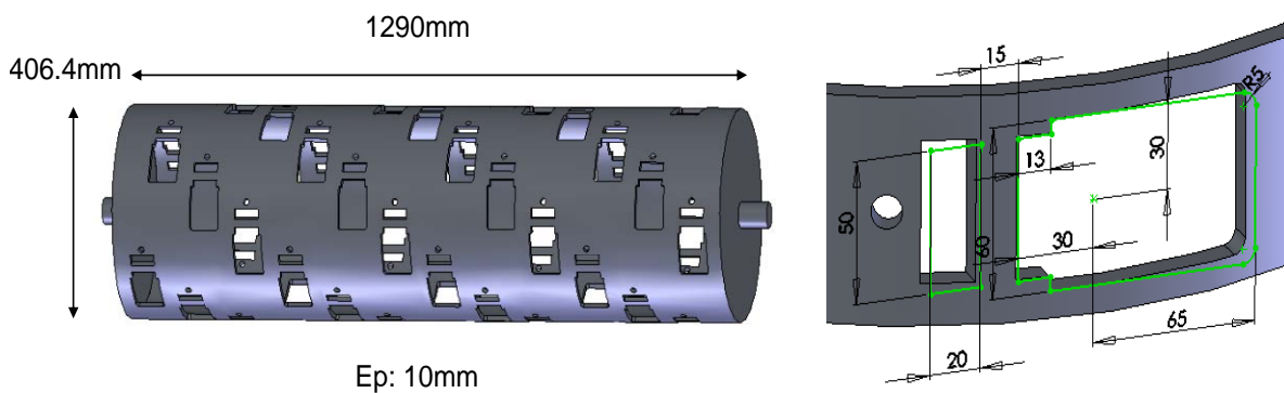
Figure 142 : à gauche, présentation des dimensions générales du corps d'outil et à droite, vue de détail d'une fenêtre
