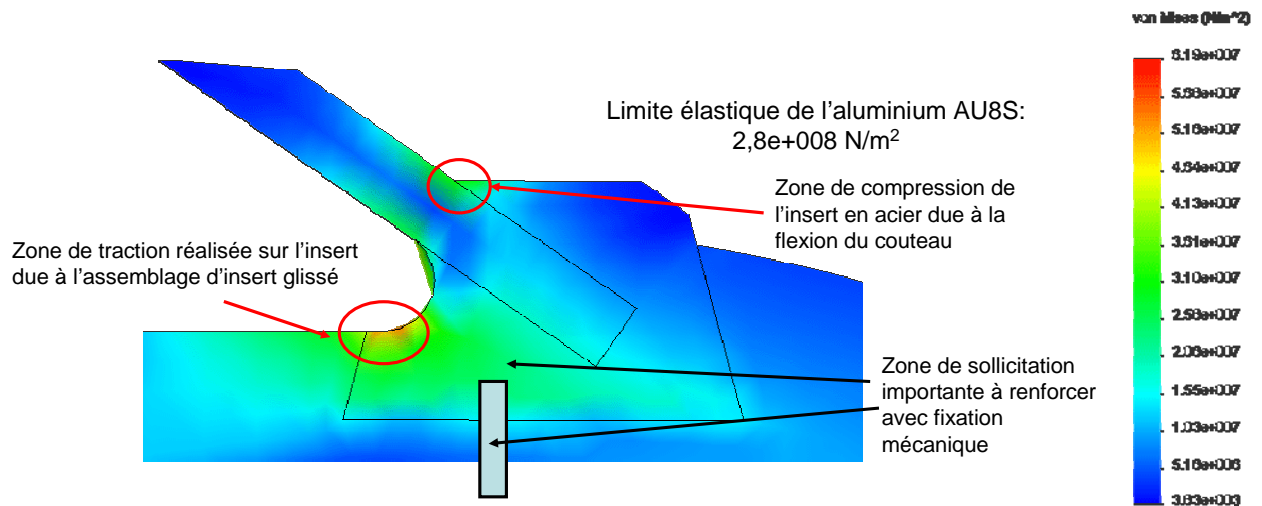
Figure 96 : Grossissement de la zone d'accroche de l'outil.
