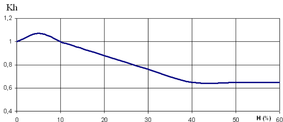
Figure 62 : Influence de l'humidité du bois sur l'effort de coupe tangentiel (Hêtre, E_m=0,2\text{mm} ) [KIVIMAA ; 40]
