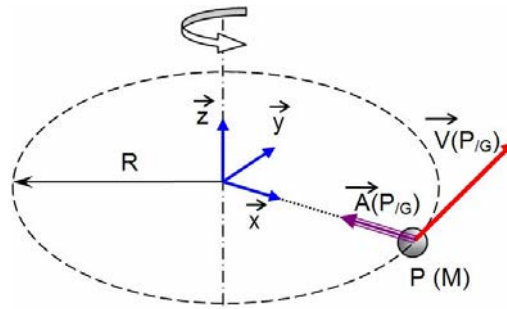
Figure 93 : Représentation schématique de l'action de la force centrifuge
