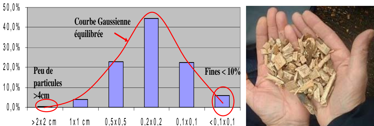
Figure 43 : A gauche, exemple d'une granulométrie correcte de petites plaquettes et à droite, photographie de plaquettes de chauffages correctement calibrées pour le chauffage
