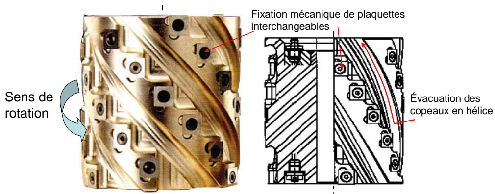
Figure 68 : Outil de rabotage hélicoïdal à plaquettes (GUILLEN Outils Techniques)
