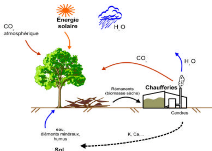
Figure 17 : Cycle simplifié du carbone (source : biomasse normandie)
