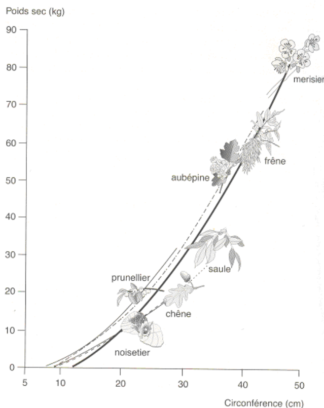
Figure 27 : Courbes de régression donnant la masse sèche du brin en fonction de sa circonférence de base [19]
