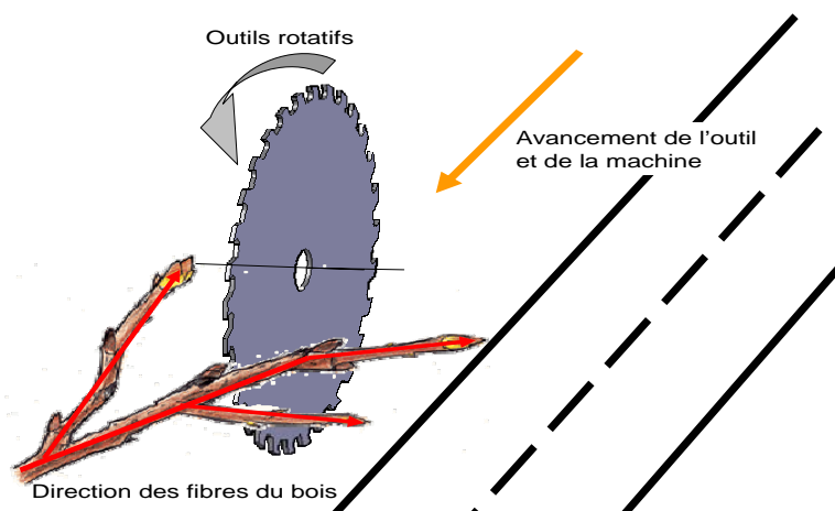
Figure 33 : Schématisation des conditions de coupe par lamier
