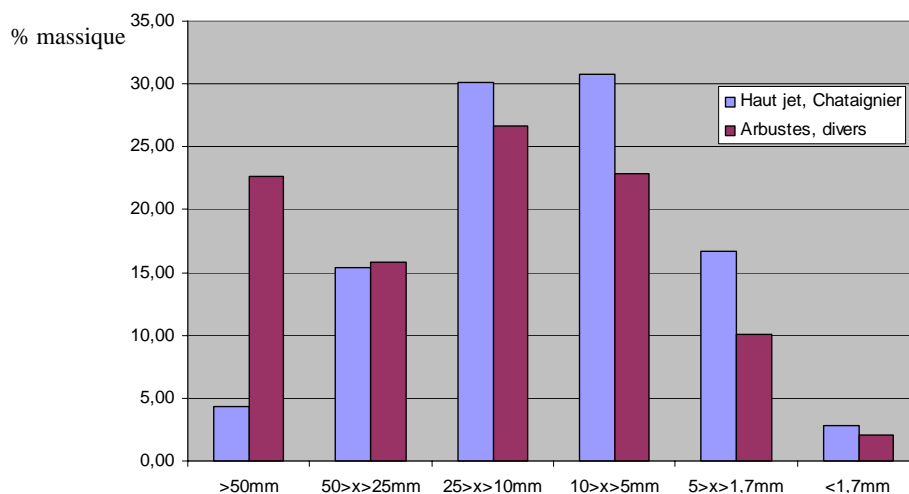
Figure 155 : Comparaison granulométrique entre de coupe d'arbres de haut jet et la coupe d'arbustes.
