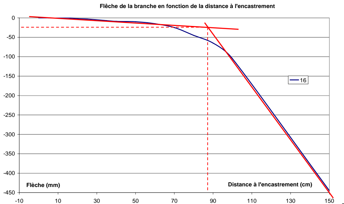
Figure 36 : Forme générale de chaque courbe et obtention du point de flexion
