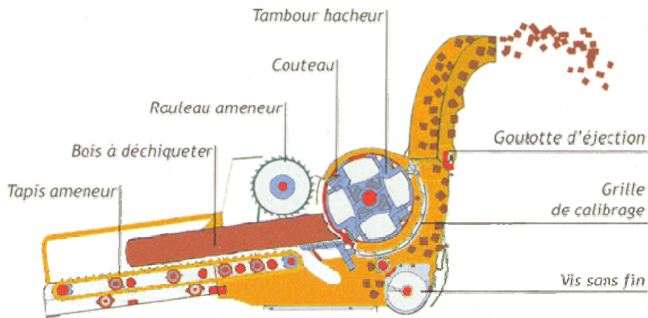
Figure 71 : Principe de fonctionnement d'un broyeur à tambour (NOREMAT)
