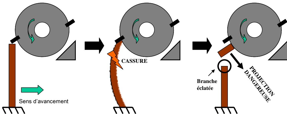
Figure 99 : Phénomènes de cassures liés à l'usinage en avalant
