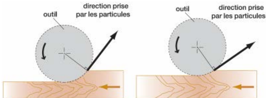
Figure 104 : Variation de la direction de projection en fonction de la prise de passe (diamètre d'outil constant)
