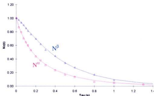
figure 2.41 Evolution des aimantations obtenues avec les séquences d'impulsion de la figure 2.40a, sur le résidu S20 de l'ubiquitine à 9.4T et 300K.
