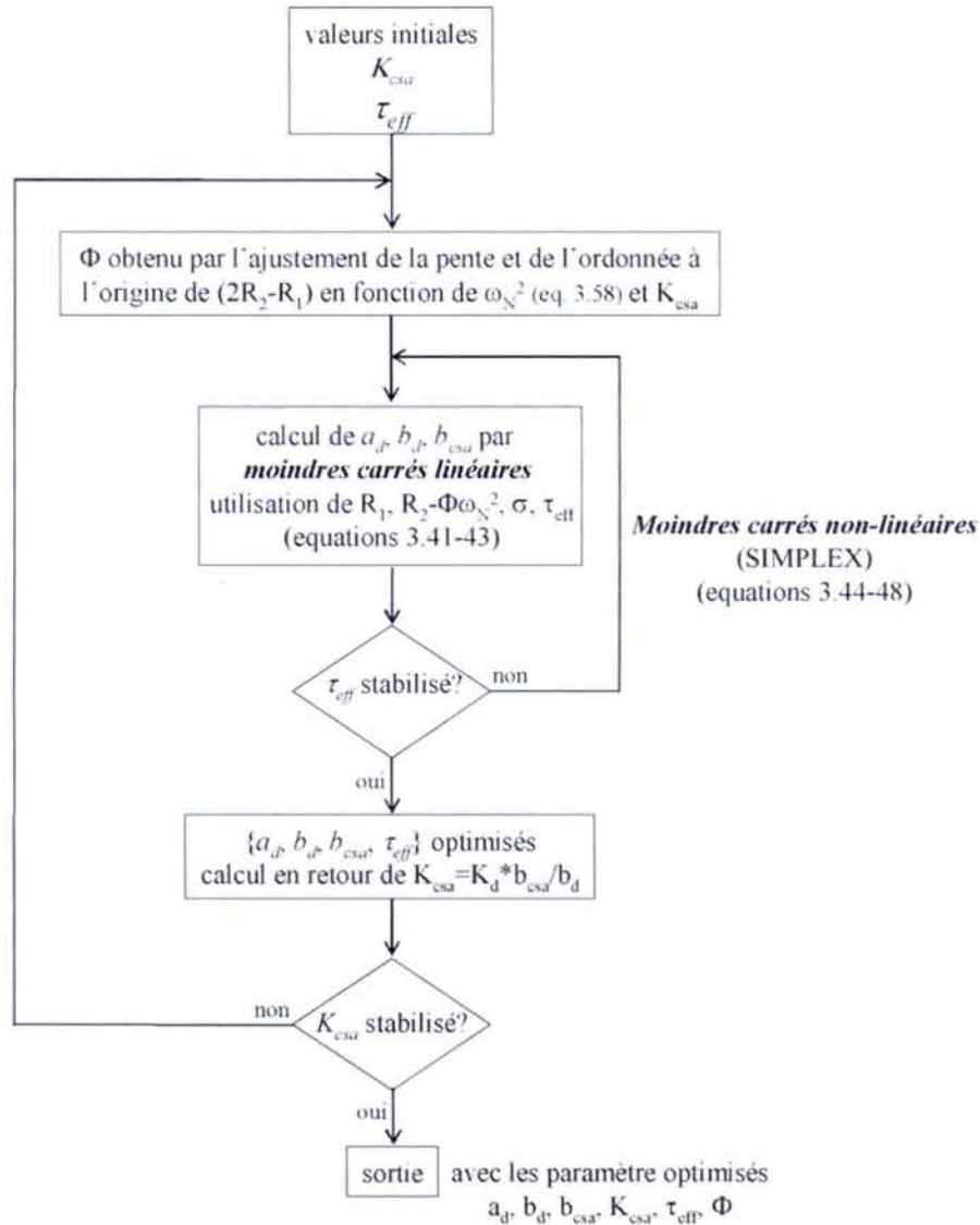
figure 3.7 Diagramme décrivant tout le processus d'ajustement. K_d est supposé constant durant toute la procédure ( r_{NH}=1.02\text{\AA} ).
