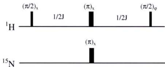
figure 2.14 Séquence BIRD ( Bilinear Rotation Decoupling ).
