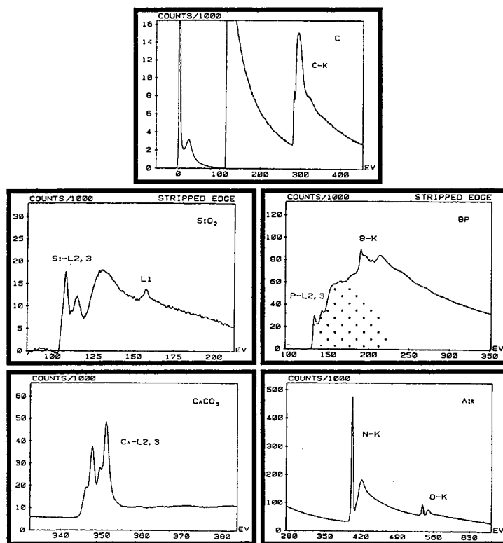
Figure 20 : Pics de pertes d'énergie caractéristiques des différents éléments recherchés (d'après EELS Atlas, 1983).
