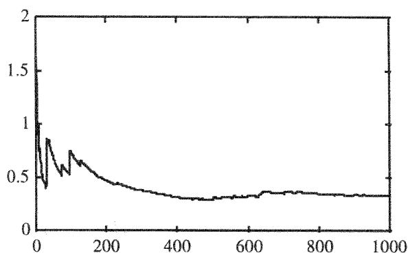
Fig. IV.14. Evolution du critère quadratique obtenue avec l'algorithme RPE.
