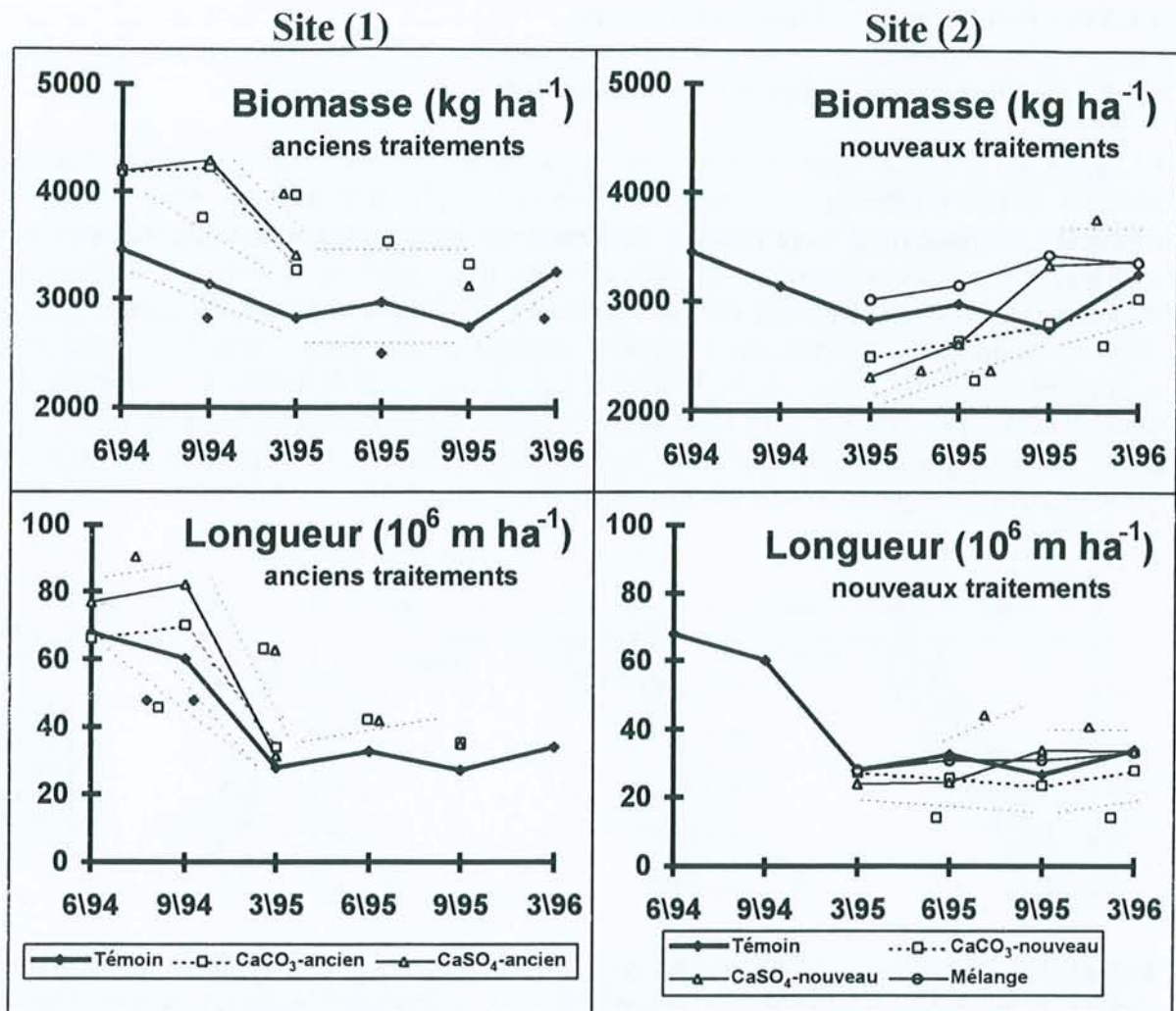
Figure 4.4 Evolution (de juin 1994 à mars 1996) de la biomasse ( \text{kg ha}^{-1} ) et de la longueur totale ( 10^6 \text{ m ha}^{-1} ) des racines fines pour les sites (1) et (2) de la Croix-Scaille (t-test utilisé pour valider les différences entre périodes au seuil de p < 0.05 , soit sur l'ensemble de 0-45 cm, soit horizon par horizon ; les différences sont indiquées par des lignes pointillées finement plus le symbole du traitement. Pour le témoin ces résultats ne sont pas répétés sur les courbes de droite).
