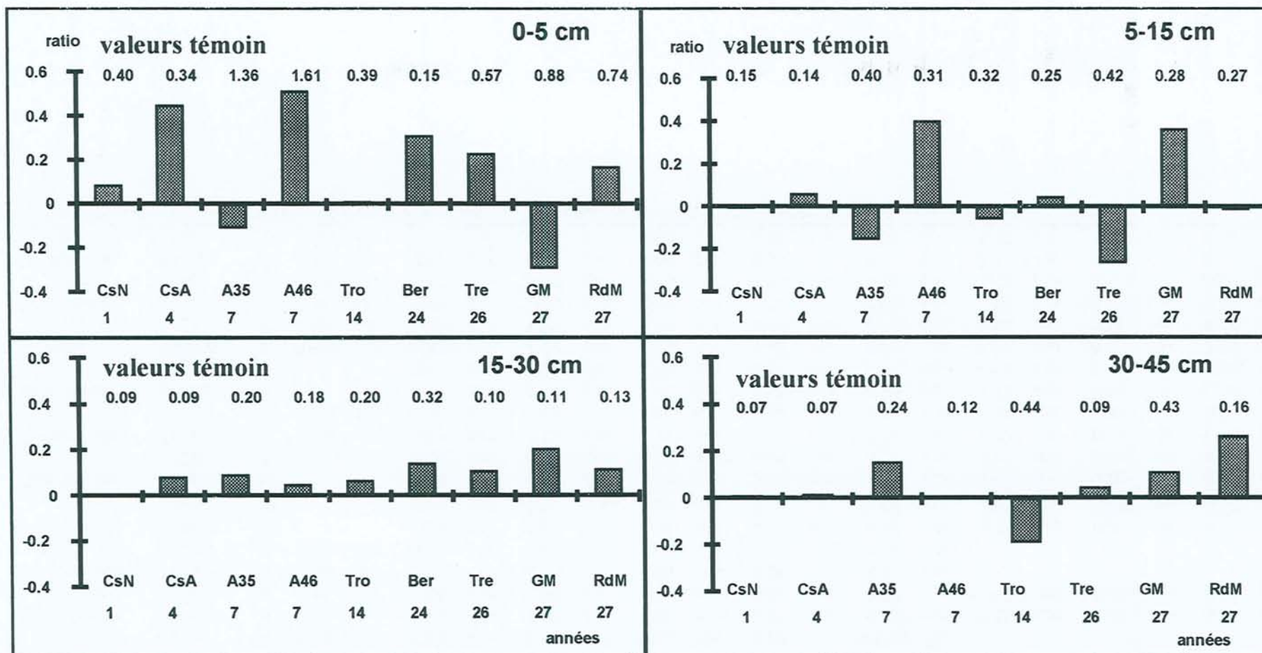
Figure 4.21 Effet de l'amendement (différences absolues: \Rightarrow Ca - Témoins) sur le rapport d'éléments minéraux Ca/Al (mole/mole) des racines fines à quatre niveaux en fonction du temps écoulé depuis l'application (sites indiqués par leurs abrégés).
