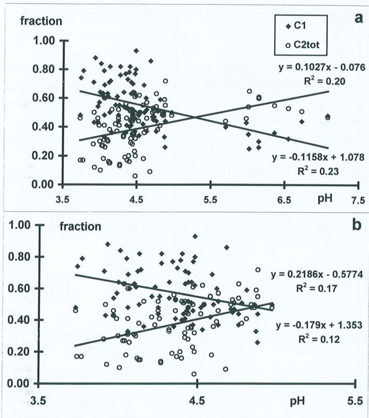
Figure 4.24 Illustration des relations entre les morphotypes ectomycorhiziens C1 et C2, et le pH : a) le site de Fontainebleau inclu et b) site de Fontainebleau exclu.
