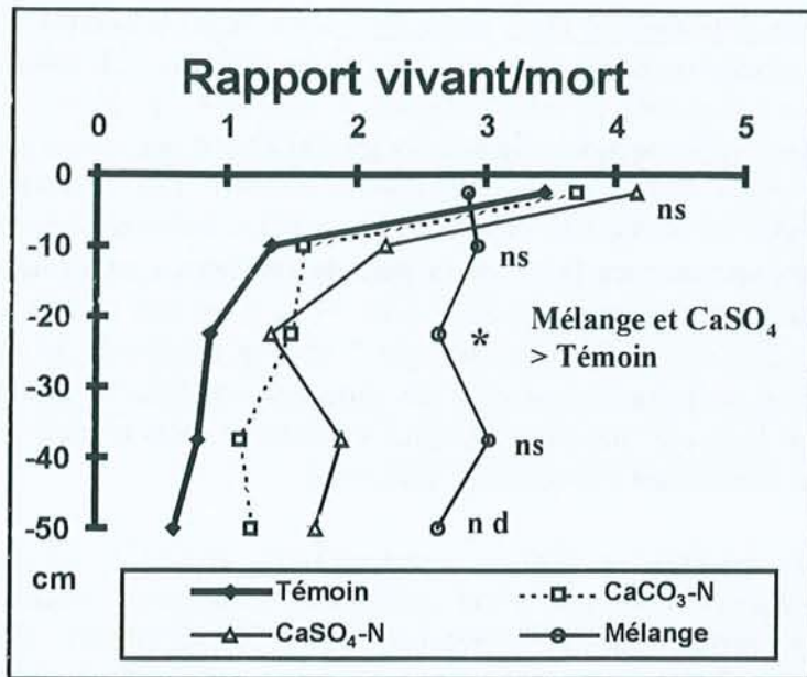
Figure 4.9 Rapport vivant/mort des racines fines dans le profil (basé sur la longueur pour le site (2) de la Croix-Scaille (stat. par horizon ; ns = non significatif et nd = non déterminé).
