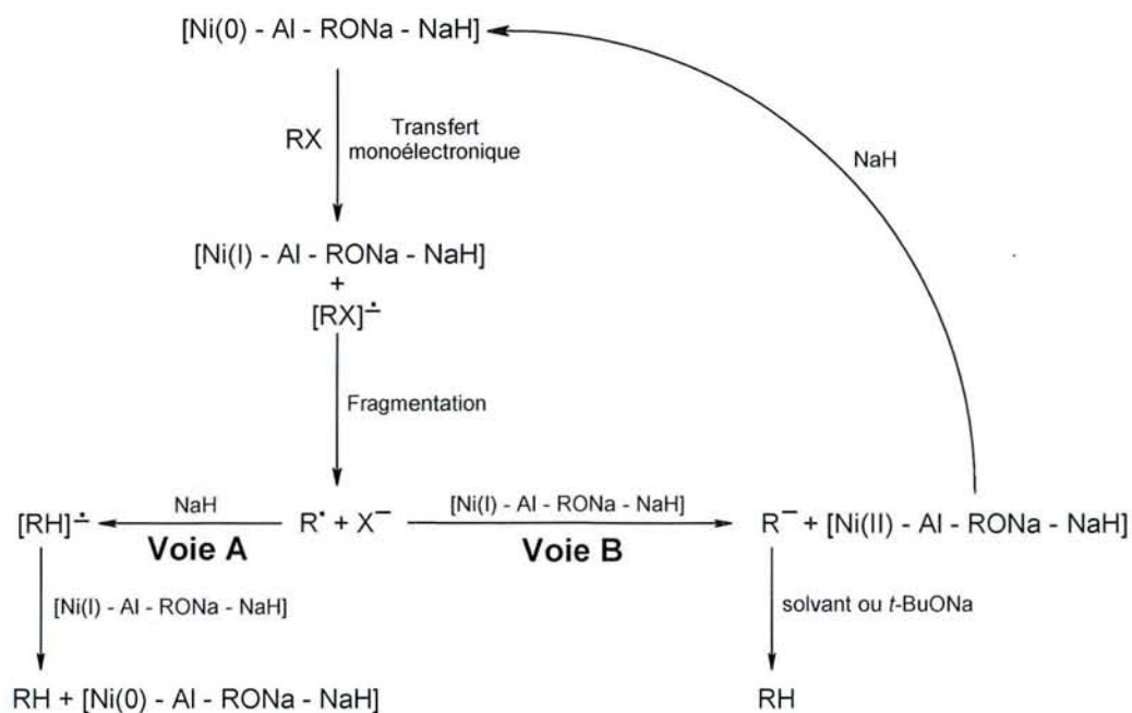
Figure 100 : Réduction par transfert monoélectronique
