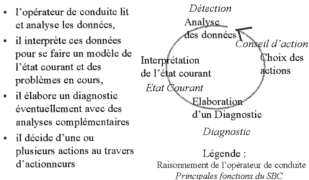
FIG. 3.5 – Le raisonnement de conduite et les quatre fonctions du SBC
