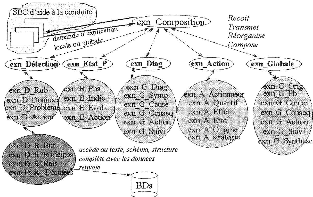
FIG. 6.11 – Architecture multi-agents de la fonction d'explication
