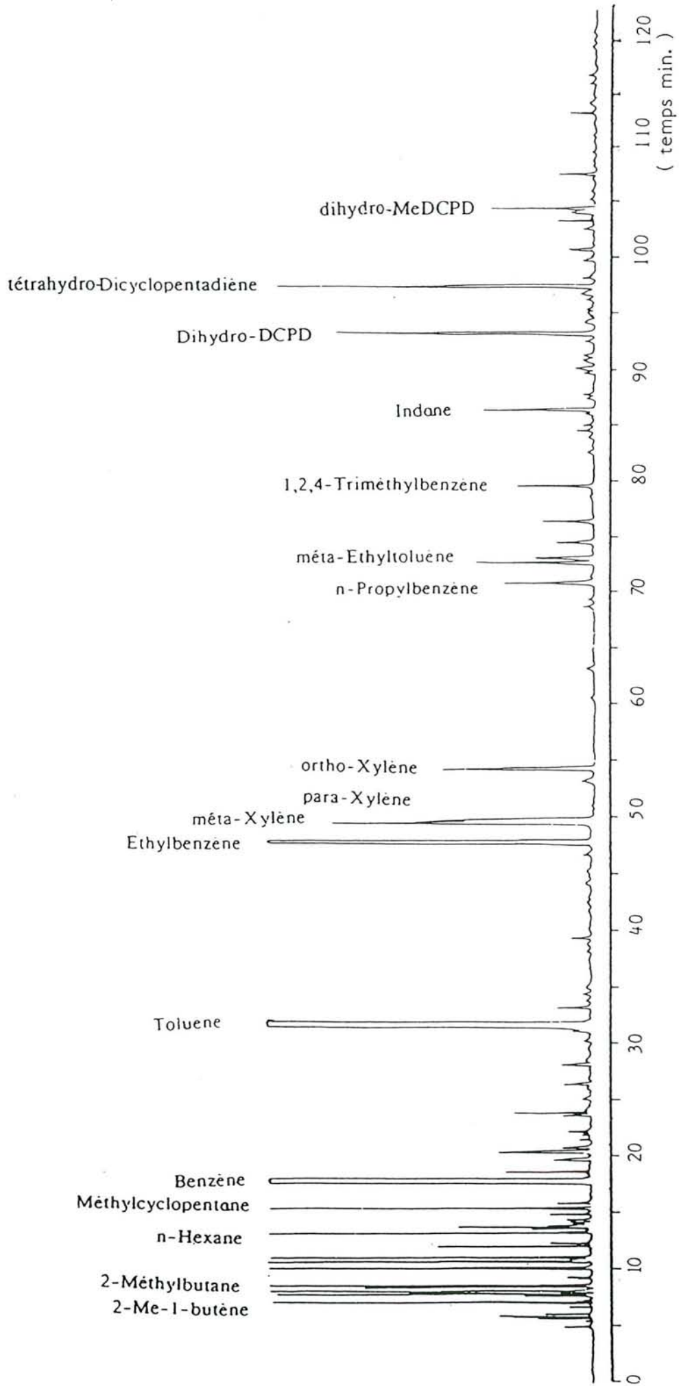
Figure 3.12: Chromatogramme de l'essence E8. Seuls les pics principaux sont mentionnés. (colonne HP 1)
