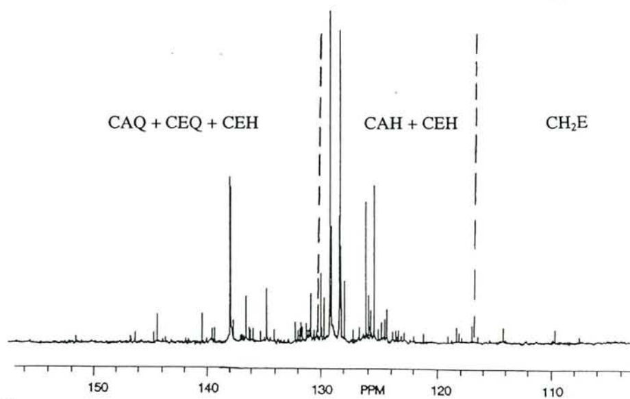
Figure 3.18: Spectre ^{13}\text{C} quantitatif à 100 MHz et spectres édités de l'essence FCC de coeur brute (partie insaturée).
