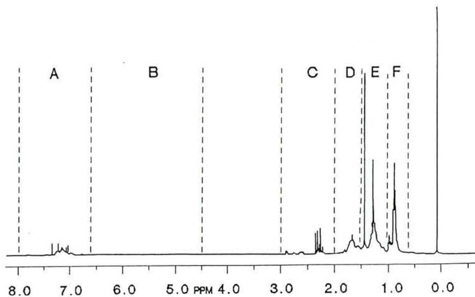
Figure 3. 8: Spectre ^1\text{H} à 400 Mhz de l'essence de charbon polonais (référence: hexaméthylsiloxanne, \delta = 0,55 ppm par rapport au TMS)
