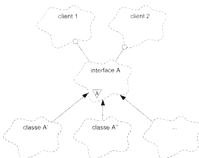
FIG. 2.10 – Classe abstraite
