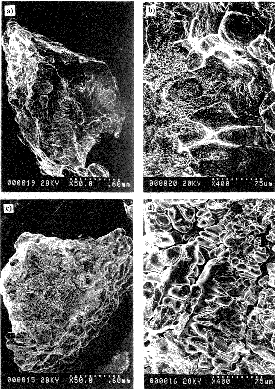
Figure III.27 : Profil fractographique des barreaux après le test de pliage
