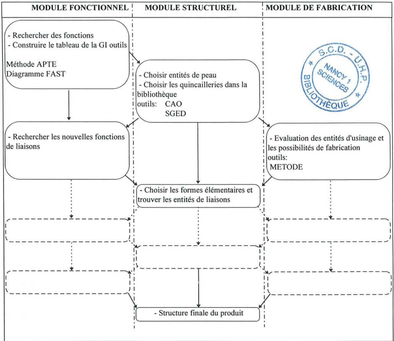
figure 2.27 : Le modèle fonctionnel, structurel et fabrication [GAR 96]
