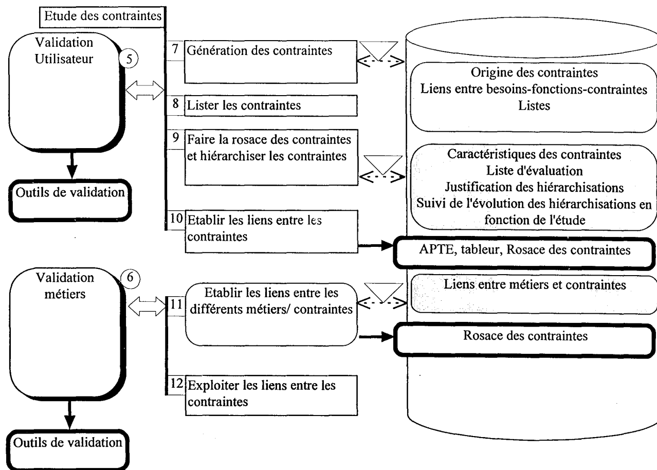
figure 4.12 : la génération de contraintes
