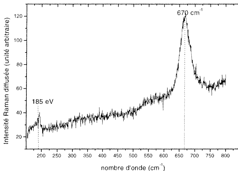
Figure E-22: Spectre de diffusion Raman obtenu pour un dépôt de \text{Fe}_3\text{O}_4 déposé sur MgO (épaisseur 50 Å).
