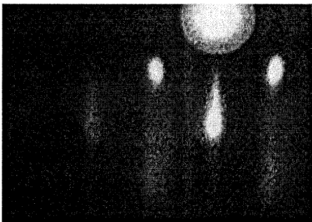
Figure E-14: Evolution des images de diffraction RHEED selon les azimuts [-110] et [010] au cours de l'évaporation de fer sur \text{MgO}(001) : (a) et (b) \text{MgO} bombardé et recuit à 800\text{ °C} , (c) épaisseur de fer de 10\text{ Å} , (d) et (e) 25\text{ Å} .
