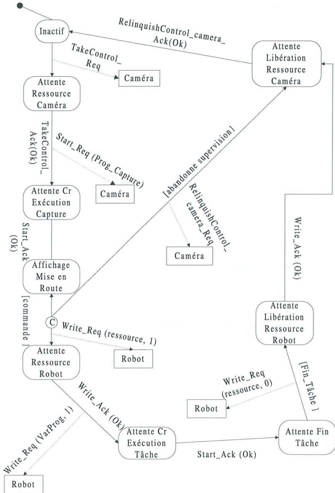
Figure 12. Diagramme d'états représentant le suivi d'événements précédent.
