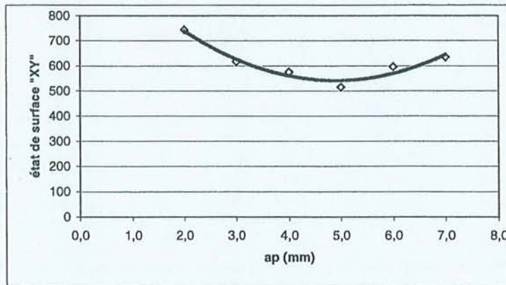
Figure 69 : Evolution de l'état de surface en fonction de l'engagement radial « ap ».
