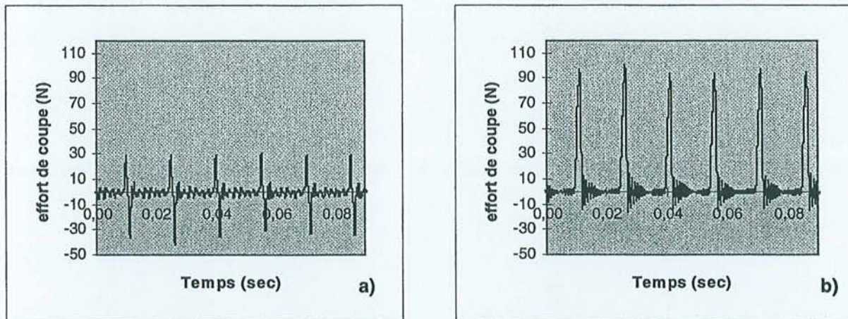
Figure 34 : a) Efforts de coupe dans la direction de la profondeur de passe x ; b) efforts de coupe dans la direction de l'avance y .
