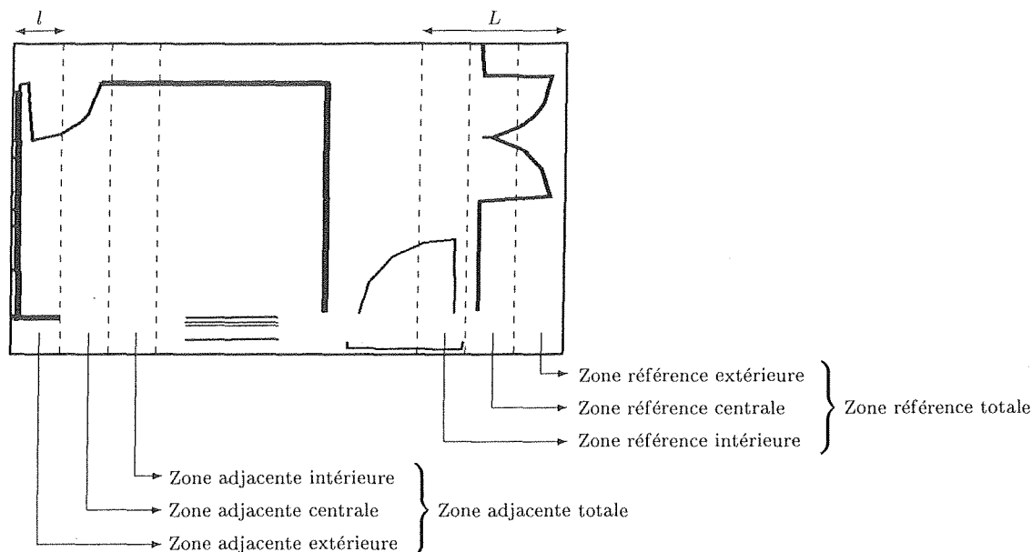
FIG. 4.2 – Détail des différentes sous-zones d'une tuile. Les sous-zones présentées sont les sous-zones verticales. Le même découpage est effectué pour les sous-zones horizontales.
